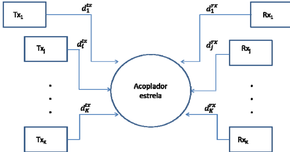
Figura 6 – Arquitetura de rede OCDMA
