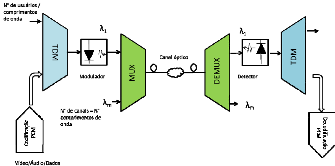
Figura 2 – Esquema básico de um sistema de comunicação utilizando tecnologia WDM.
