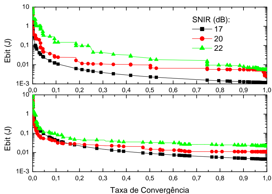
Figura 16 – Soma da energia por bit por OCPs em função da taxa de convergência utilizando
