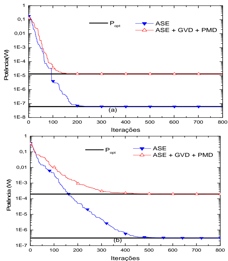
Figura 15 – Somatória da evolução da potência PSO para a) 4 OCPs; b) 8 OCPs, considerando 1 span como referência com R = 10 Gbps. Duas situações avaliadas: i) efeito da ASE; ii) ASE, GVD e PMD.
