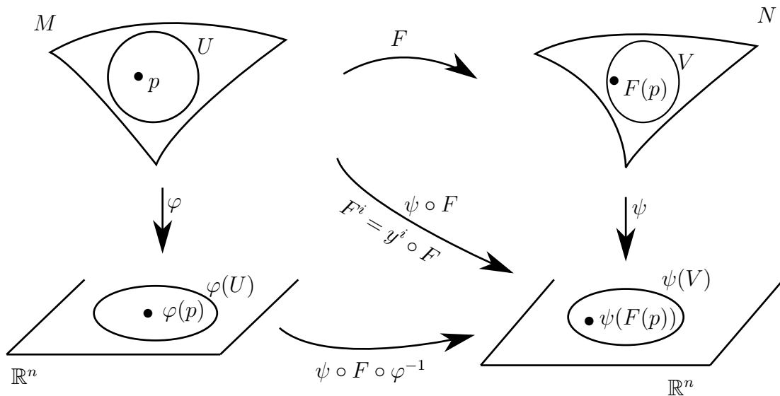
Figura 1.7: Teorema da Função Inversa
