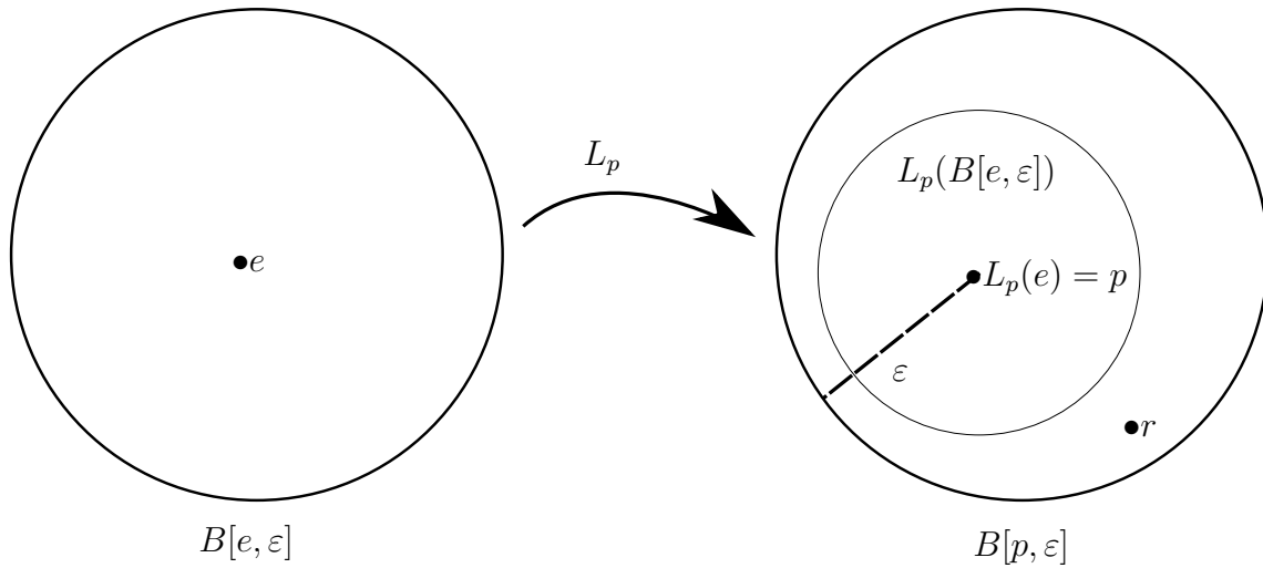
Figura 2.2: Prova do Lema 2.39(b)
