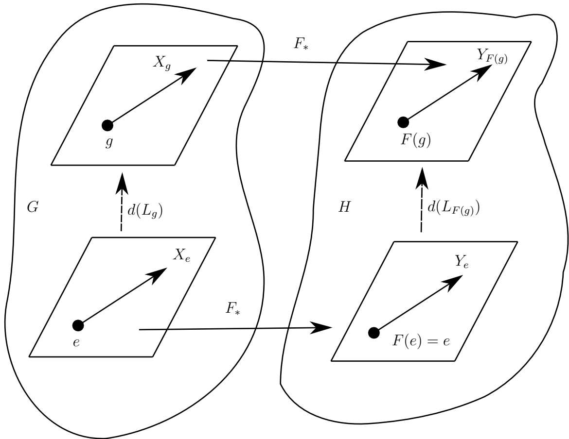
Figura 1.11: Homomorfismo induzido entre álgebras de Lie
