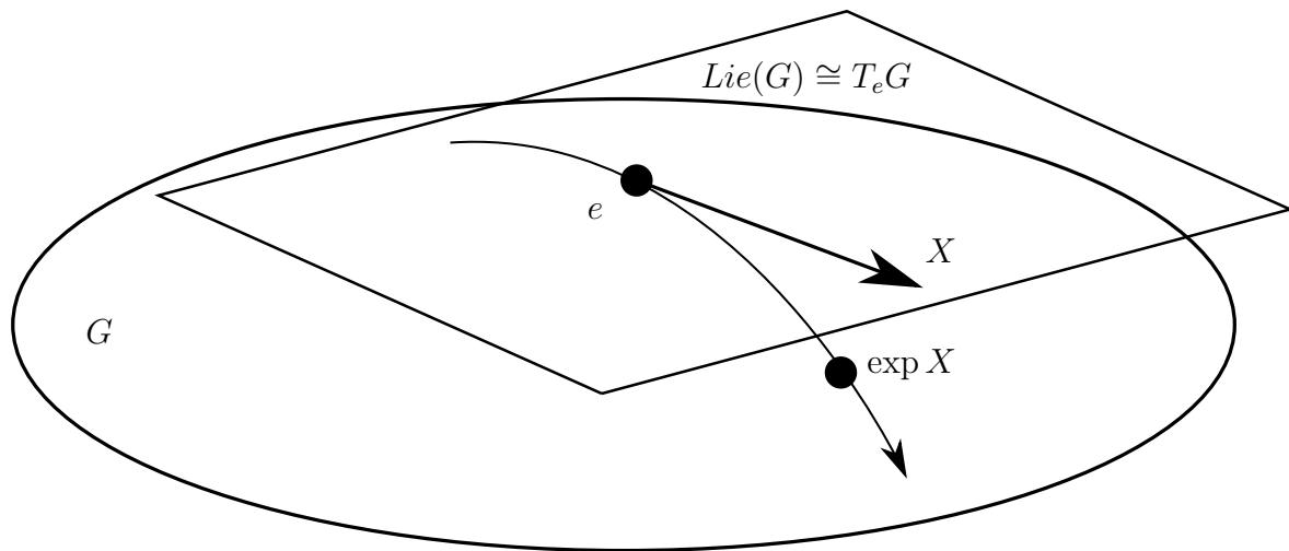
Figura 1.13: A aplicação exponencial
