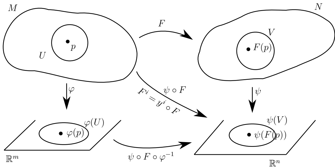
Figura 1.6: A matriz Jacobiana
