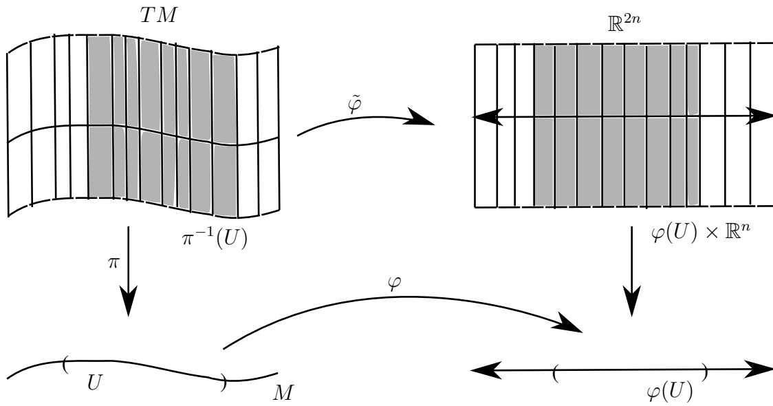
Figura 1.8: Fibrado tangente para as coordenadas
