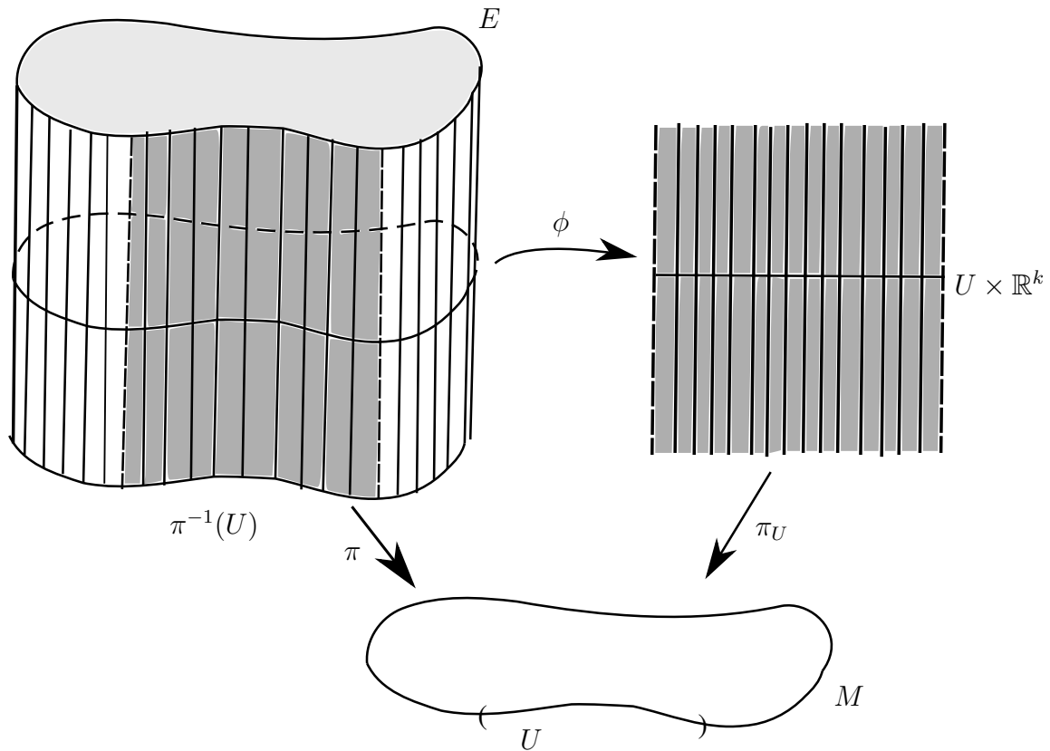
Figura 1.12: Uma trivialização local de um fibrado vetorial
