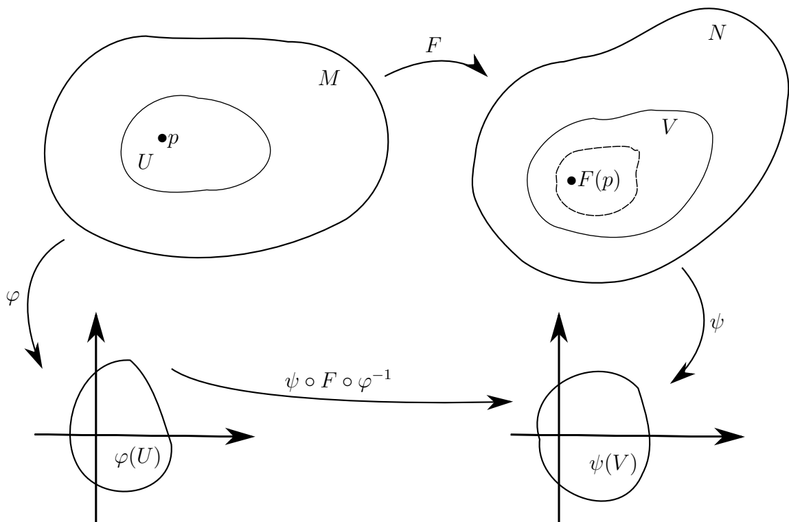
Figura 1.3: Definição de Aplicação Suave
