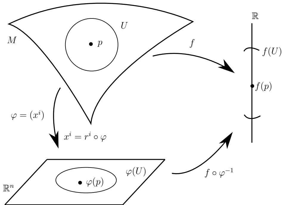
Figura 1.5: A derivada parcial
