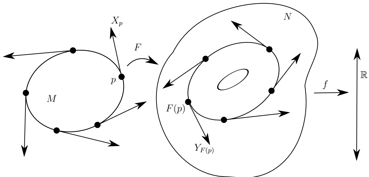
Figura 1.9: Campos vetoriais F -relacionados
