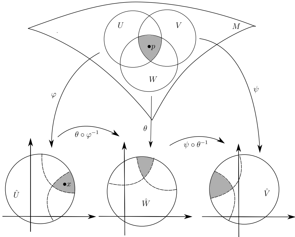
Figura 1.2: Prova da Prop. 1.5(a)
