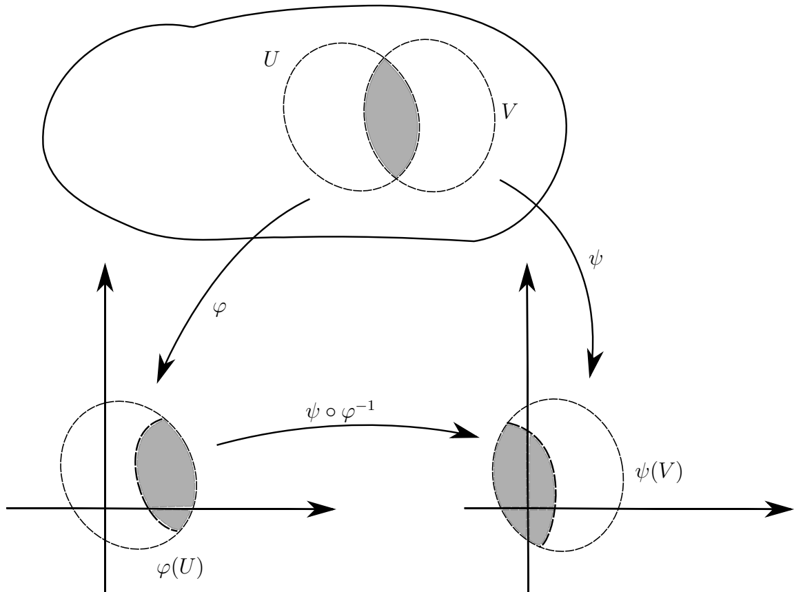
Figura 1.1: Aplicação de transição
