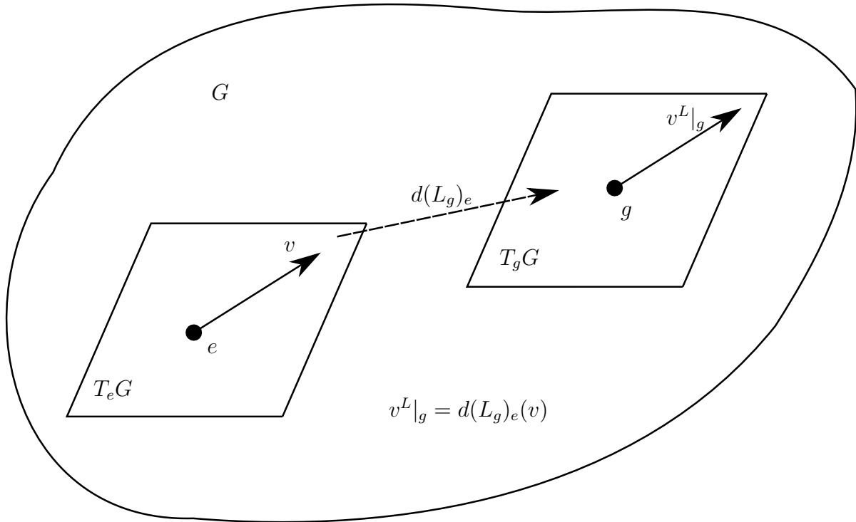
Figura 1.10: Definindo um campo vetorial invariante à esquerda
