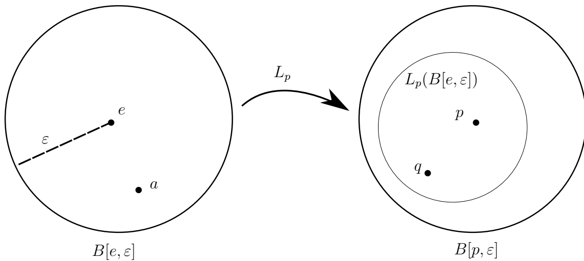
Figura 2.1: Prova do Lema 2.39(a)
