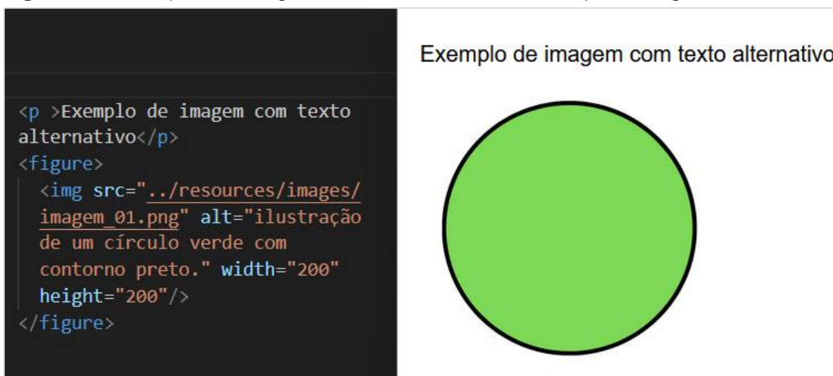
Figura 1 – Exemplo de código HTML com texto alternativo para imagem
