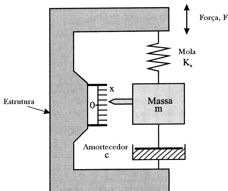
Figura 5.1: Sistema massa-mola. Fonte: Modificado de Lawrence (1998)
