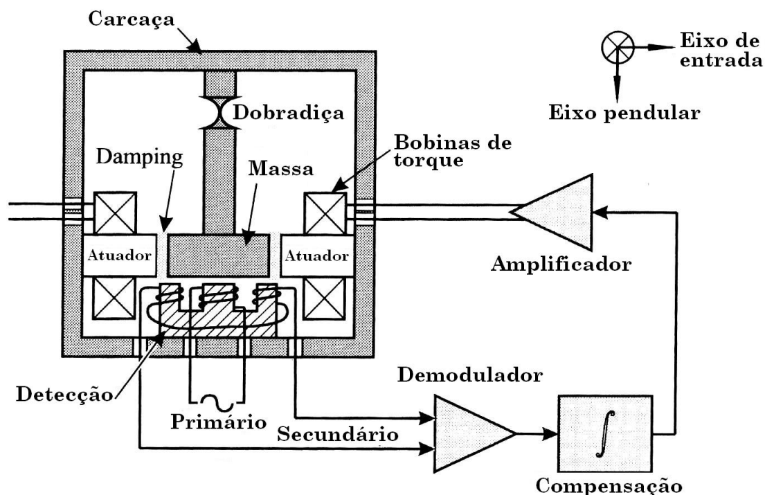
Figura 5.2: Acelerômetro pendular servo controlado.
