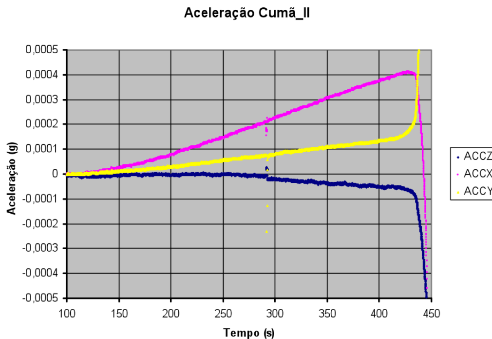
Figura 3.7: Acelerações observadas pela plataforma Microg1 durante o período de microgravidade nos eixos X, Y e Z.
