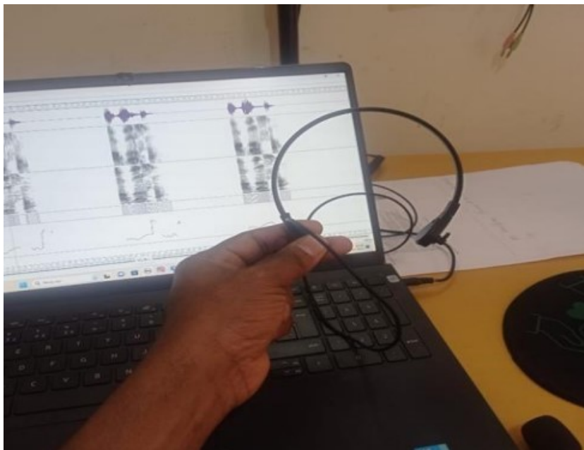
Figura 25 – Captura de Voz por Laringofone
