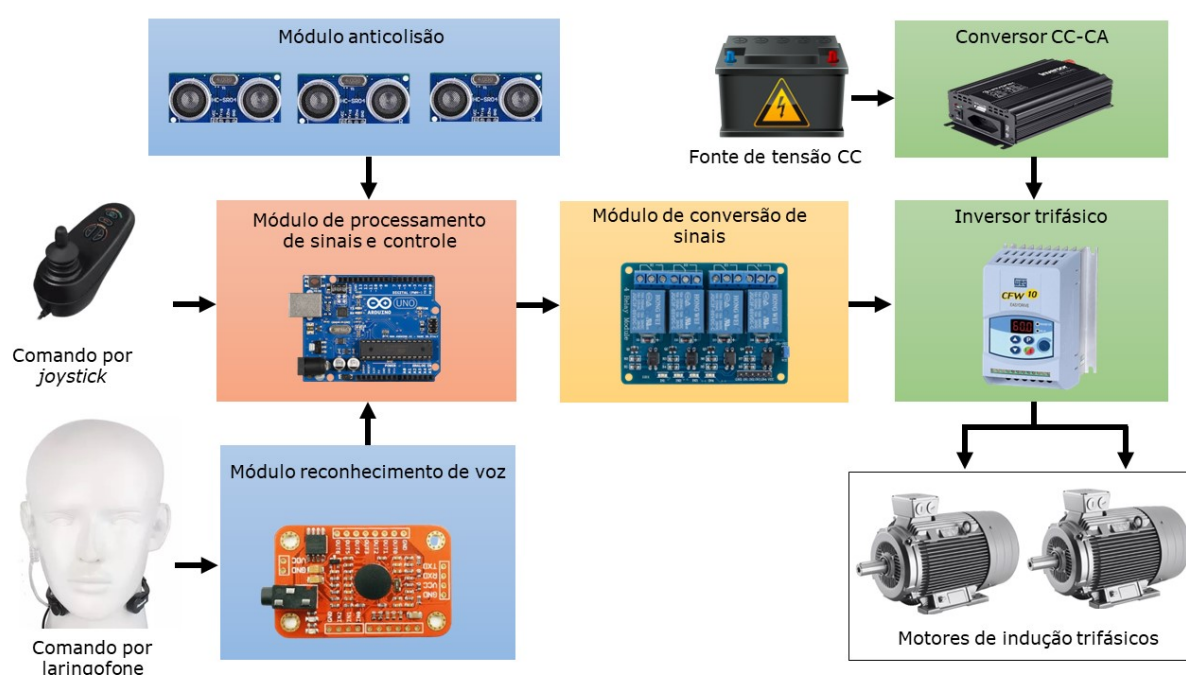
Figura 10 – Sistema Proposto em Blocos funcionais.
