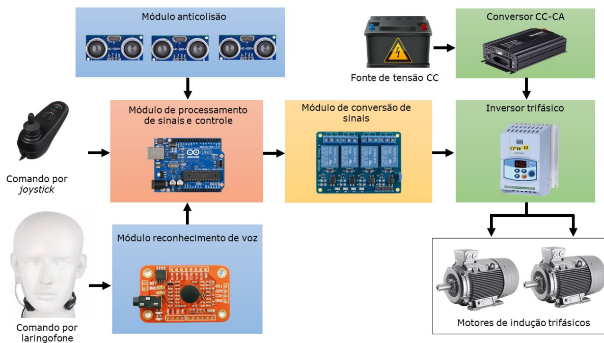
Figura 3 – Blocos Funcionais do Protótipo.
