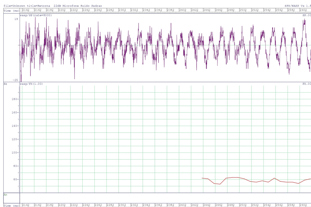
Figura 32 – Gráfico do Sinal de Comando de Voz Retorna à 22 dB – Microfone com ruído
