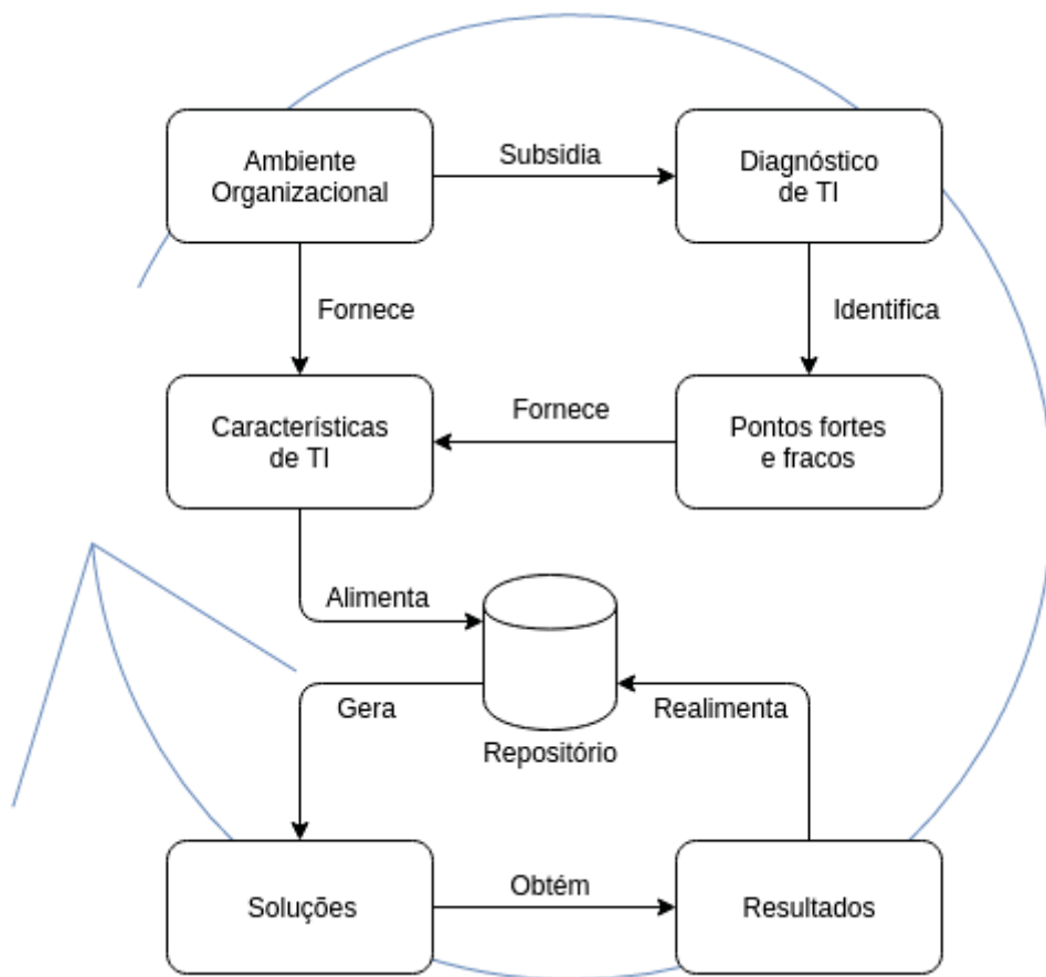
Figura 2 – Visão geral do framework . Adaptado de [2].
