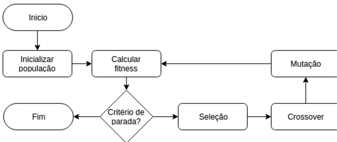
Figura 11 – Fluxograma do funcionamento do GA. Adaptado de [5].
