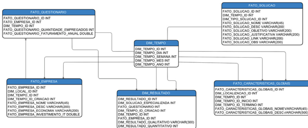
Figura 16 – Relacionamento entre os fatos do repositório.
