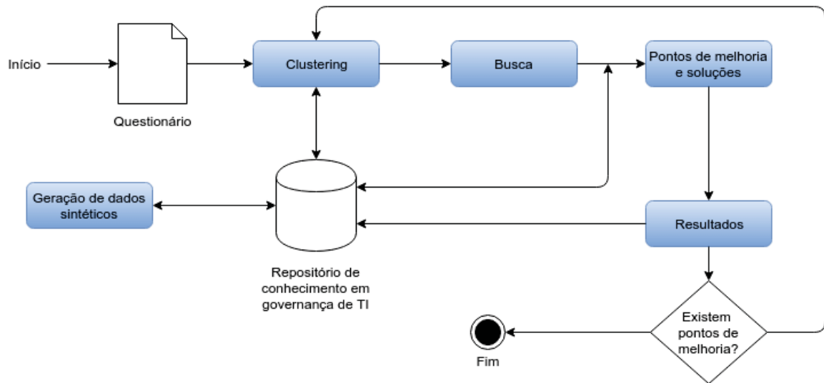
Figura 14 – Arquitetura do sistema de recomendação de pontos de melhoria em governança de TI.
