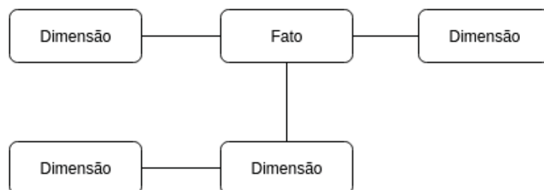
Figura 7 – Modelo floco de neve. Adaptado de [3].
