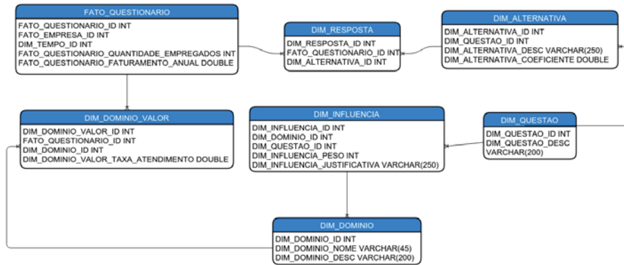
Figura 17 – Mapeamento do questionário pelo repositório.
