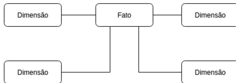
Figura 6 – Modelo estrela. Adaptado de [3].
