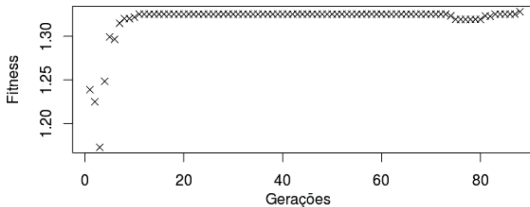
Figura 19 – Exemplo de evolução do fitness por geração.
