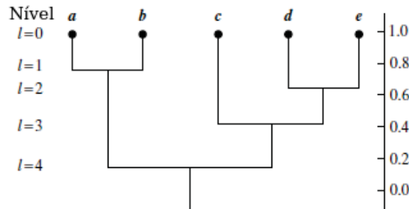
Figura 10 – Exemplo de resultado de uma estratégia aglomerativa. Disponível em [3].
