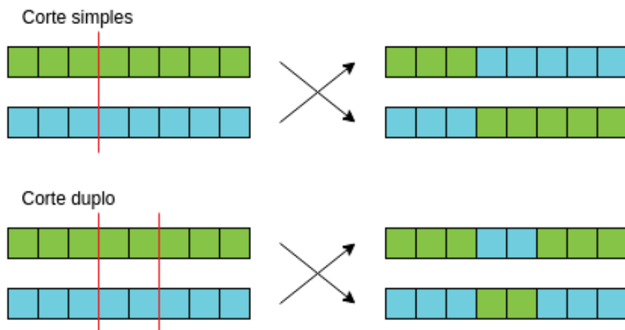
Figura 12 – Esquematização do processo de crossover com corte simples e duplo.
