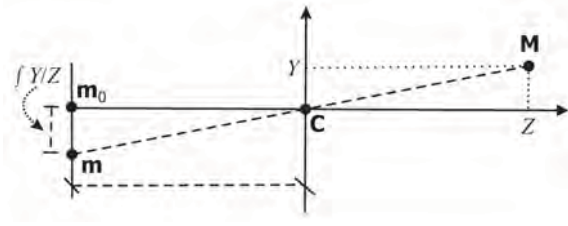
Figura 2.3: Determinação da ordenada do ponto \mathbf{m} em função das coordenadas do ponto \mathbf{M}
