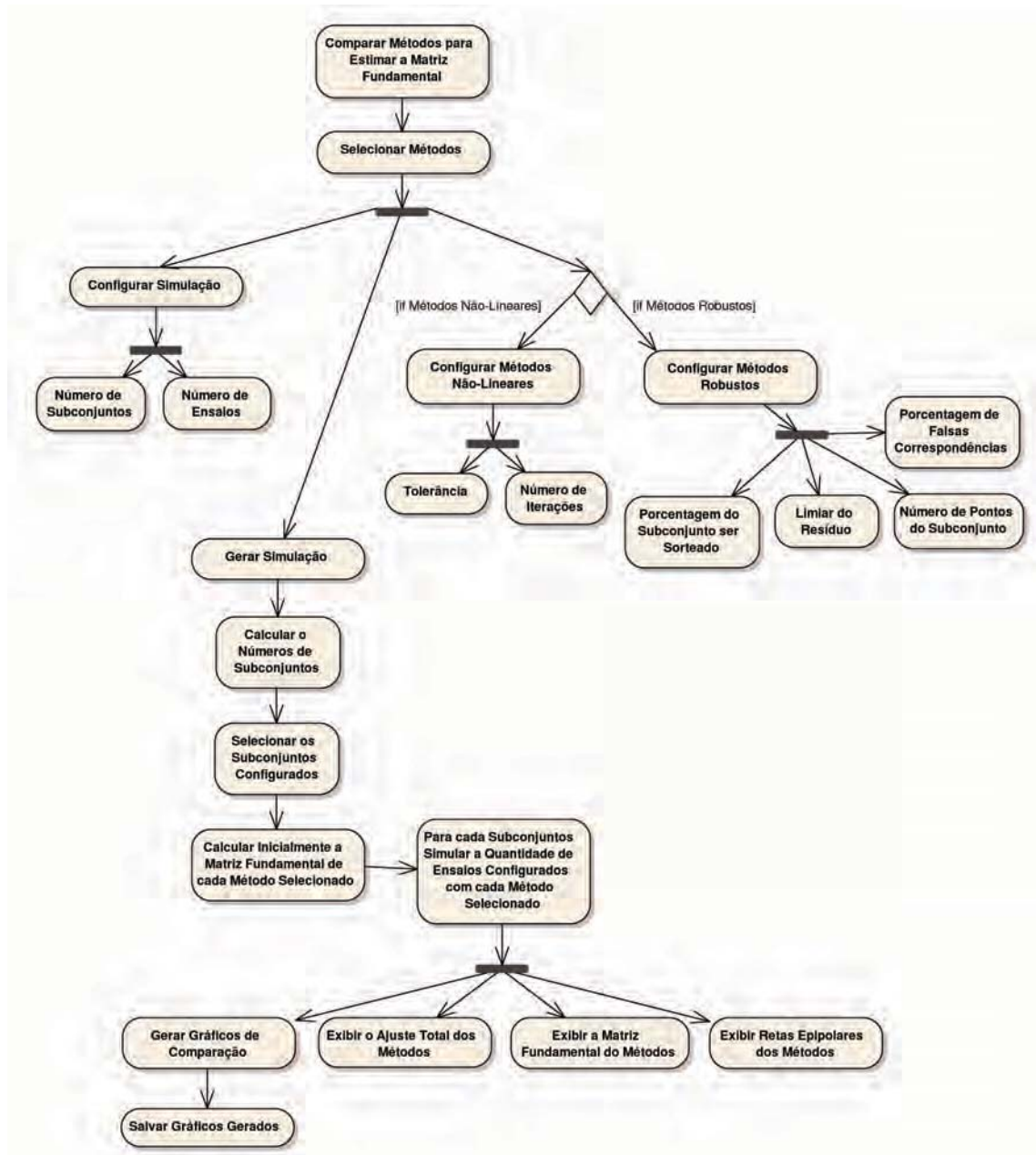
Figura 3.12: Atividades da Simulação de Comparações entre Métodos para Estimar a Matriz Fundamental
