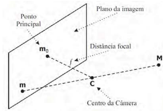
Figura 2.1: Esboço de uma câmera pinhole .
