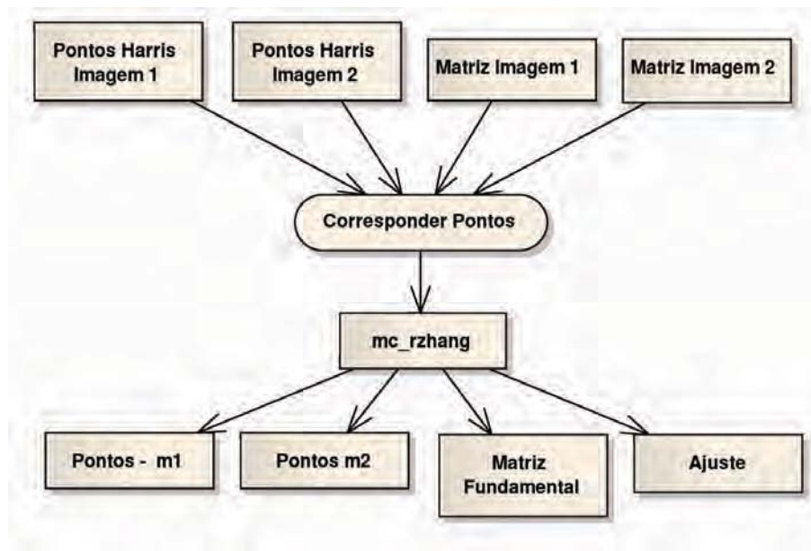
Figura 3.10: Atividades da Correspondência de Pontos pelo Ambiente Computacional
