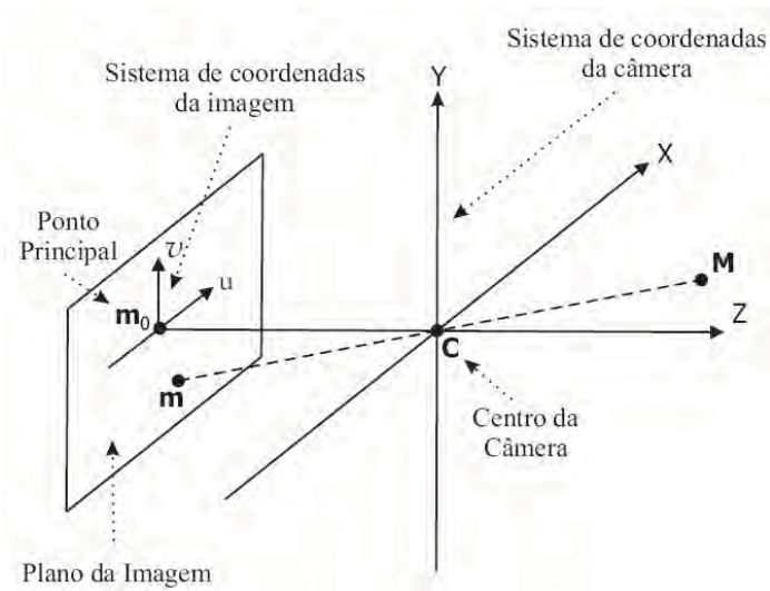
Figura 2.1: Esboço de uma câmera pinhole .
