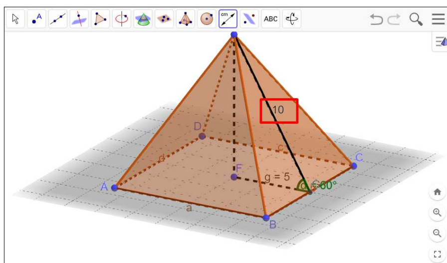
Figura 48 – Cálculo do apótema da pirâmide no GeoGebra
