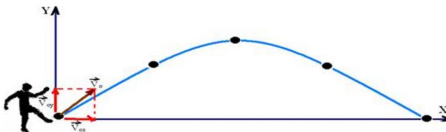
Imagem 13 – fonte: http://fisicaevestibular.com.br/novo/wp-content/uploads/migracao/lancamento-obliquo/i_37adfe7059a981ab_html_d4dad34f.png
