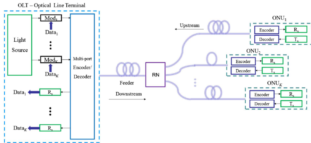
Figura 2.3: Arquitetura de rede 40G-OCDMA-PON.
