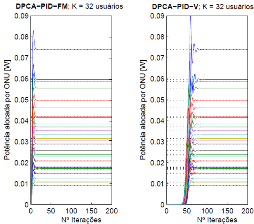
Figura 5.19: 40G-PON-OCDMA com 32 ONUs. Alocação de potência por ONU para DPCA-PID-FM e DPCA-PID-V.
