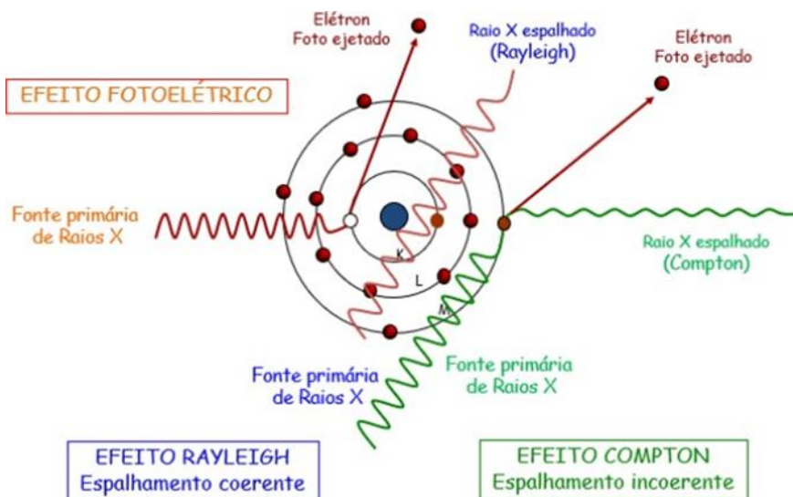
Figura 2 – Representação esquemática dos efeitos Fotoelétricos e os de espalhamento Compton e Rayleigh em um átomo. Em vermelho, indicando o elétron ejetado pelo Efeito Fotoelétrico; em azul, o feixe de Raios X espalhado sem perda de energia na interação; e em verde, o feixe espalhado com ângulo diferente do ângulo de incidência.
