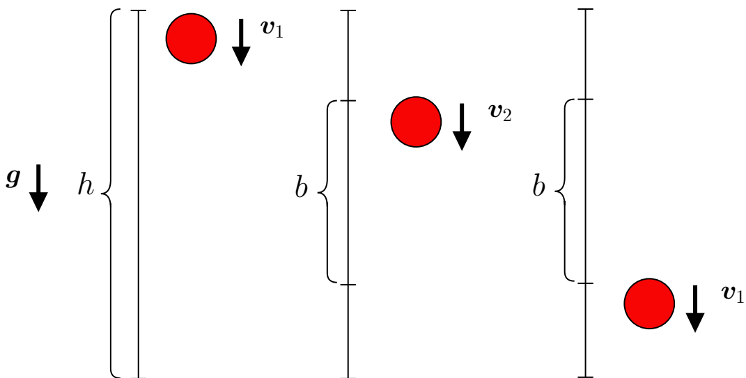
Figura 3.26: Representação de um experimento no qual soltamos uma bolinha de uma certa altura e esta apresenta uma velocidade descontínua em seu percurso no trajeto delimitado por b . Fonte: Autor.
