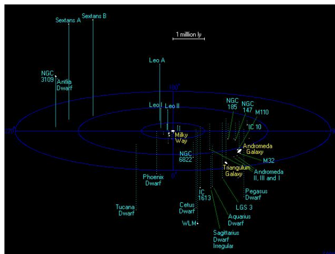
Figura 3.9: Ilustração de 1 milhão de anos-luz de afastamento da Via Láctea. Fonte: Richard Powell.
