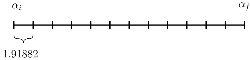
Figura 5.4: Grade ilustrativa dos valores de \alpha com divisão em 12 partes iguais no intervalo de redshift 0 \leq z \leq 10^{10} .
