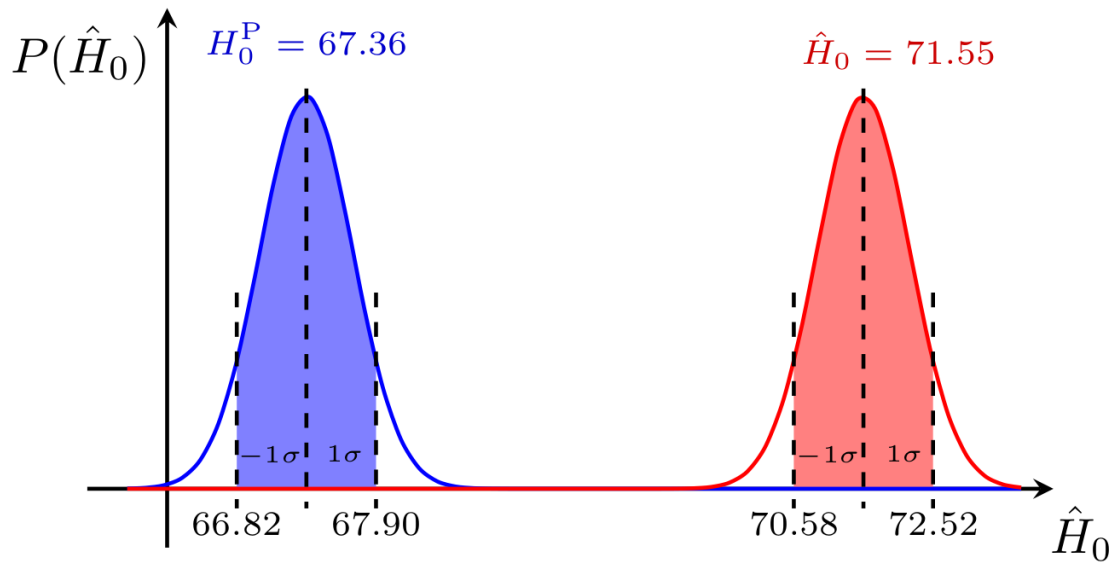
Figura 6.2: Representação ilustrativa da distribuição marginal de \hat{H}_0 e da medida do Planck H_0^P associando 1\sigma as suas respectivas regiões de confiança. Região de confiança de \hat{H}_0 e da medida do Planck H_0^P , ambas associadas a 1\sigma = 68.3\% de confiança.
