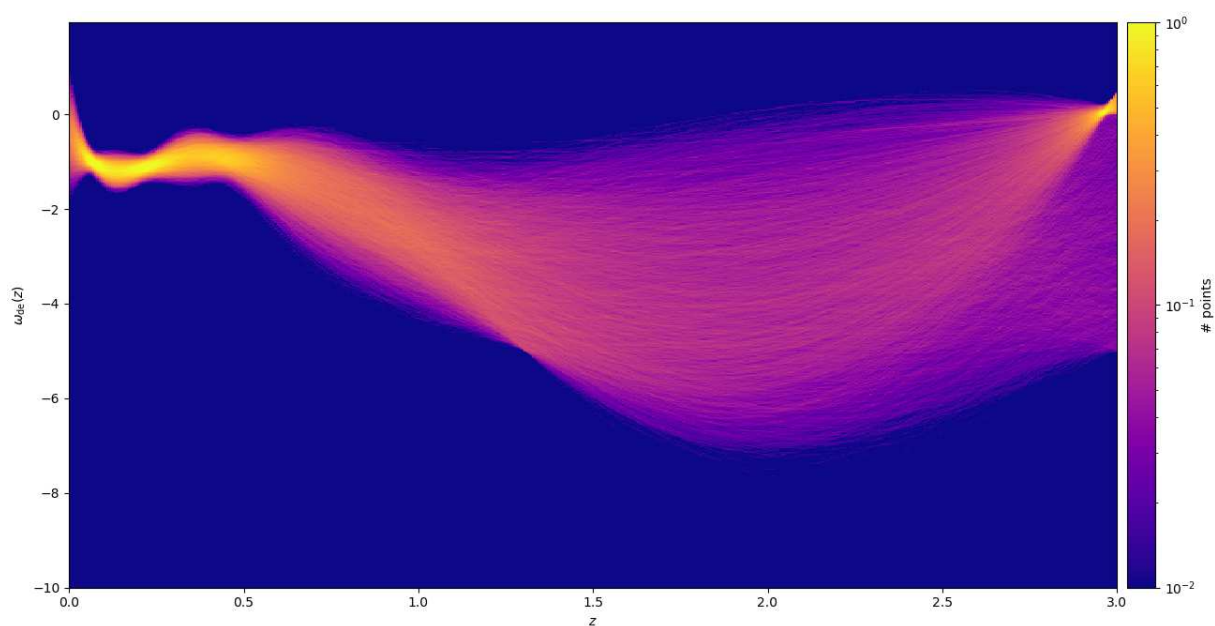
Figura A.1: Gráfico de densidade de probabilidade para o best-fit de 6 nós na interpolação polinomial de w(z) para o intervalo de redshift de 0 \leq z \leq 3.0 .
