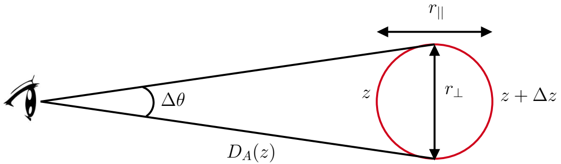
Figura 4.1: Representação trigonométrica para as duas contribuições da escala acústica: a radial r_{\parallel} e a transversal r_{\perp} . Fonte: Autor.
