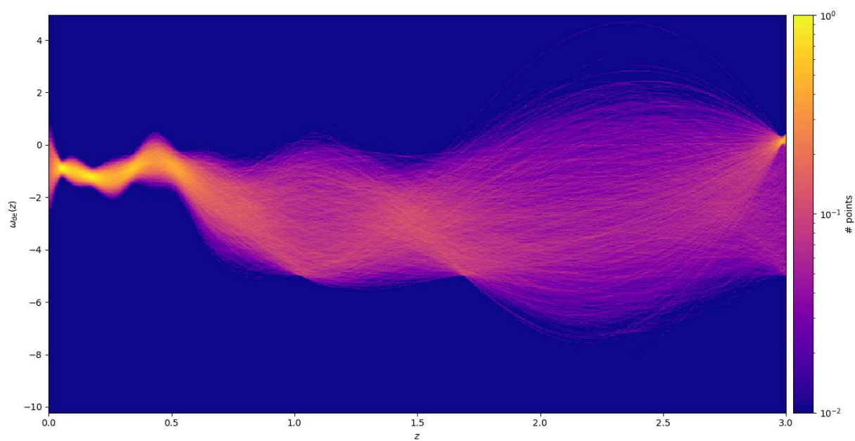
Figura A.3: Gráfico de densidade de probabilidade para o best-fit de 8 nós na interpolação polinomial de w(z) para o intervalo de redshift de 0 \leq z \leq 3.0 .
