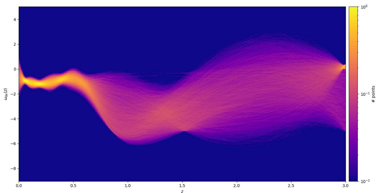
Figura A.2: Gráfico de densidade de probabilidade para o best-fit de 7 nós na interpolação polinomial de w(z) para o intervalo de redshift de 0 \leq z \leq 3.0 .
