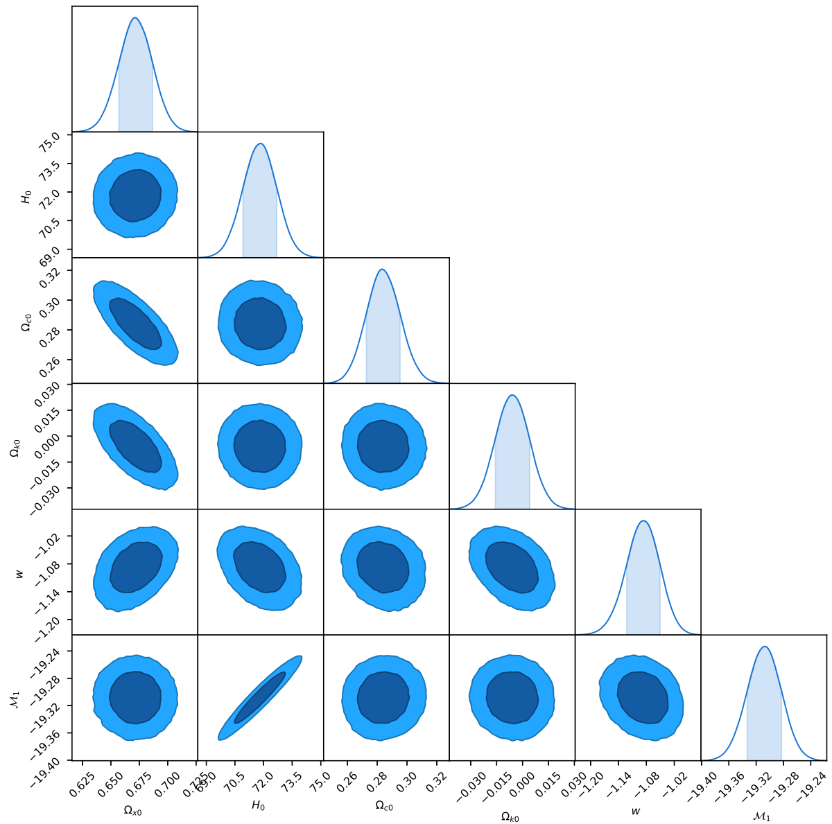
Figura 6.6: Regiões de confiança de 1\sigma = 68.3\% (central/escuro) e 2\sigma = 95.4\% (externa/clara) para os parâmetros cosmológicos H_0 , \Omega_{\text{DE}0} , \Omega_{c0} , \Omega_{\kappa0} , w , e M_1 (Modelo XCDM ( w constante)). A área sombreada na distribuição marginal representa 1\sigma .
