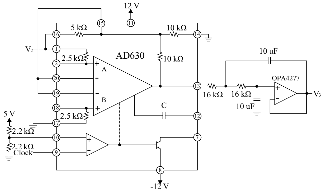
Figura 3.8: Esquemático do circuito de amplificação Lock-in .
