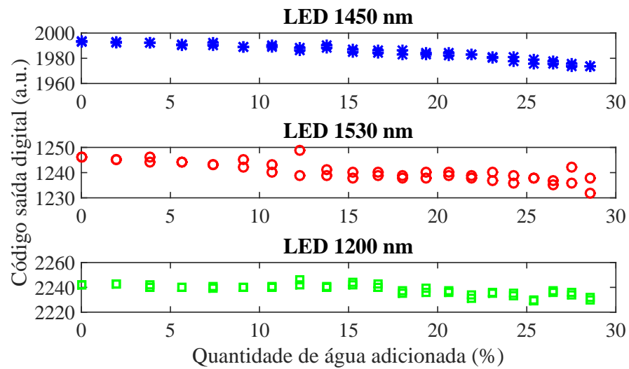
Figura 4.10: Valores de saída do conversor A/D para os LEDs de 1450 nm, 1530nm e 1200 nm.
