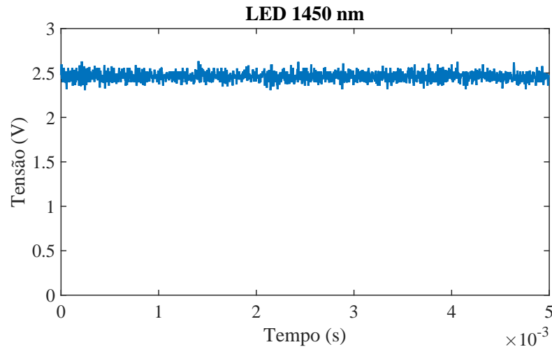
Figura 4.8: Sinal de saída do amplificador Lock-in .
