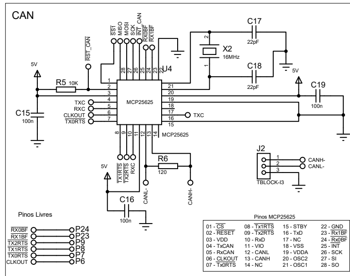
Figura 3.2: Esquemático para utilização do CI MCP25625.
