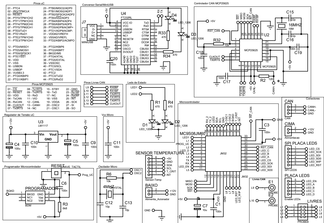
Figura A.2: Diagrama esquemático da placa de controle do driver dos LEDs.
