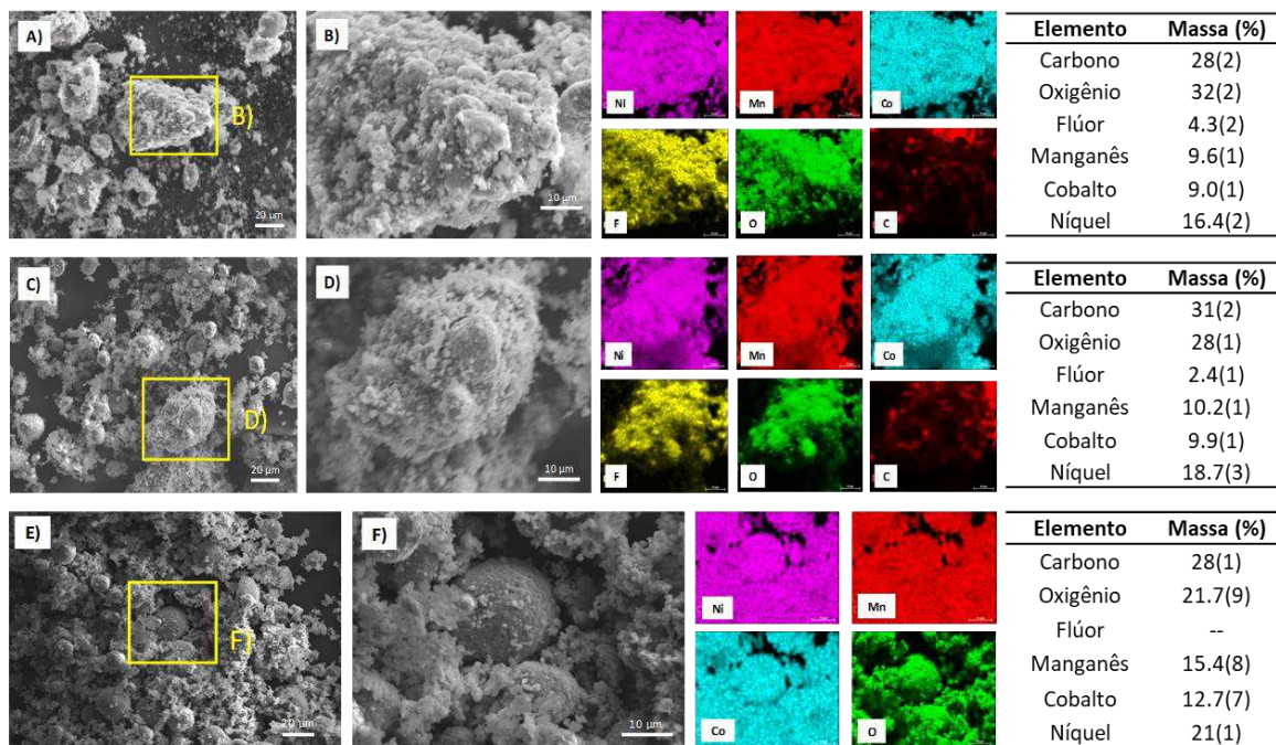
Figura 38 - Análise de MEV e EDX dos materiais do catodo EoL como-recebido (a) e (b), delaminado (c) e (d) e após a reliação (e) e (f)
