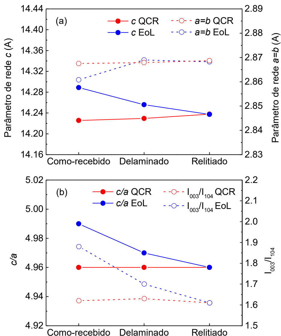
Figura 34 - Parâmetros de rede c e a=b e (a) a razão c/a , e a razão de intensidade I_{003}/I_{104} para os compostos nas condições de recebimento, delaminação e relitiação das amostras QCR e EoL (b)
