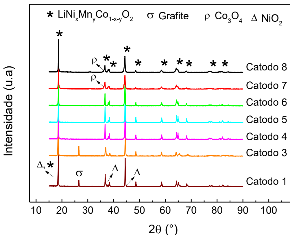
Figura 14 - Difractogramas de raios-X dos pós extraídos dos catodos da Tabela 1
