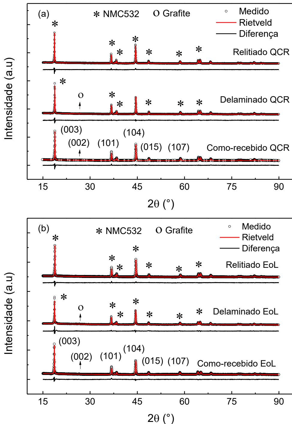
Figura 33 – Difratomogramas de raios-X das amostras QCR (a) e EoL (b) como-recebidas, delaminadas e após a relitiação via estado sólido
