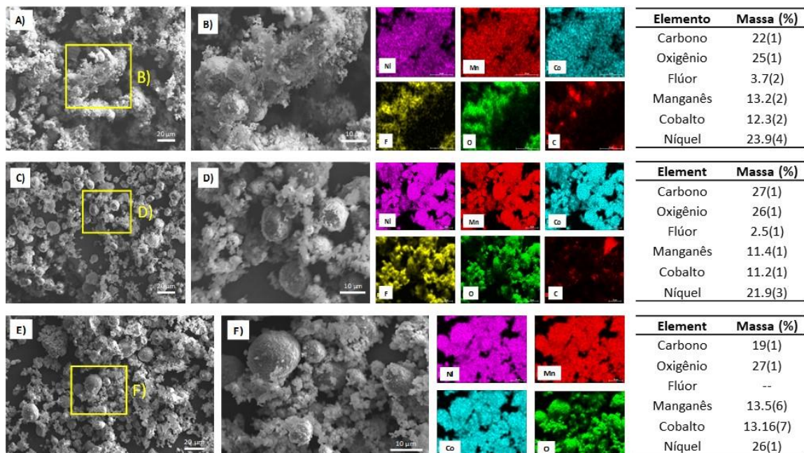
Figura 37 - Análise de MEV e EDX dos materiais do catodo QCR como-recebido (a) e (b), delaminado (c) e (d) e após a reliação (e) e (f)
