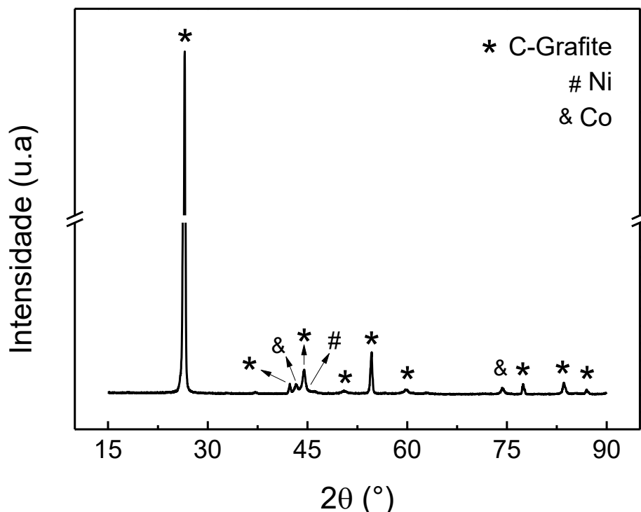
Figura 23 - Difratograma de raios-X do resíduo recuperado por filtração após a solubilização da amostra MG 4 em ácido cítrico e peróxido de hidrogênio (H 2 O 2 )
