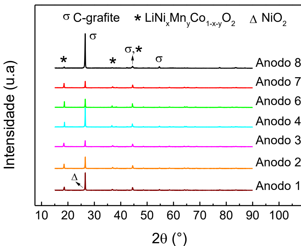
Figura 16 - Difrátogramas de raios-X dos pós extraídos dos anodos das baterias utilizadas neste estudo
