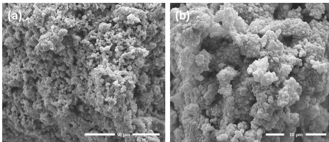
Figura 28 - Microscopia Eletrônica de Varredura dos grãos do pó de \text{Li}_1\text{Ni}_{0,5}\text{Mn}_{0,3}\text{Co}_{0,2}\text{O}_2 resintetizado a 850\text{ }^\circ\text{C} por 10 horas nos aumentos 2500x (a) e 10000 (b)
