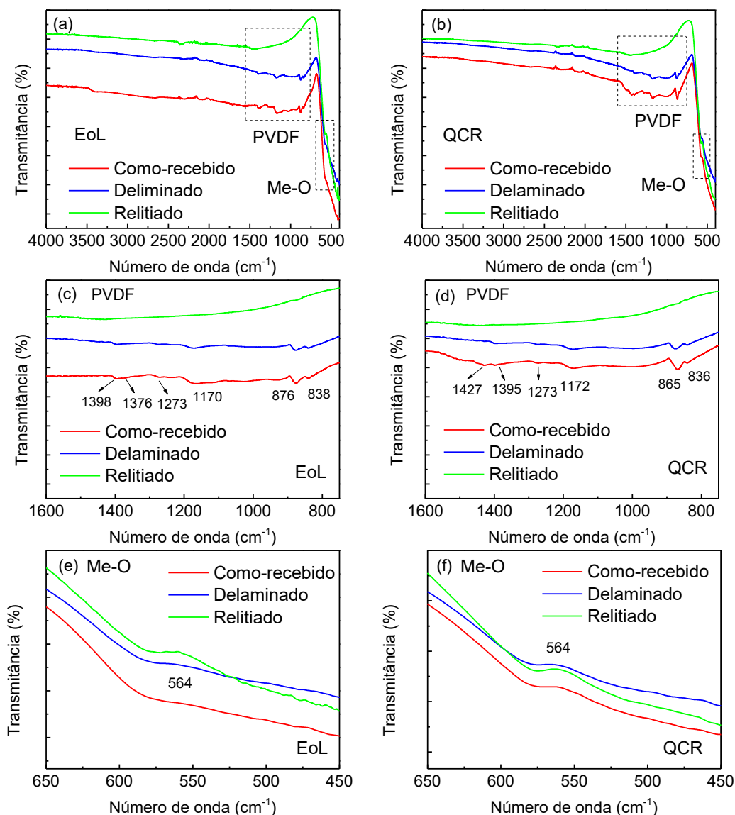
Figura 36 - Espectros de transmitância no infravermelho para os materiais de catodo QCR e EoL, nas condições: como recebidos, delaminados e relitados
