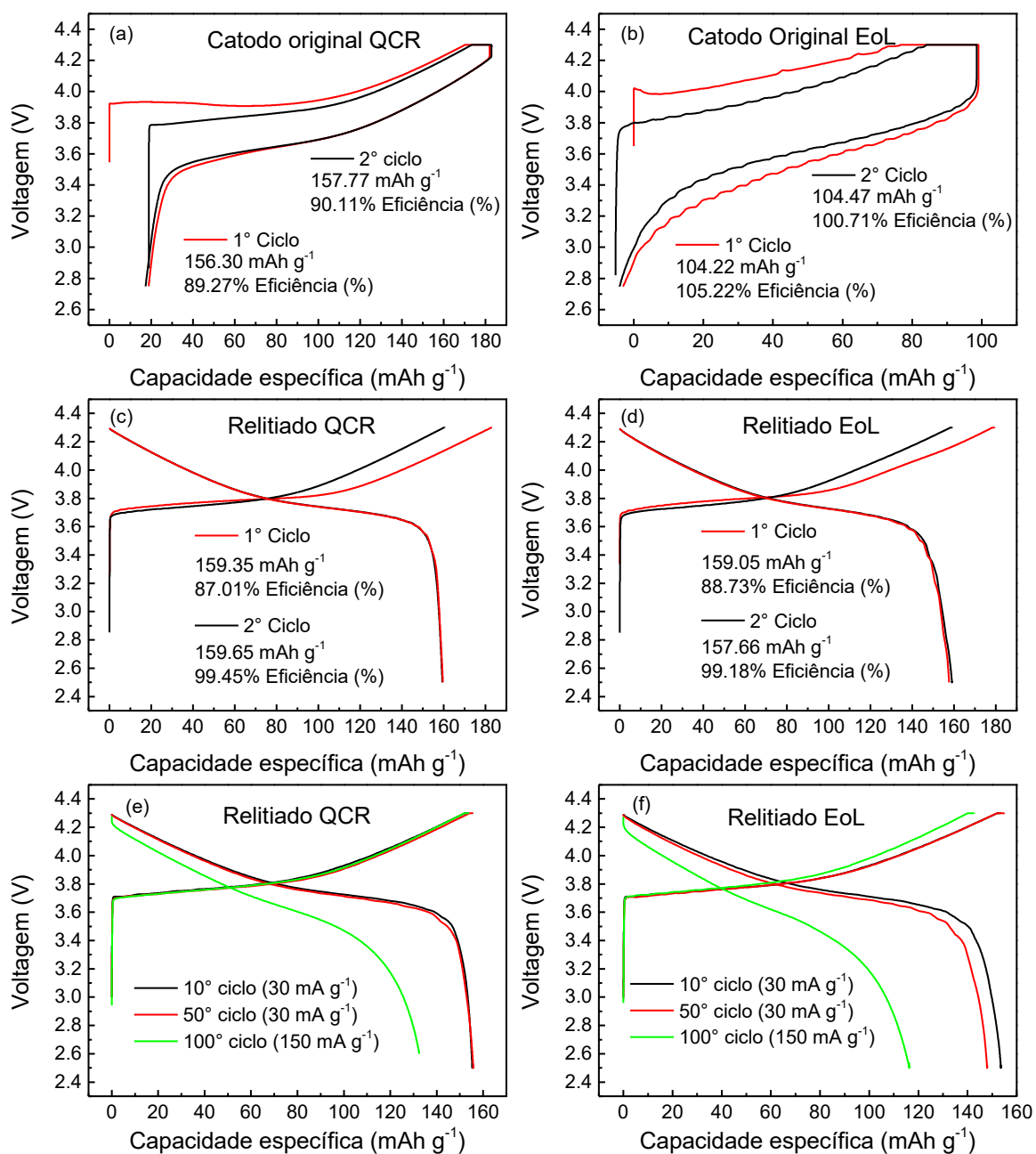
Figura 41 - Ciclos de carga-descarga de formação para os catodos originais QCR e EoL em (a) e (b), respectivamente, e para seus catodos relitiados em (c) e (d). Os ciclos de carga-descarga do 10 o , 50 o e 100 o para os catodos QCR e EoL relitiados são apresentados em (e) e (f)
