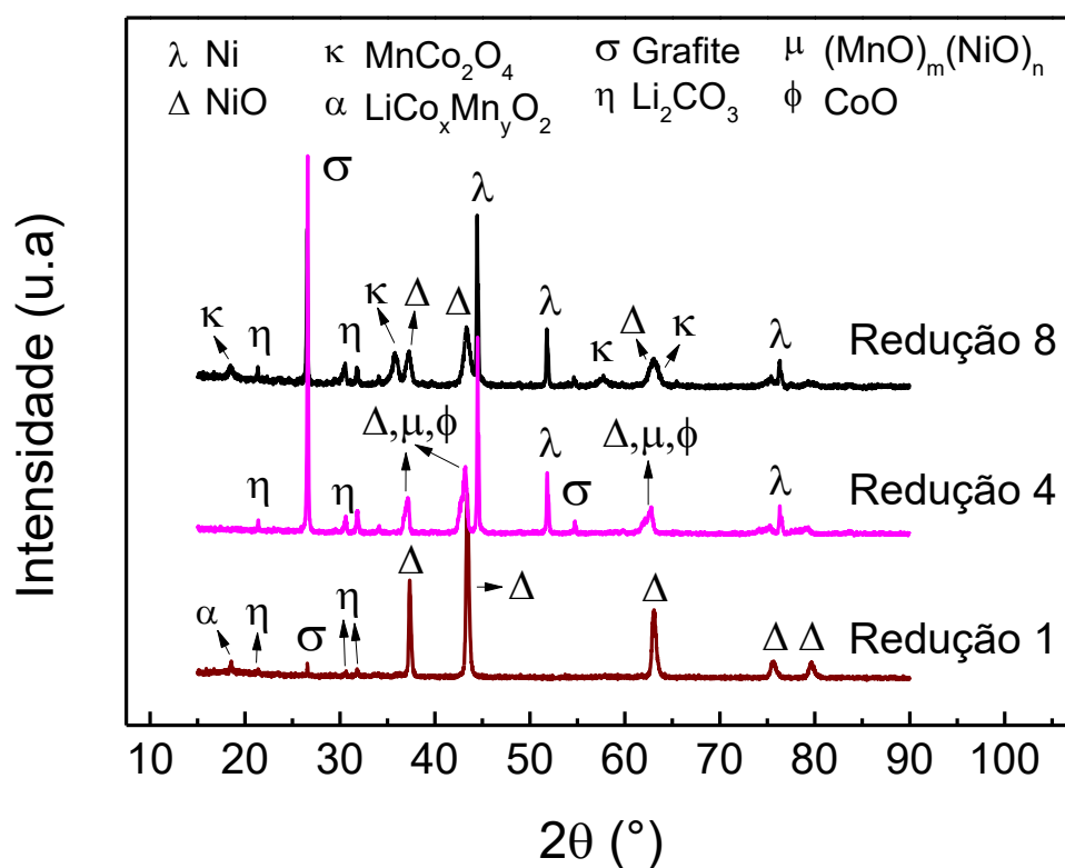
Figura 18 - Difratomogramas de raios-X dos produtos das reduções carbotérmicas do NMC/C-grafite das baterias 1, 4 e 8 realizados a 650 °C por 30 minutos sob fluxo de 0,4 L min -1 de argônio.
