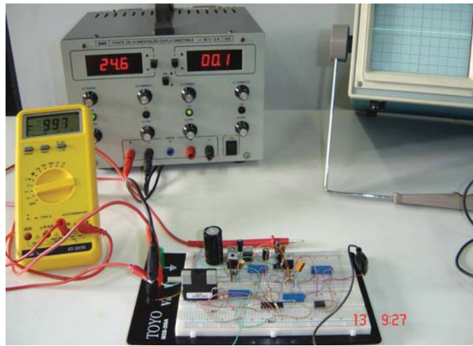
Figura 3.5: Circuito de teste do transdutor de flux de ar no primeiro plano do proto-board , e da fonte de alimentação no segundo plano.
