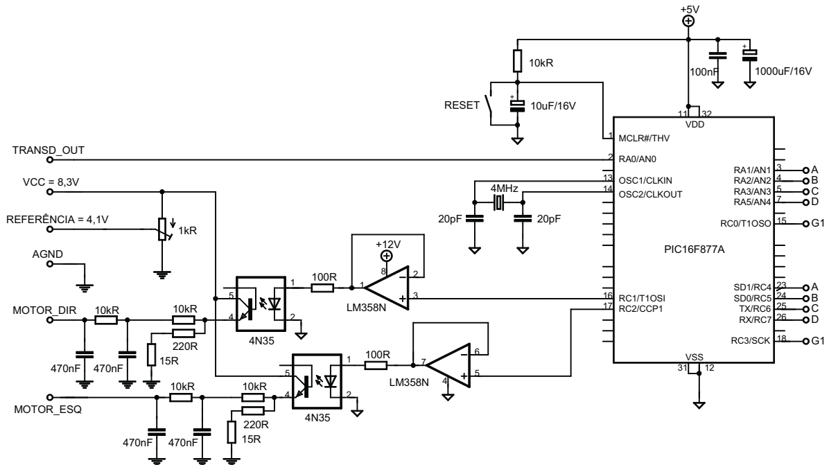
Figura 3.8: Esquemático do circuito do microcontrolador e do gerador dos sinais analógicos de controle.
