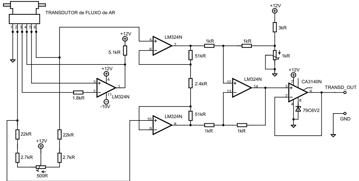
Figura 3.6: Esquemático do circuito de condicionamento do transdutor de flux de ar.
