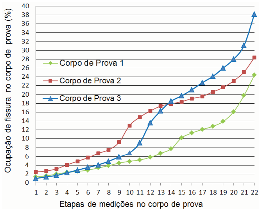
Figura 24 – Gráfico com os valores da região percentual ocupada pelas fissuras em três corpos de prova obtidos com a plataforma móvel em 22 etapas de medições.
