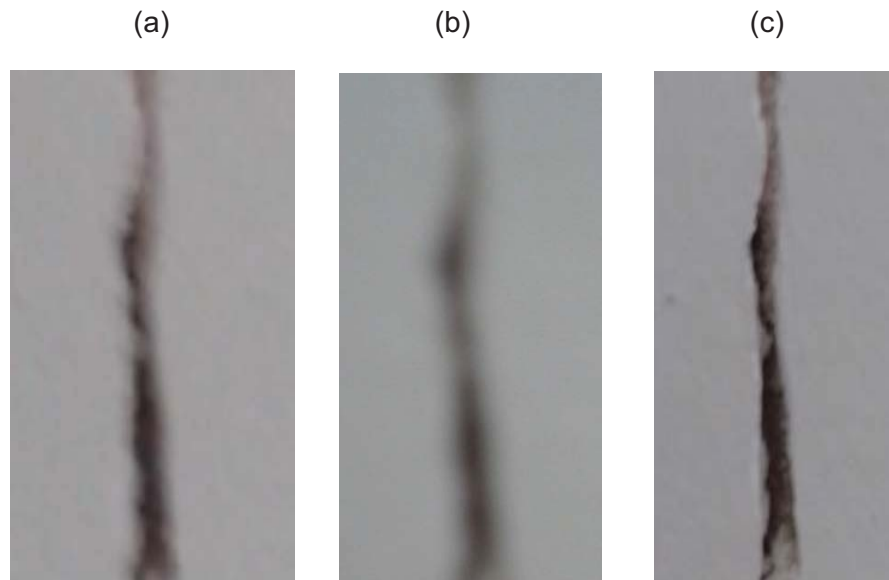
Figura 4 – Imagem de uma fissura em alvenaria com diferentes distâncias de trabalho. (a) Imagem obtida com valor acima da WD_{max} . (b) Imagem obtida com valor abaixo da WD_{min} . (c) Imagem com a distância de trabalho entre o valor mínimo ( WD_{min} ) e máximo ( WD_{max} ).
