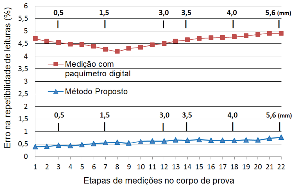
Figura 28 – Comparação de erro de repetibilidade entre o método proposto e o método convencional com o paquímetro digital, em relação às dimensões físicas das aberturas de fissuras.
