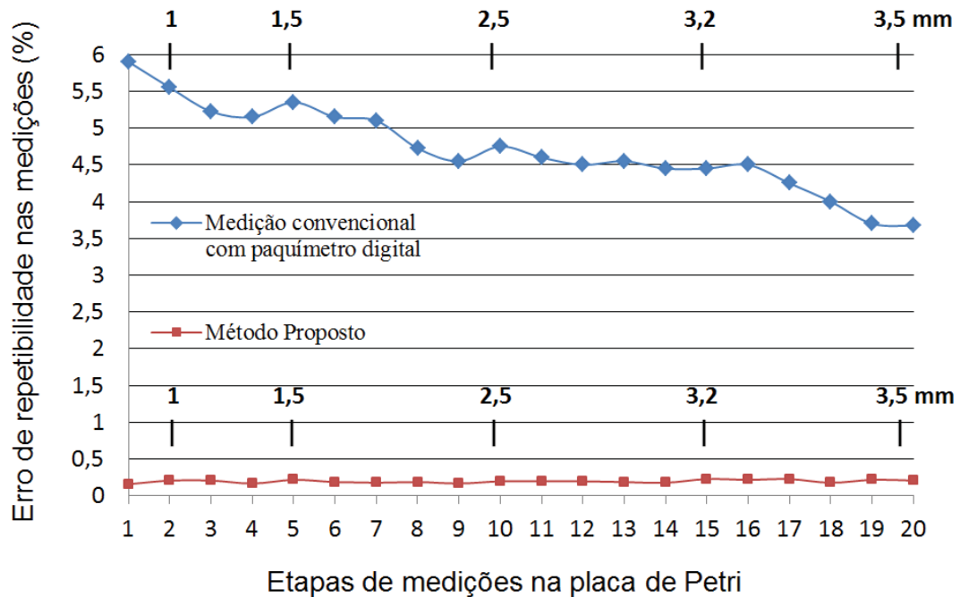
Figura 35 – Comparação de erro de repetibilidade entre o método proposto e o método convencional com o paquímetro digital em relação às dimensões físicas das colônias. Foram 20 etapas de medições na placa de Petri.
