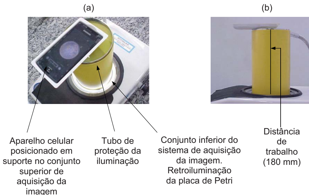
Figura 29 – Sistema aquisição de imagem com o sistema de visão proposto para monitoramento de colônias. (a). Aparelho celular posicionado sobre uma placa de Petri na base suporte com o tubo de proteção da iluminação. (b) Detalhe da distância de trabalho entre a câmera do aparelho celular e a placa de Petri localizada no conjunto inferior do sistema de aquisição da imagem.
