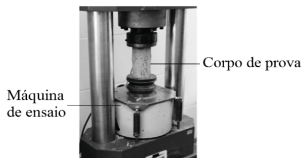
Figura 22 – Máquina de ensaio utilizada na engenharia civil para verificar comportamento e resistência à compressão em corpo de prova.
