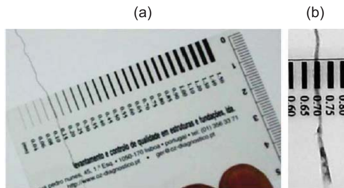
Figura 8 – Instrumento comparador de fissuras. (a) Comparador durante a medição da abertura de fissura sobre a estrutura em alvenaria avariada. (b) Detalhe da escala do instrumento comparador com a indicação de 0,70mm de abertura de fissura.
