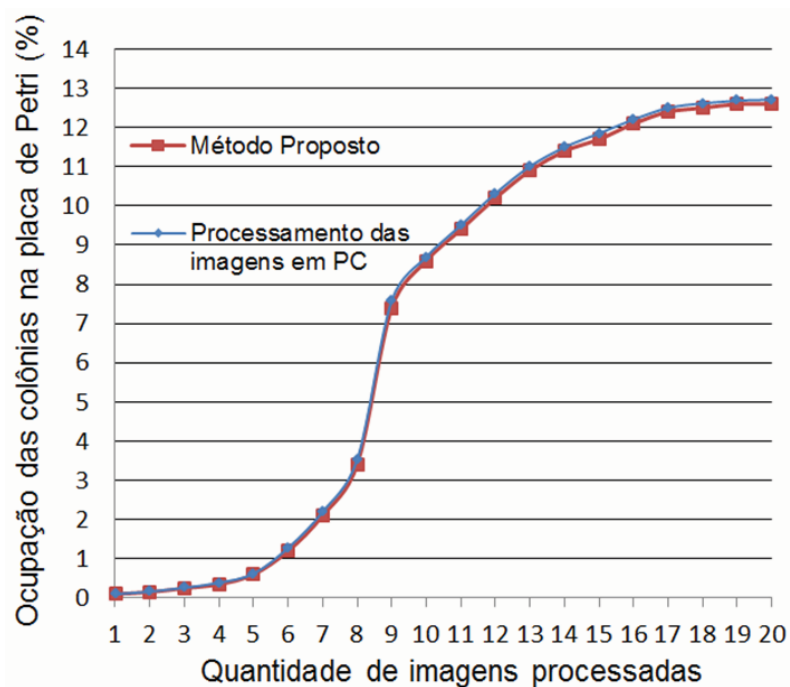
Figura 38 – Comparação de medição das imagens da placa de Petri em diluição 10^{-4} ml de S. cerevisiae entre o método proposto e o processamento das imagens em PC. Foram 20 imagens processadas.
