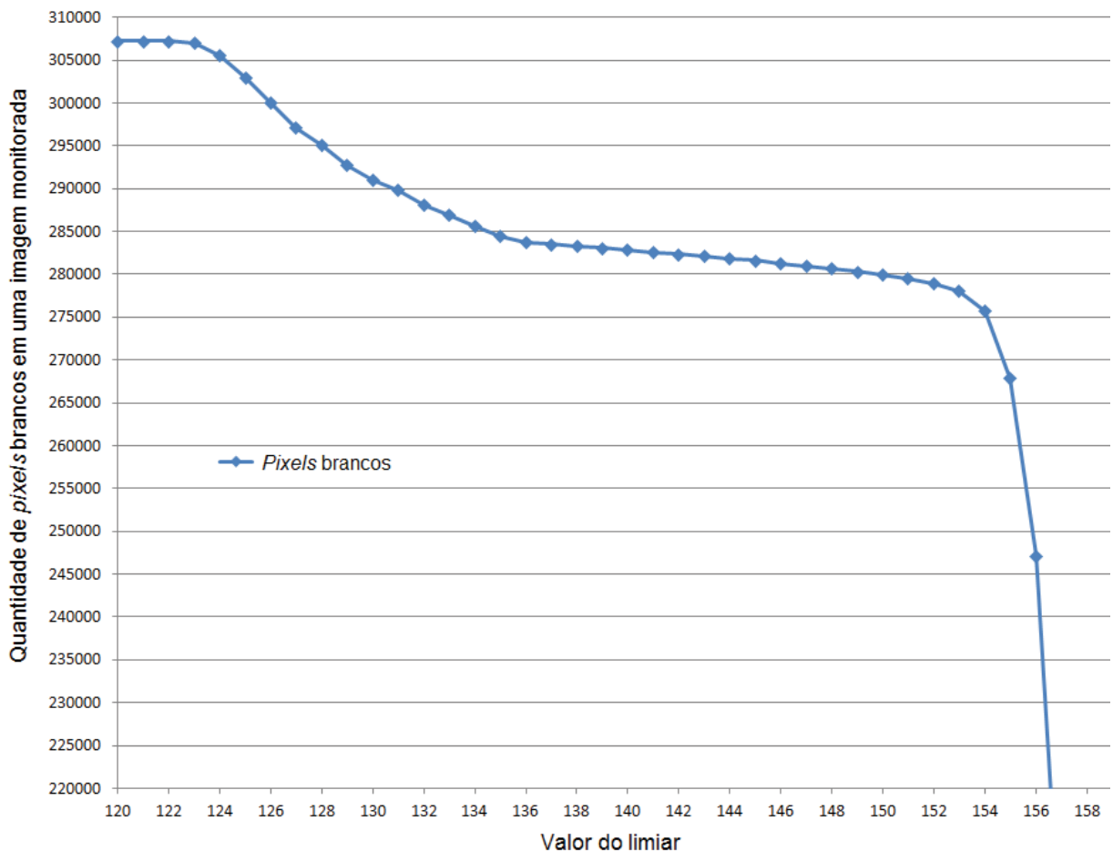
Figura 36 – Quantidade de pixels brancos em uma imagem em função da variação do valor do limiar aplicado.
