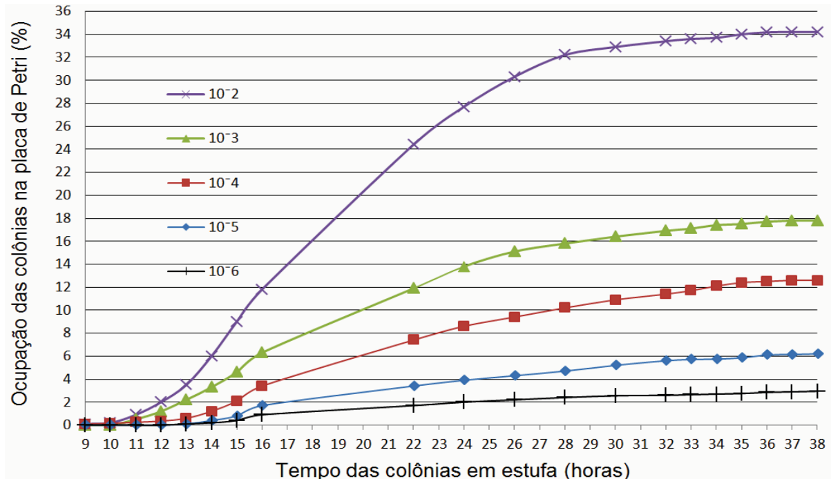
Figura 32 – Ocupação proporcional das colônias em cada placa de Petri obtido pelo sistema proposto com S. cerevisiae nas diluições: 10^{-6} , 10^{-5} , 10^{-4} , 10^{-3} e 10^{-2} ml. Foram 20 medições (fases de crescimento das colônias) entre a 9ª e 38ª hora de incubação.
