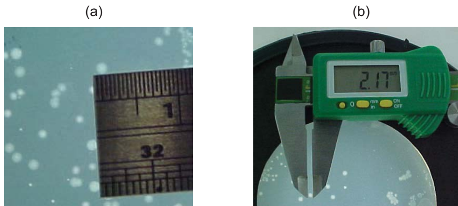
Figura 14 – Instrumentos de metrologia dimensional em medição convencional de colônia do micro-organismo S. cerevisiae . (a) Escala graduada. (b) Instrumento paquímetro digital.
