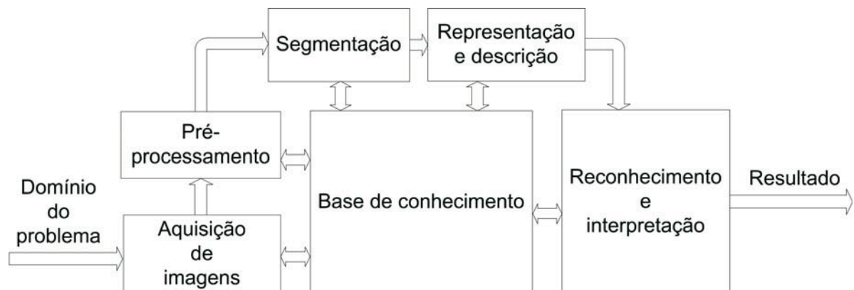
Figura 2 – Componentes de um sistema de processamento de imagens.
