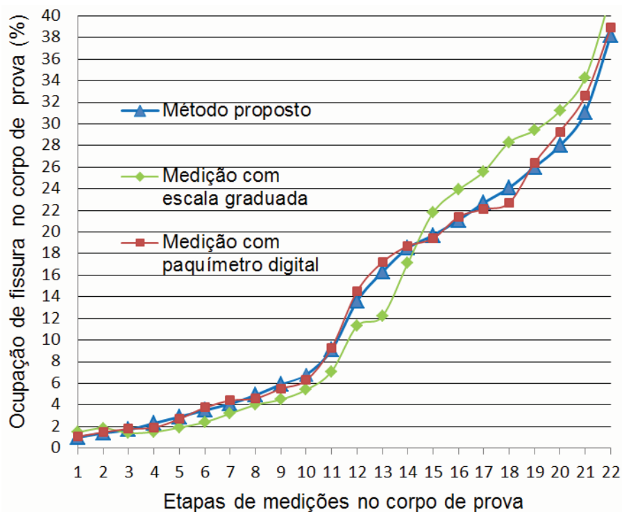
Figura 25 – Gráfico apresentando os erros médios percentuais na repetibilidade entre as medições dos técnicos (A e B) com a régua graduada, o paquímetro digital, e o sistema proposto. Foram 22 etapas de medição, durante o monitoramento de fissuras no corpo de prova número 3.
