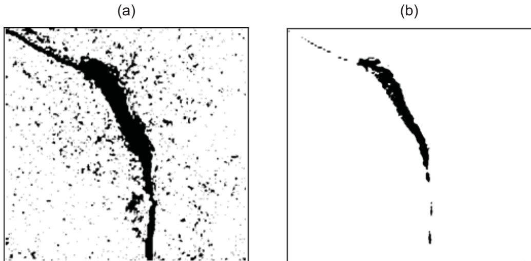
Figura 19 – Imagem binária da fissura em alvenaria com diferentes limiares. (a) Imagem binária de uma fissura em alvenaria com valor do limiar em 154, apresentando características do fundo da imagem. (b) Imagem binária de fissura em alvenaria aplicando o valor de limiar 138, perdendo forma na fissura.
