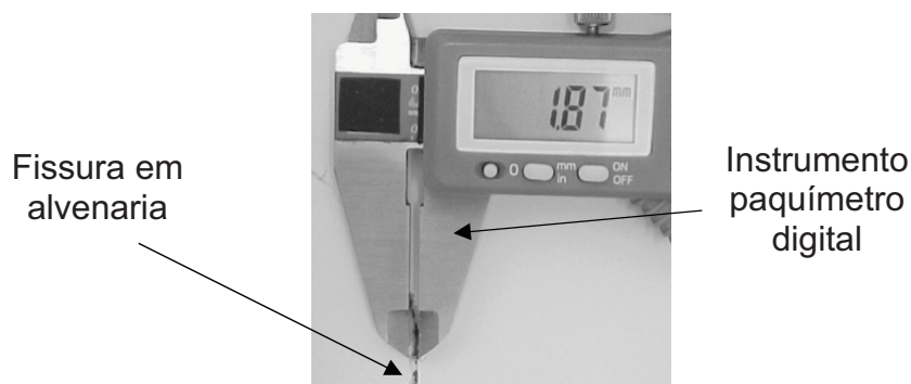
Figura 9 – Instrumento paquímetro digital em medição convencional da abertura da fissura em alvenaria. A dimensão da fissura é indicada no visor após posicionamento do instrumento sobre a fissura na estrutura avariada.
