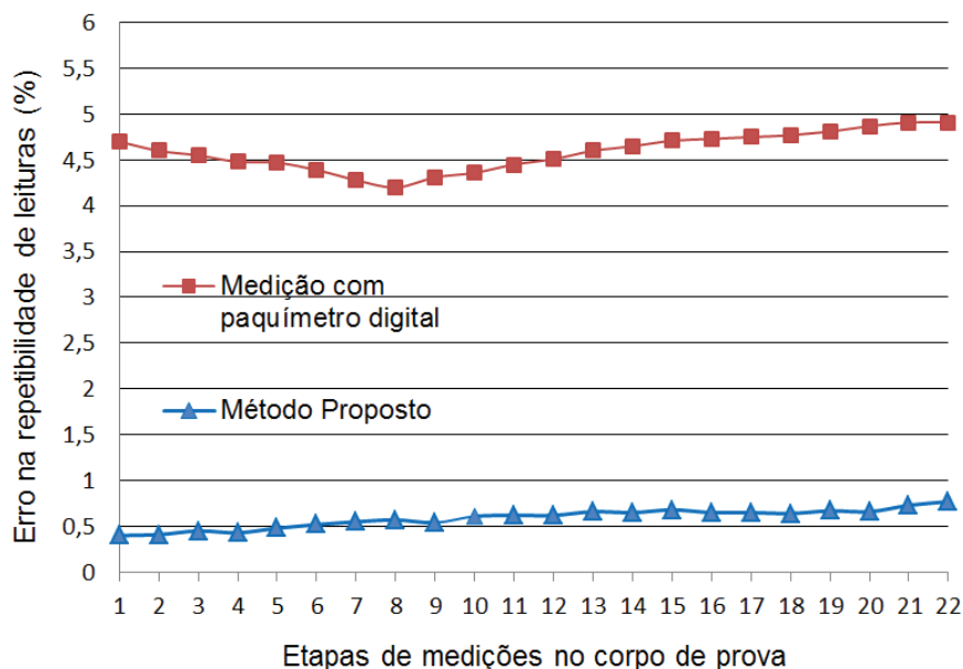
Figura 26 – Gráfico com os valores de erros de repetibilidade de medições de fissura no corpo de prova. No total, foram realizadas 22 etapas de comparações entre o paquímetro digital e o método proposto.
