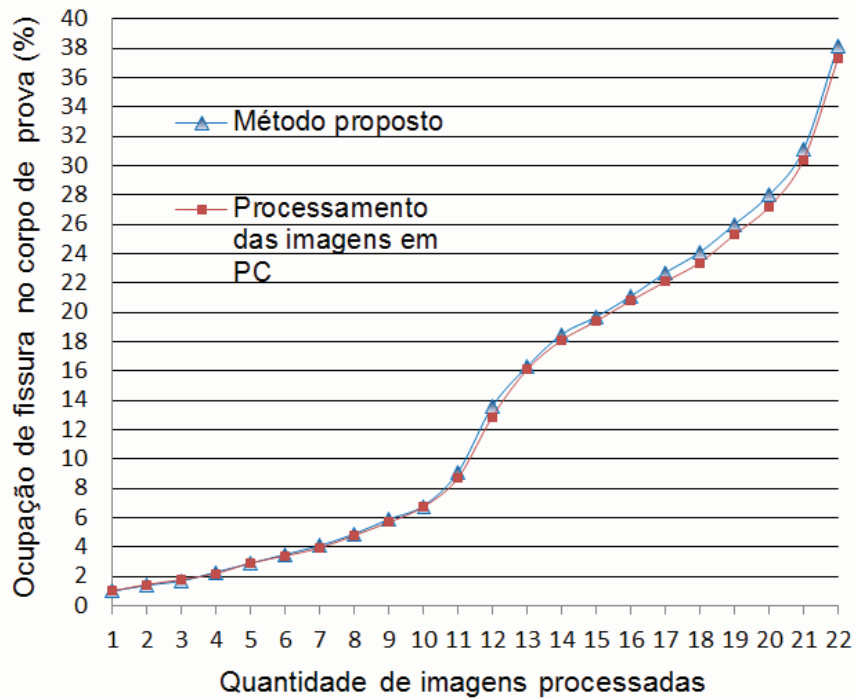
Figura 37 – Comparação de medição entre as imagens do corpo de prova número 3 no método proposto e o processamento das imagens no PC. Foram 22 imagens processadas.
