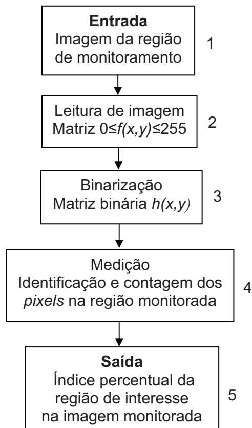
Figura 17 – Diagrama em blocos do processamento digital da imagem no sistema de monitoramento proposto.
