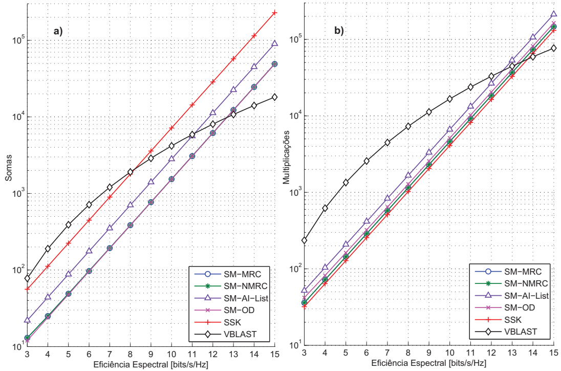
Figura 4.4: Complexidade em termos de número de operações complexas para esquemas SM e V-BLAST com BPSK e r \in [3 : 15] [bits/s/Hz]. a) Somas complexas; b) Multiplicações complexas.
