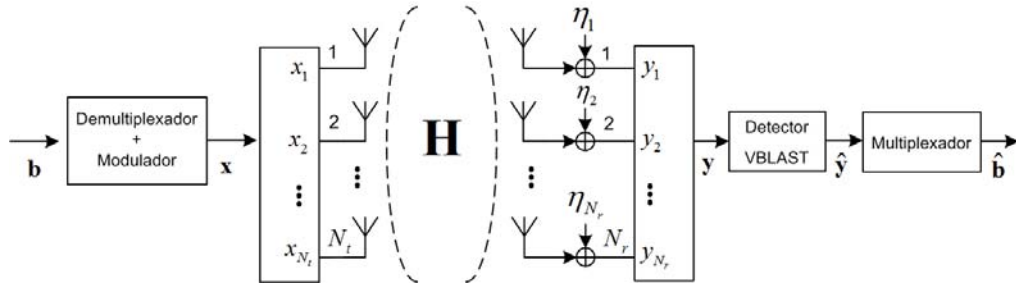
Figura 3.1: Modelo topológico para V-BLAST.
