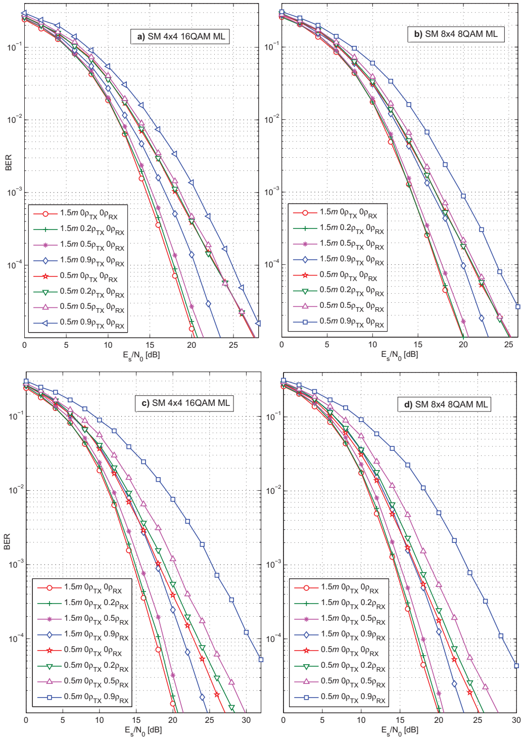
Figura 5.13: Desempenho BER para detector ótimo SM em canal Nakagami- m correlacionado ( r = 6 [bits/s/Hz], N_r = 4 ). Correlação no transmissor: a) N_t = 4 , M = 16 e b) N_t = 8 , M = 8 ; Correlação no receptor: c) N_t = 4 , M = 16 e d) N_t = 8 , M = 8 ;
