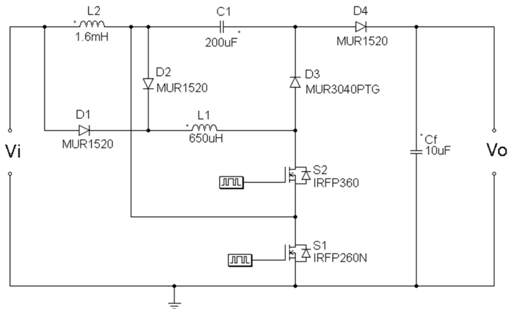
Figura 59 – Circuito de potência.
