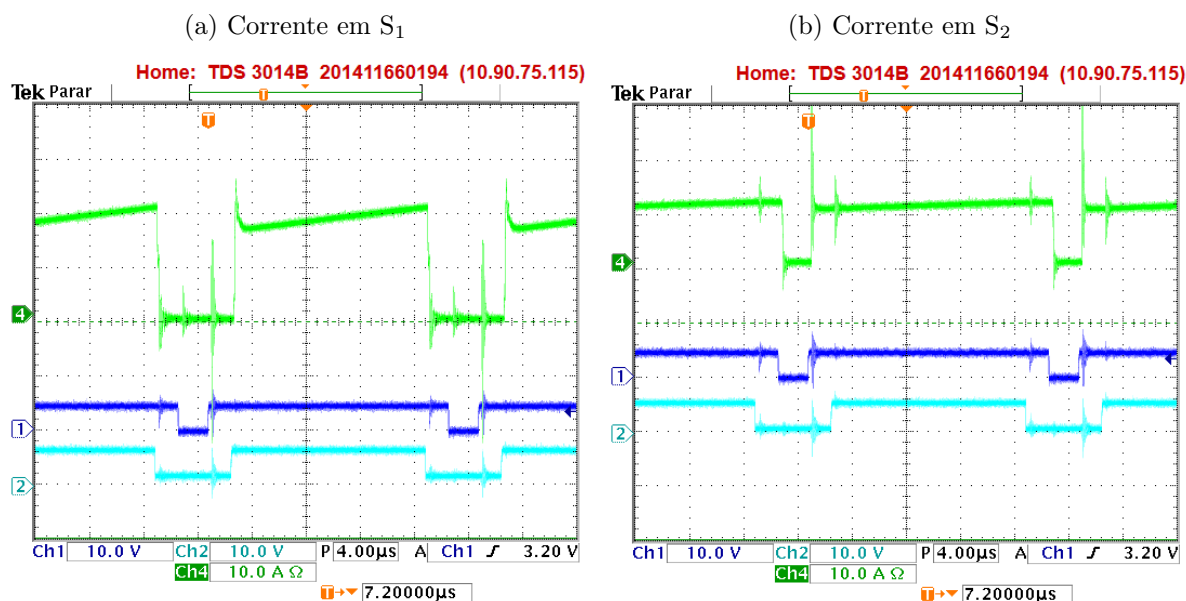
Figura 76 – Correntes nos interruptores S_1 e S_2 .
