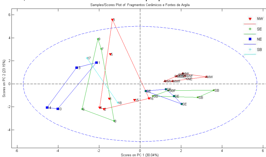
Figura 88 – Scores com as fontes de argila e fragmentos cerâmicos encontrados nas senzalas NW, NE, e SE na fazenda do Colégio dos Jesuítas e as SB da fazenda de São Bento, na análise sem os dados de Fe com pré-processamento auto escalamento.
