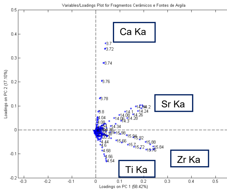
Figura 52 – Loadings com os fragmentos e fontes de argila encontradas nas senzalas NW, NE, e SE na fazenda do Colégio dos Jesuítas e as SB da fazenda de São Bento, na análise sem os dados de Fe e pré-processamento de dados centrados na média.
