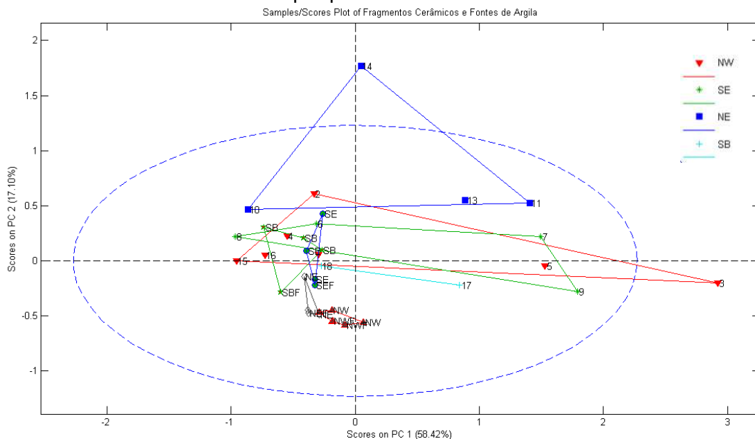
Figura 51 – Scores com os fragmentos e fontes de argila encontradas nas senzalas NW, NE, e SE na fazenda do Colégio dos Jesuítas e as SB da fazenda de São Bento sem os dados de Fe e pré-processamento de dados centrados na média.
