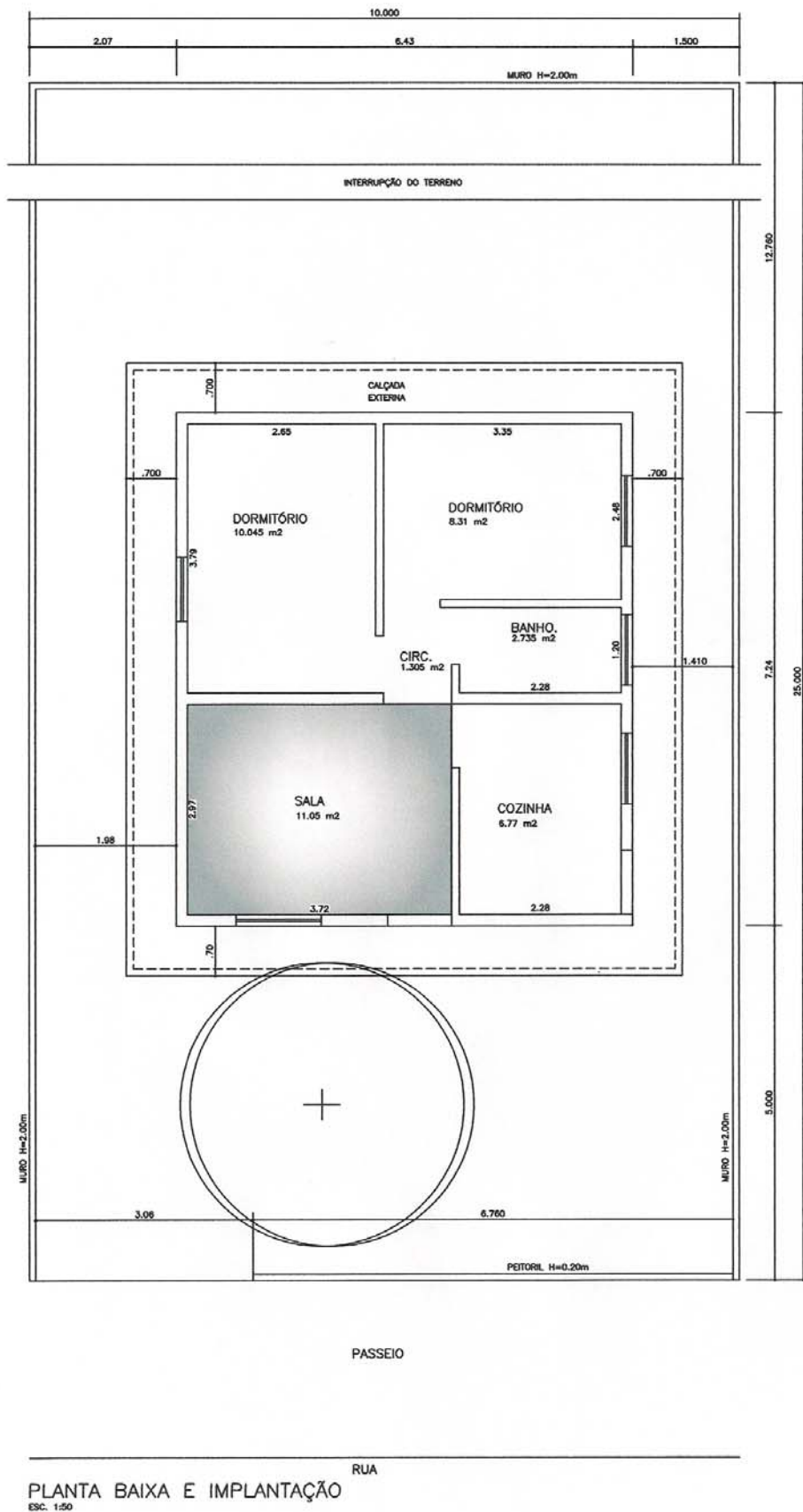
Figura 17 - Planta Baixa e Implantação genérica da casa tipo 1. Fonte: COHAB, 2009.
