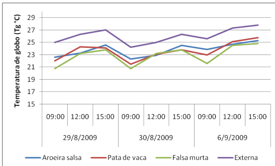
Figura 22 - Temperatura de globo (Tg °C) das três espécies arbóreas.
