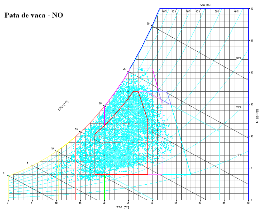
Figura 28 - Carta bioclimática do ambiente interno referente à situação Pata de vaca na face NO.
