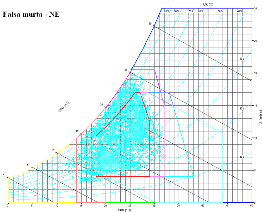
Figura 30 - Carta bioclimática do ambiente interno com a presença do elemento de sombreamento Falsa murta na face NE.
