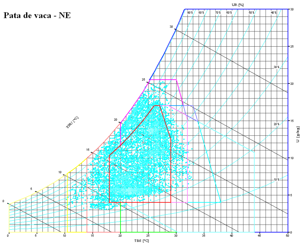
Figura 32 - Carta bioclimática do ambiente interno com a presença do elemento de sombreamento Pata de vaca na face NE.
