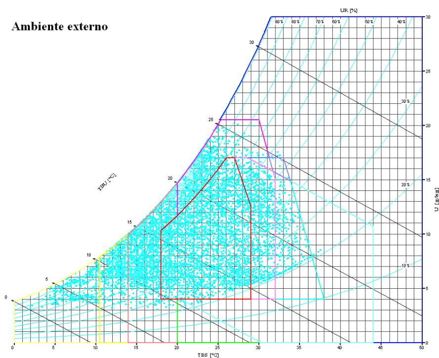
Figura 24 - Carta bioclimática do ambiente externo válido como referência para todas as situações.
