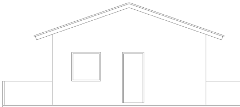
Figura 15 - Elevação frontal da casa tipo 1. Fonte: COHAB, 2009.
