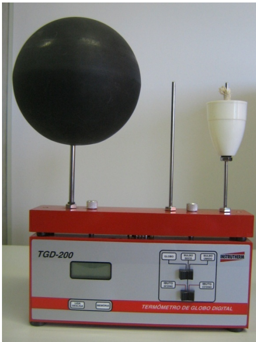
Figura 12 - Termômetro de globo da Instrutherm modelo TGD 200.
