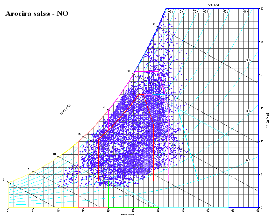
Figura 27 - Carta bioclimática do ambiente interno referente à situação Aroeira salsa na face NO.
