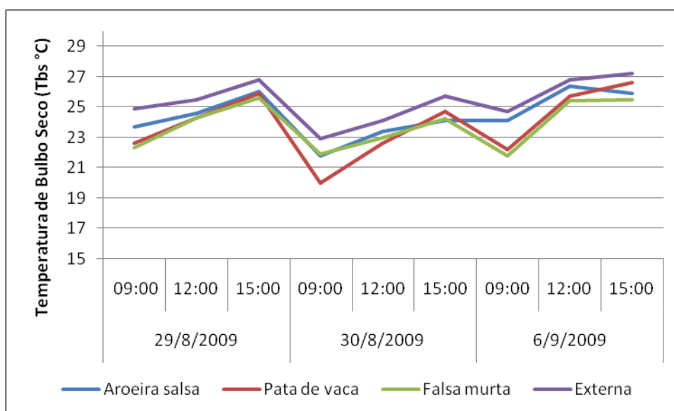
Figura 23 - Temperatura de bulbo seco (Tbs °C) das três espécies arbóreas.
