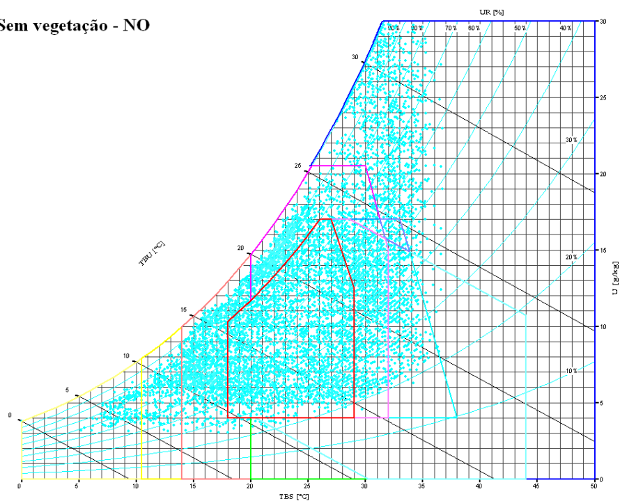
Figura 25 - Carta bioclimática do ambiente interno referente à situação sem vegetação na face NO.
