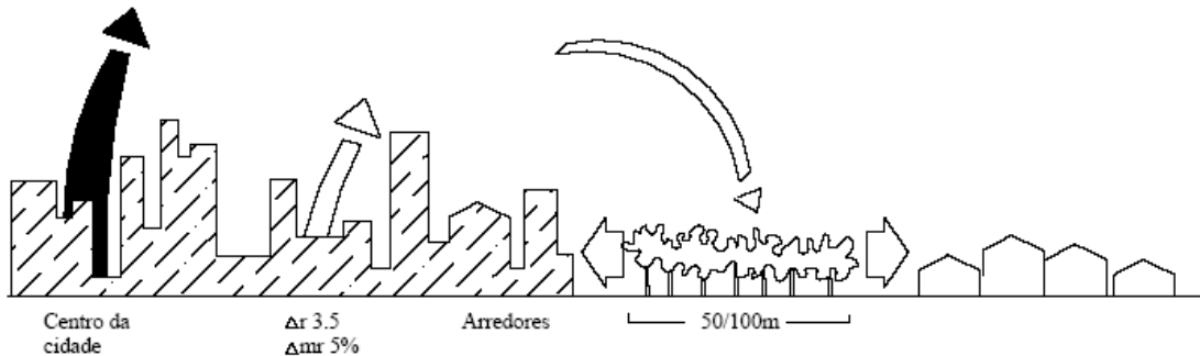
Figura 3 - Efeito do umedecimento do ar por uma área com vegetação.
