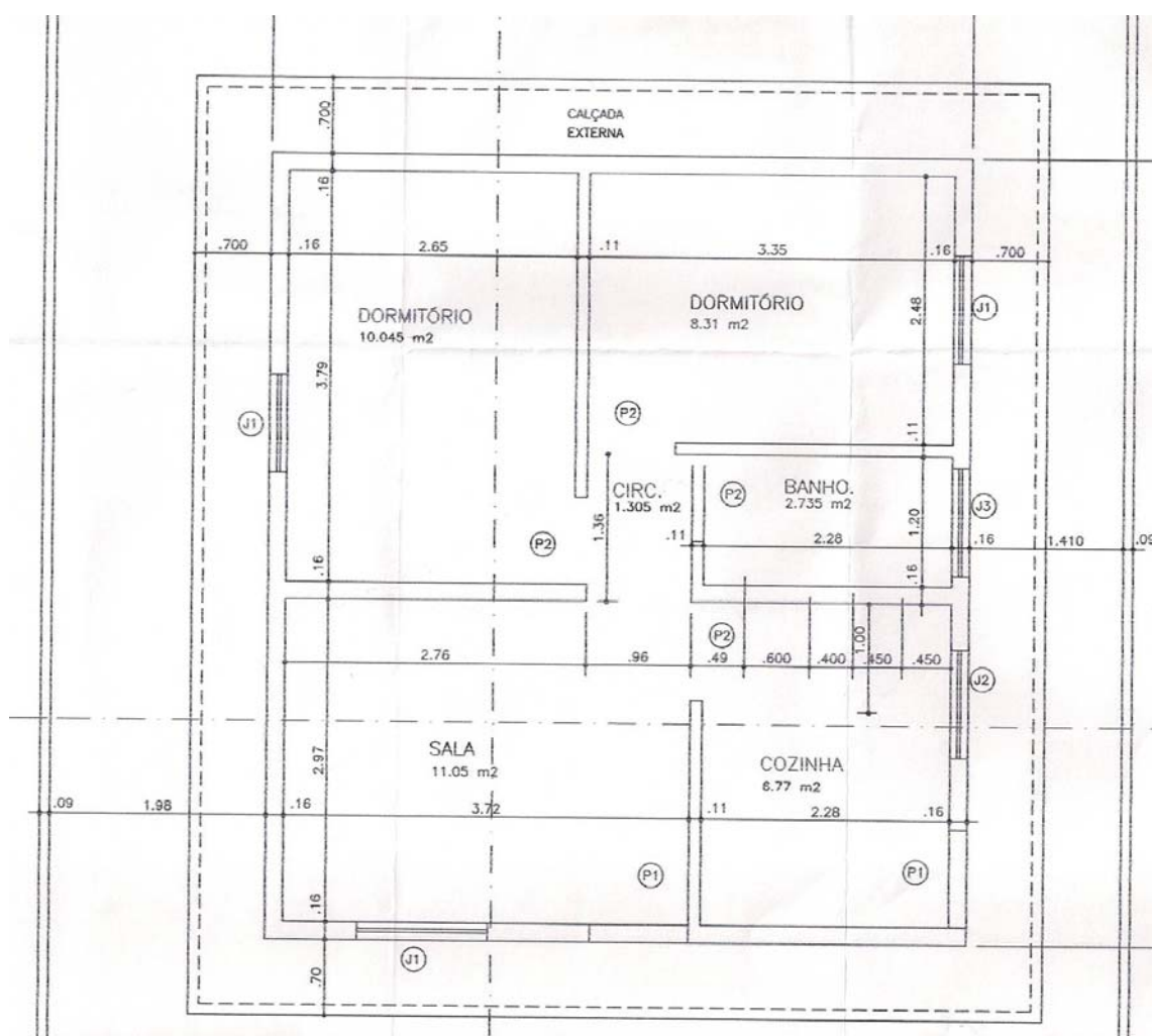
Figura 14 - Planta Baixa da casa tipo 1.
