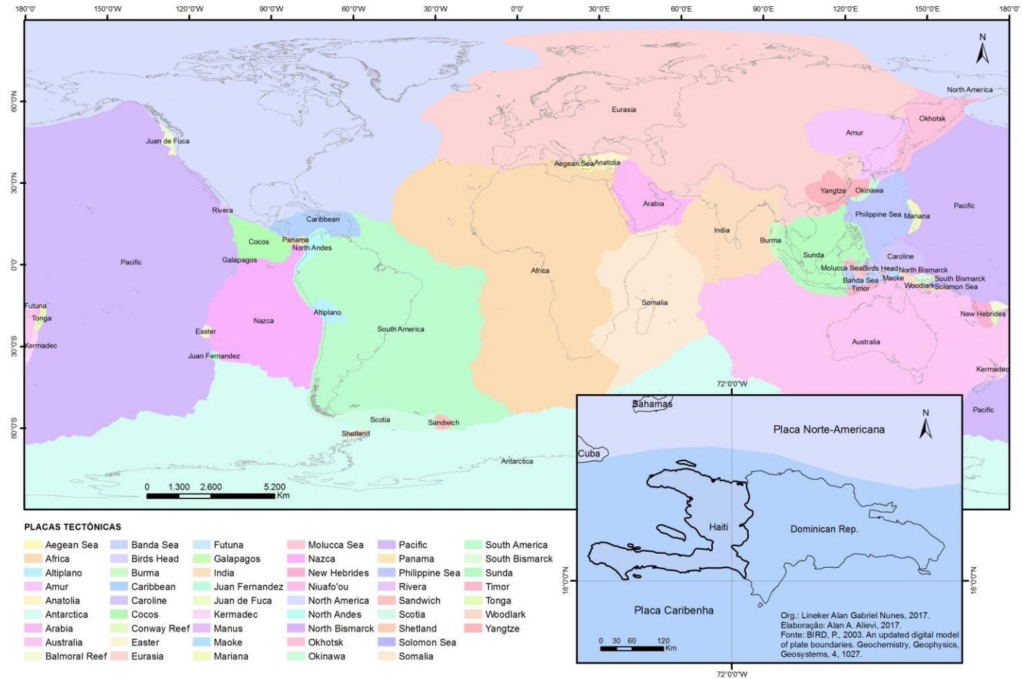
Figura 5 - Localização das Placas Tectônicas
