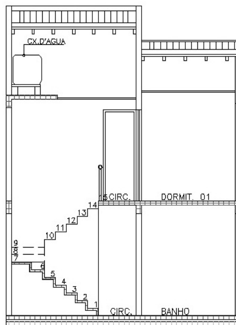
Figura 9 – Esquema de um corte.
