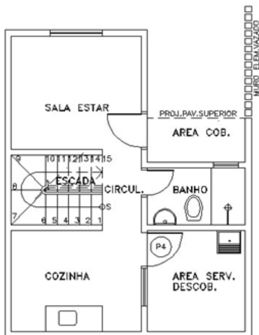
Figura 7 – Planta baixa do pavimento térreo
