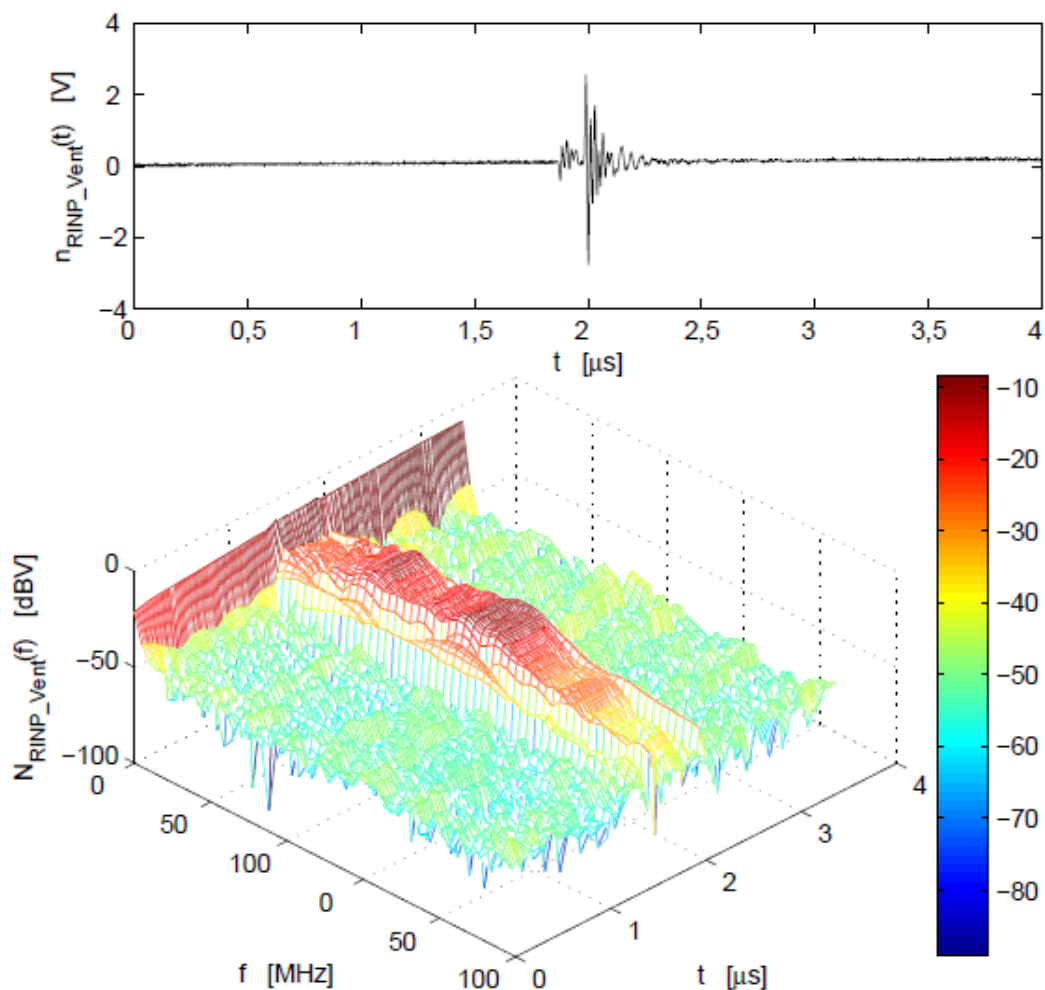
Figura 4.5 – Comportamento impulsivo e espectral do RINP gerado pelo desligamento de um ventilador de mesa de 60W.
