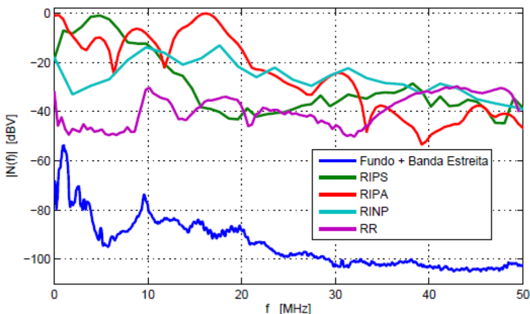
Figura 4.11 – Faixas de magnitudes espectrais medias relativas as ocorrências de cada ruído analisado.
