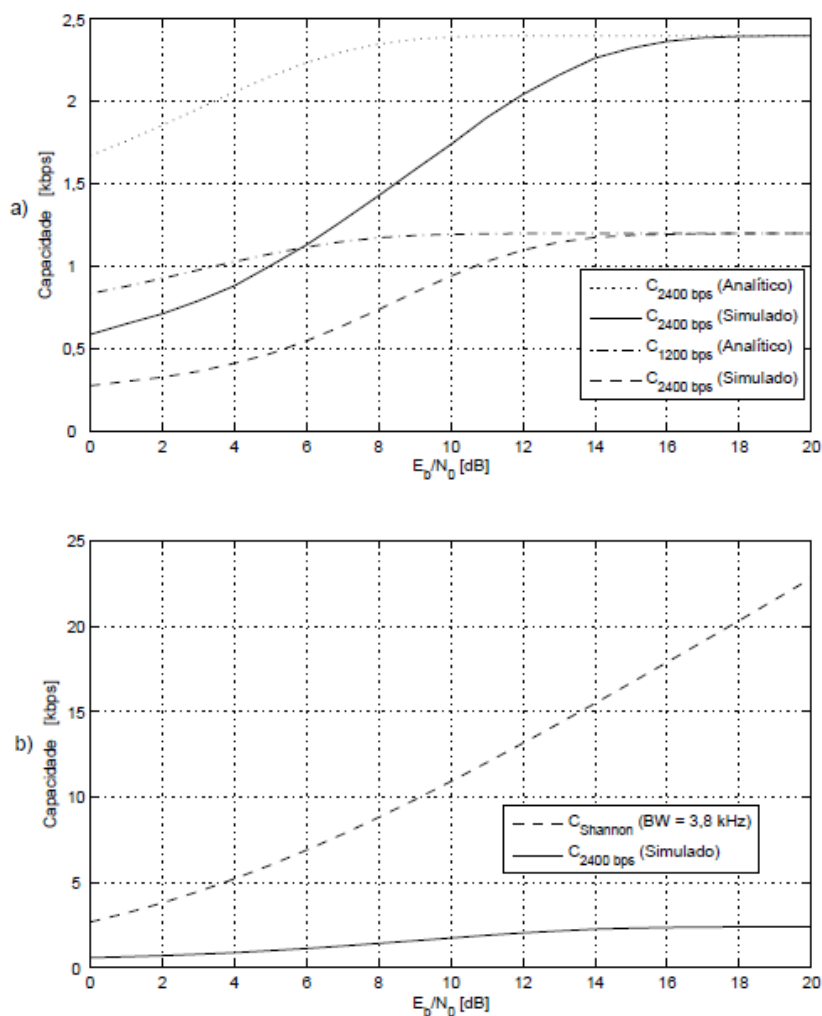
Figura 5.13 – Comparações entre a capacidade do sistema obtida por simulacao com o analítico em a), e com o limite teorico em b).
