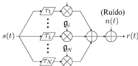
Figura 2.3 – Diagrama do modelo por eco representando o caminho multipercursos.
