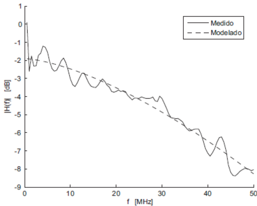
Figura 3.8 – Medicao e modelagem da atenuacao de um canal de 18, 2m sem derivacao
