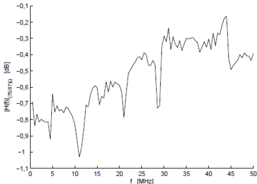
Figura 3.7 – Resposta em magnitude espectral do transformador de impedancia de linha de 75 \Omega para 87 \Omega .
