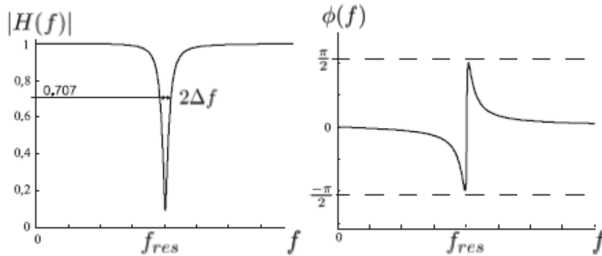
Figura 2.7 – Magnitude e fase da funcao de transferencia para um bloco SR.
