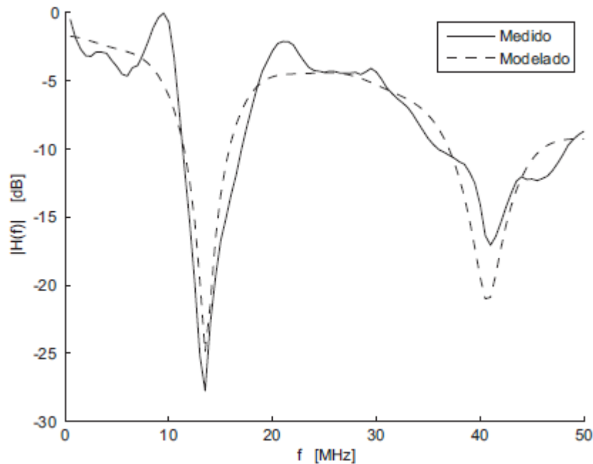
Figura 3.9 – Medicao e simulacao da resposta em frequencia para 4 percursos.
