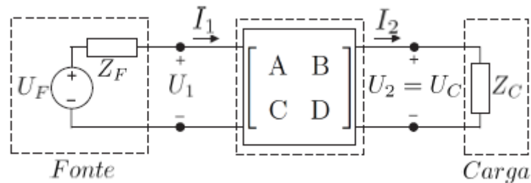
Figura 2.9 – Rede de duas portas conectada a uma fonte de tensão e carga.
