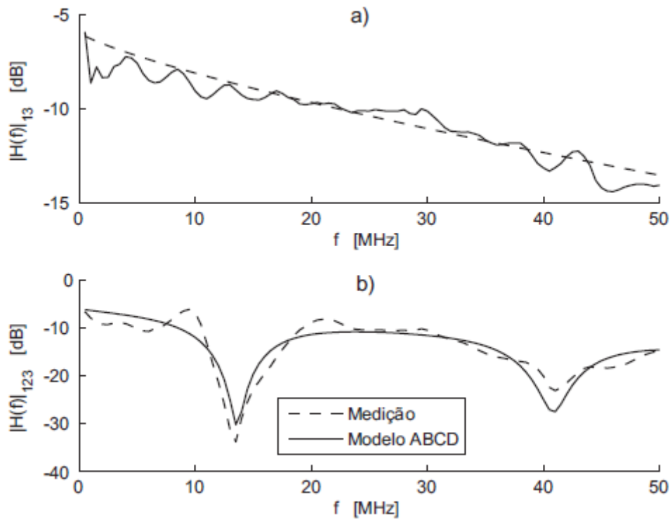
Figura 3.13 – Resposta em magnitude da medicao e do modelo sem derivação em a) e com derivação em b).
