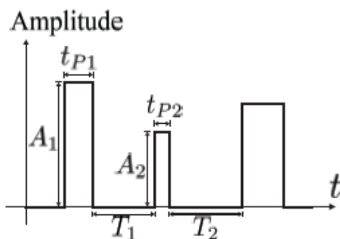
Figura 2.19 – Envoltória do ruído impulsivo não periódico.
