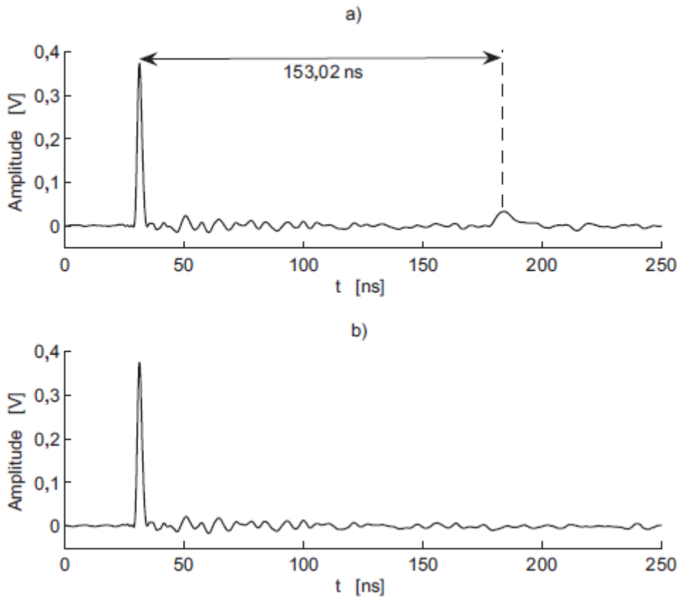
Figura 3.14 – Refletometria de canal de 18, 2m sem derivacao: terminacao em aberto em a), com terminador resistivo de 125, 9 em b).
