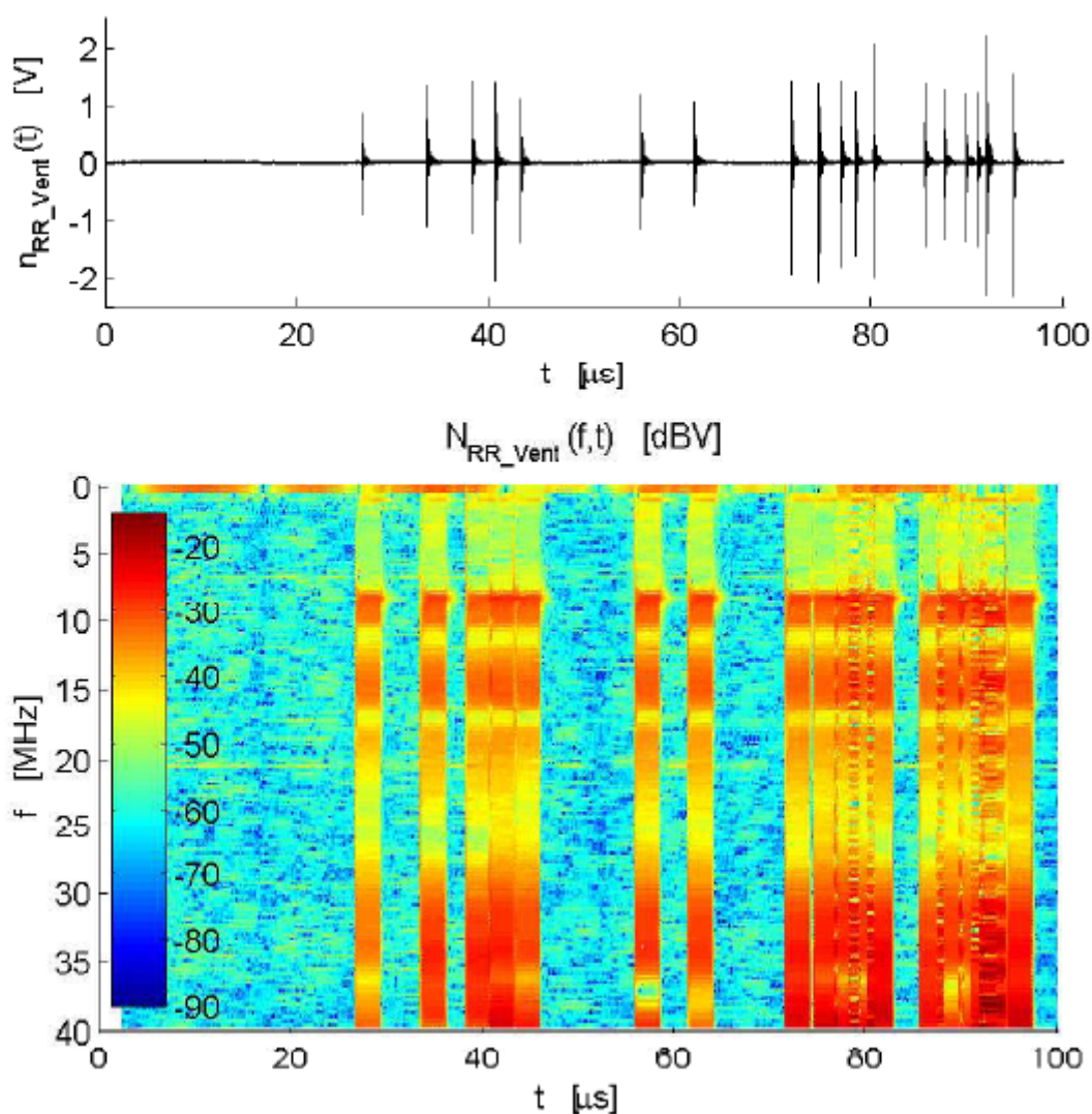
Figura 4.7 – RR gerado pelo acionamento de um ventilador.
