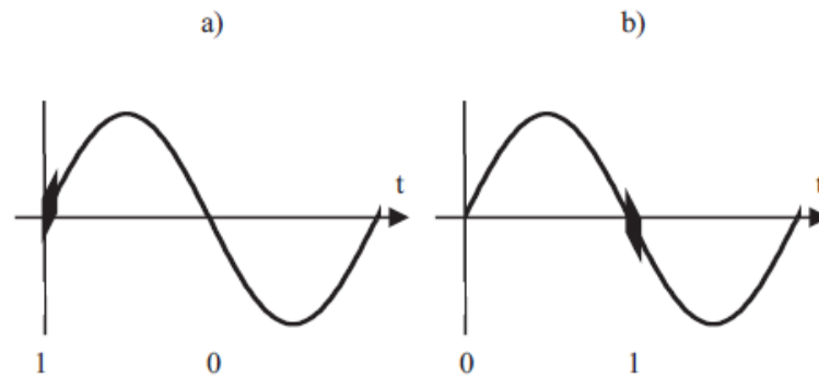
Figura 2.26 – Um bit dos codigos da casa ou do dispositivo/funcao do protocolo X10. Bit 1 e seu complementar em a), bit 0 e seu complementar em b).
