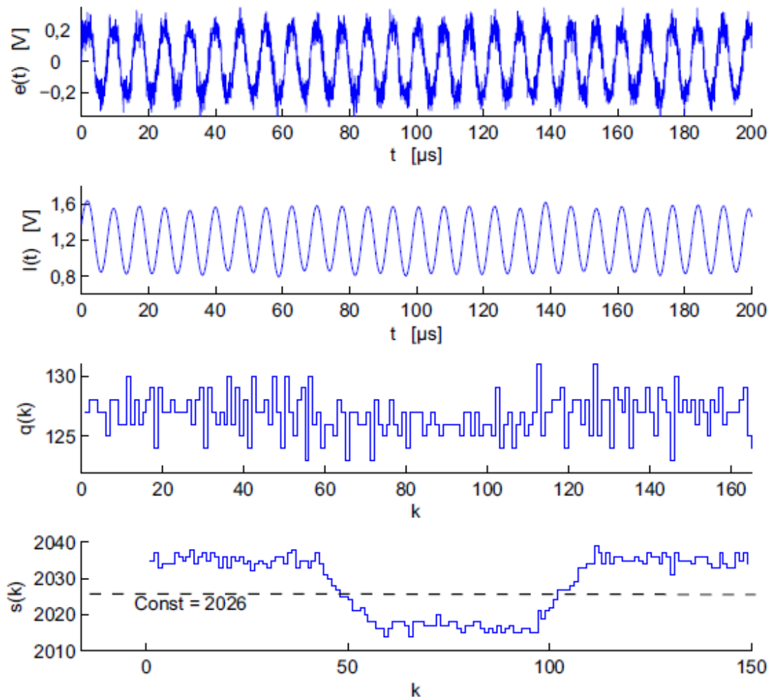
Figura 5.9 – Principais sinais gerados pelo script do receptor para SNR de 10 dB.
