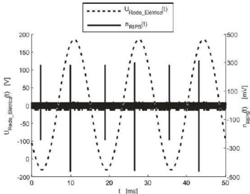
Figura 2.13 – Ruído impulsivo sincrono medido em uma TUG residencial
