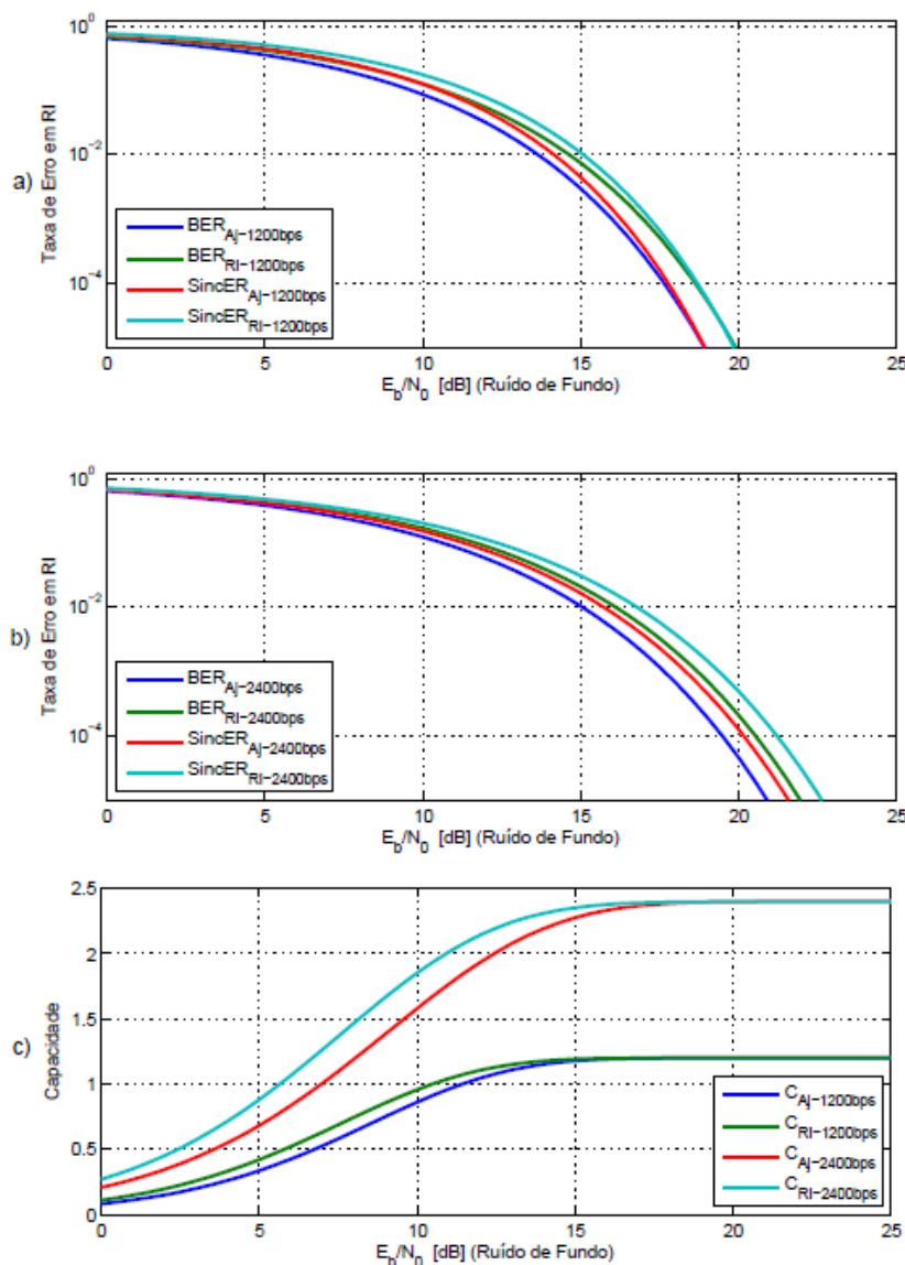
Figura 5.14 – Probabilidades de erro obtidas pelo ajuste das curvas de simulação do sistema proposto e também quando submetido ao modelo que inclui os ruídos impulsivos nas taxas de transmissão de 1200 bps em a), e de 2400 bps em b). Em c) e apresentado a capacidade do sistema.
