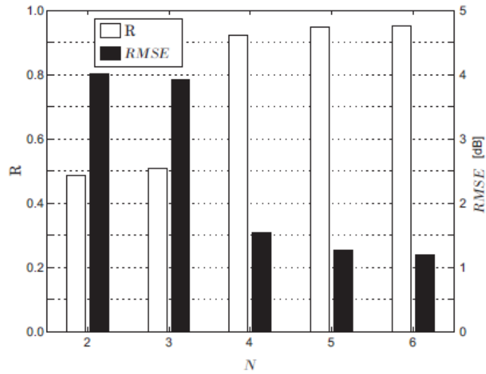
Figura 3.11 – Correlacao R e RMSE para diferentes numeros N de BSRs.
