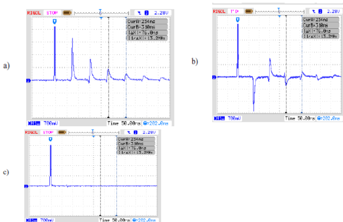
Figura 3.5 – Refletometria em um cabo coaxial de 50\ \Omega de 7,5\text{ m} .
