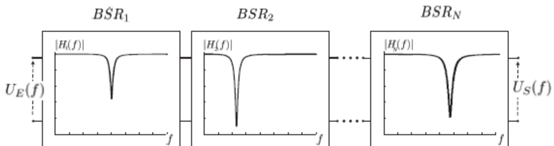
Figura 2.8 – Modelo por blocos serie ressonantes.
