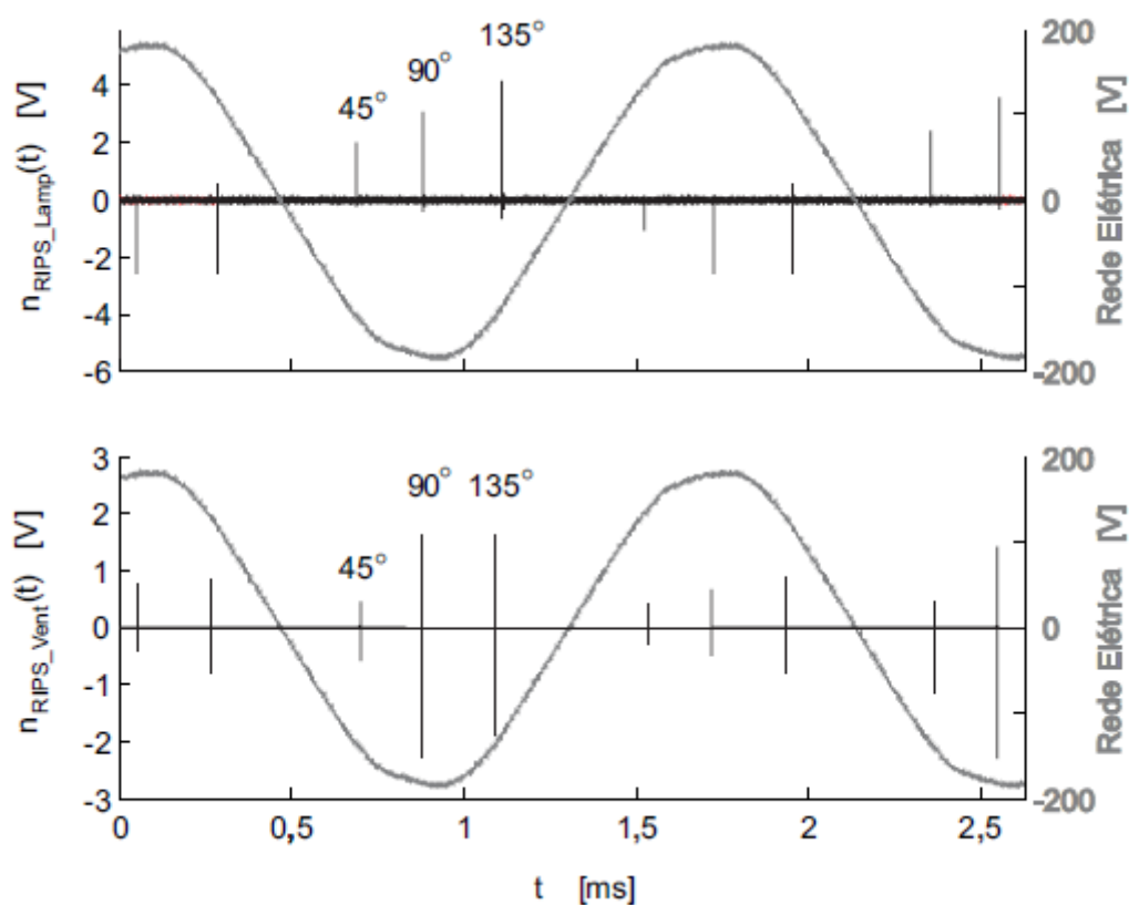
Figura 4.2 – RIPS gerado por um dimmer para ângulos de disparo próximos a 45o, 90o e 135o, para uma lampada incandescente e para um ventilador de mesa.
