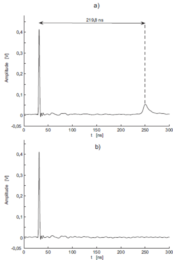
Figura 3.6 – Refletometria de canal de 18, 2m sem derivacao: a) terminação em aberto e b) com terminador resistivo de 87,9Ω.
