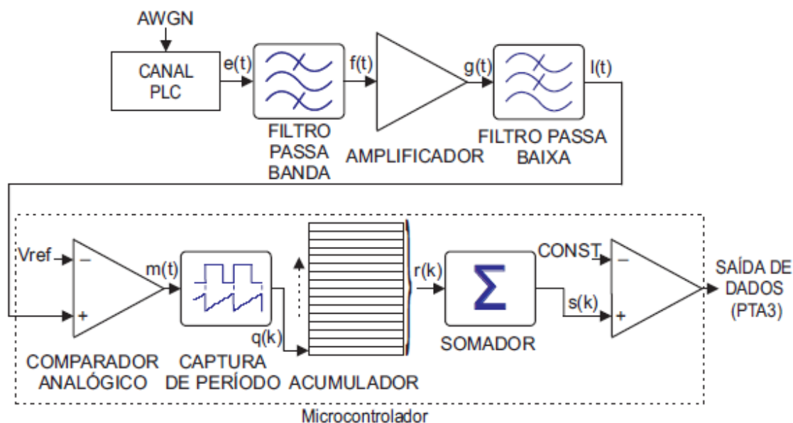
Figura 5.2 – Diagrama de blocos do receptor KNX proposto.
