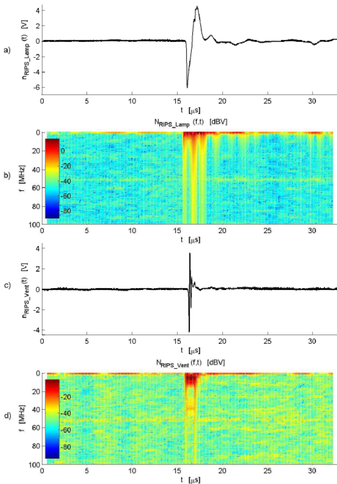
Figura 4.3 – Ruído no tempo e sua magnitude espectral ao longo do tempo de um pulso de ruído RIPS gerado por um dimmer acionando uma lampada em a) e b), e um ventilador em c) e d).
