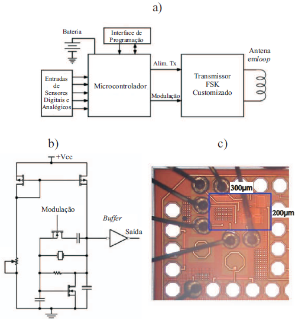
Figura 2.29 – Diagrama de blocos do sistema transmissor em a), diagrama elétrico do transmissor em b) e foto com ampliação de 20X do chip transmissor em c) (COHN et al., 2010).
