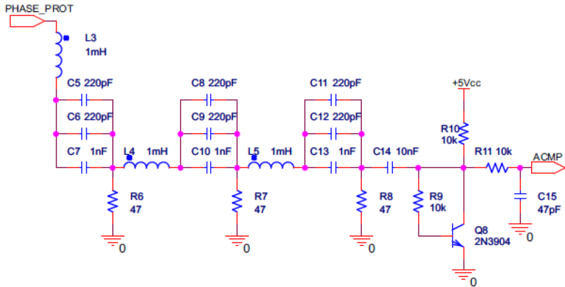
Figura 5.6 – Diagrama elétrico do circuito de recepcao.
