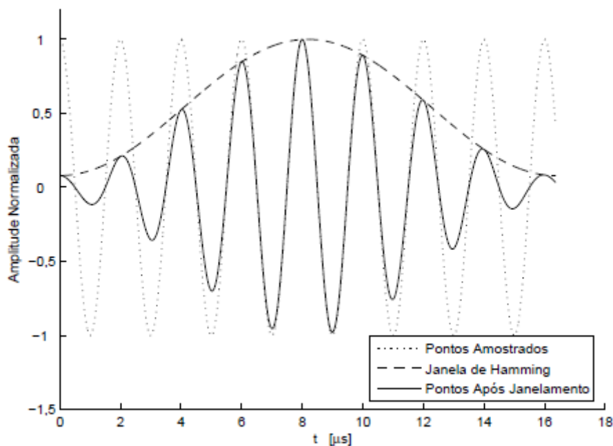
Figura B.2 – Exemplo de Janelamento de Pontos Pela Funcao de Hamming
