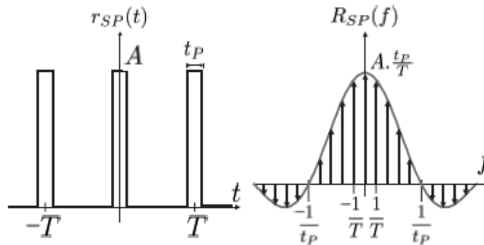
Figura 2.18 – Envoltório e respectivo espectro de um ruído impulsivo periódico.
