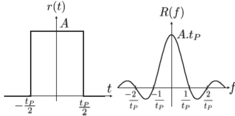
Figura 2.16 – Envoltório do ruído impulsivo periódico e seu espectro associado.
