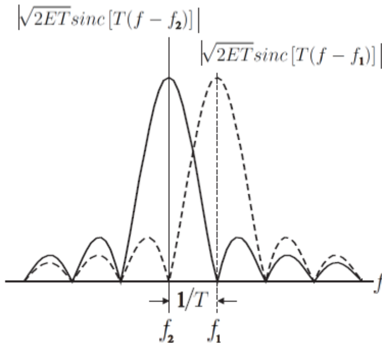
Figura 2.24 – Magnitude Espectral de cada símbolo BFSK
