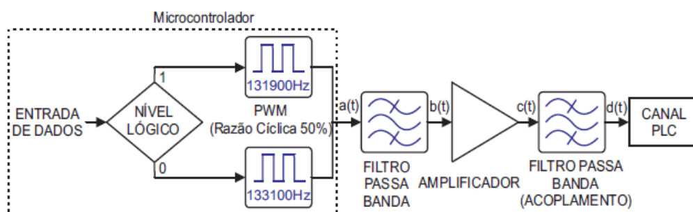
Figura 5.1 – Diagrama de blocos do transmissor KNX proposto.
