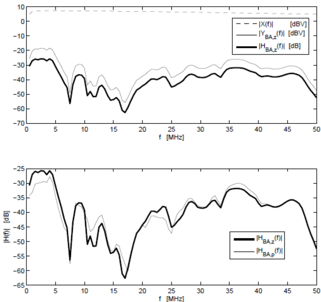
Figura 3.19 – Obtencao da funcao de transferencia de magnitude no percurso BA em a) e comparacao entre as funcoes obtidas na passagem por zero e no pico de tensao da rede eletrica em b).
