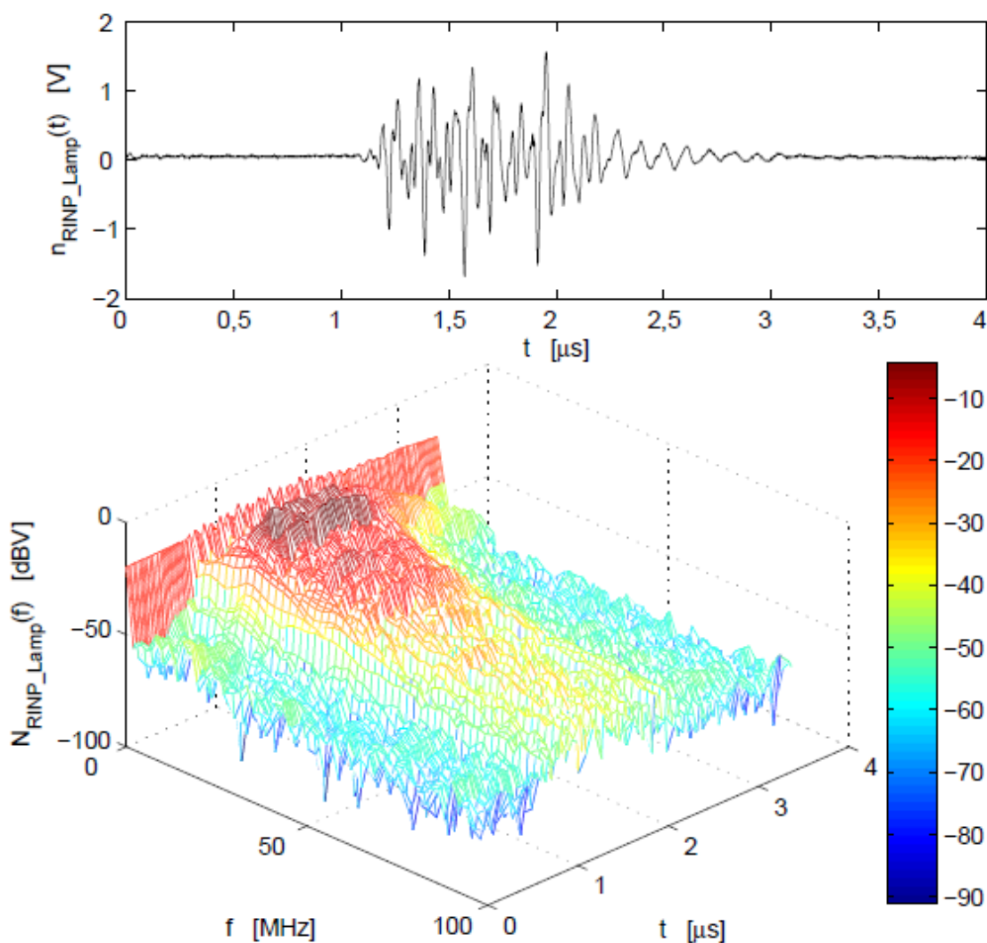
Figura 4.6 – Comportamento impulsivo e espectral do RINP gerado pelo desligamento de um reator de lampada fluorescente de 40W.
