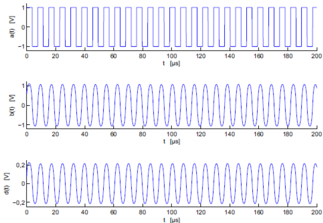
Figura 5.8 – Sinais gerados por simulação relativos a modulação de parte de um símbolo a ser transmitido.
