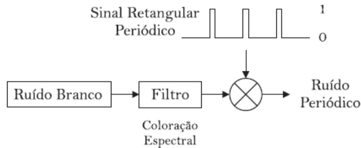
Figura 2.14 – Modelagem do ruído impulsivo periódico.
