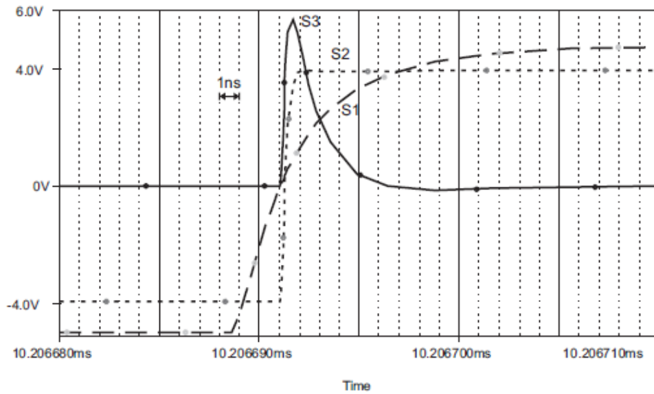
Figura 3.2 – Resultados da simulação PSPICER de um pulso do gerador
