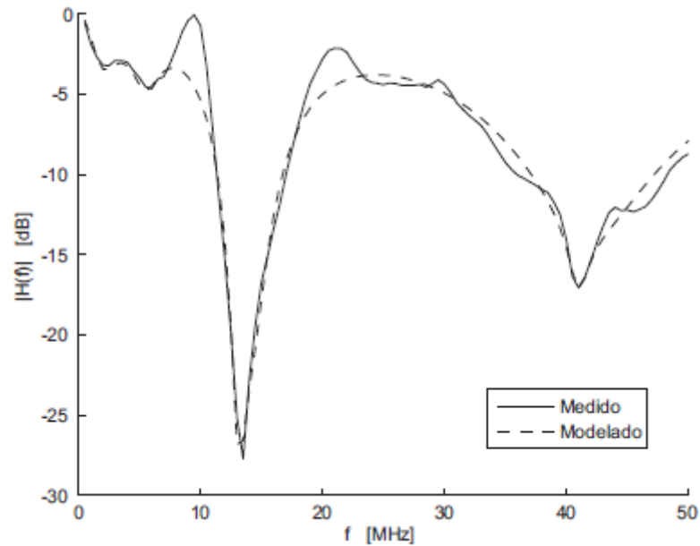
Figura 3.10 – Resposta em magnitude da medicao e do modelo por 6 BSRs.
