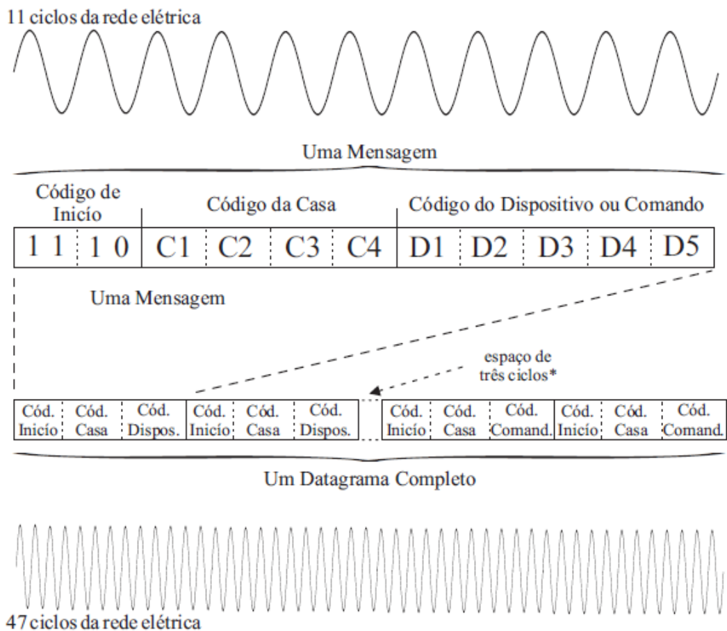
Figura 2.27 – Formato de um Datagrama Basico Completo do Protocolo X10
