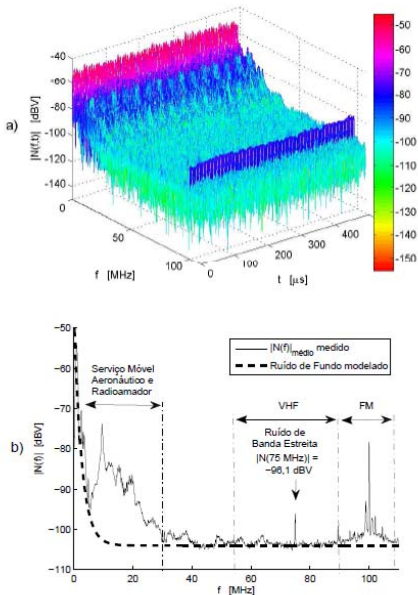
Figura 4.1 – Magnitude espectral do ruído capturado em uma TUG numa residencia. Ao longo do tempo em a), médio e ruído de fundo modelado em b).
