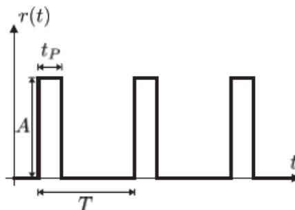
Figura 2.15 – Modelagem da envoltoria do ruído impulsivo periódico.
