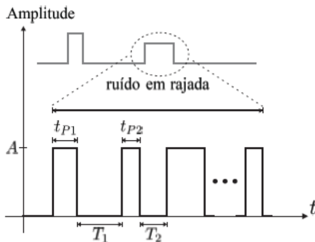
Figura 2.20 – Modelagem do Ruído em Rajada (RR).
