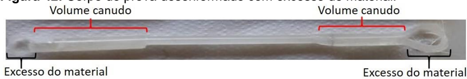
Figura 42: Corpo de prova desenformado com excesso de material.
