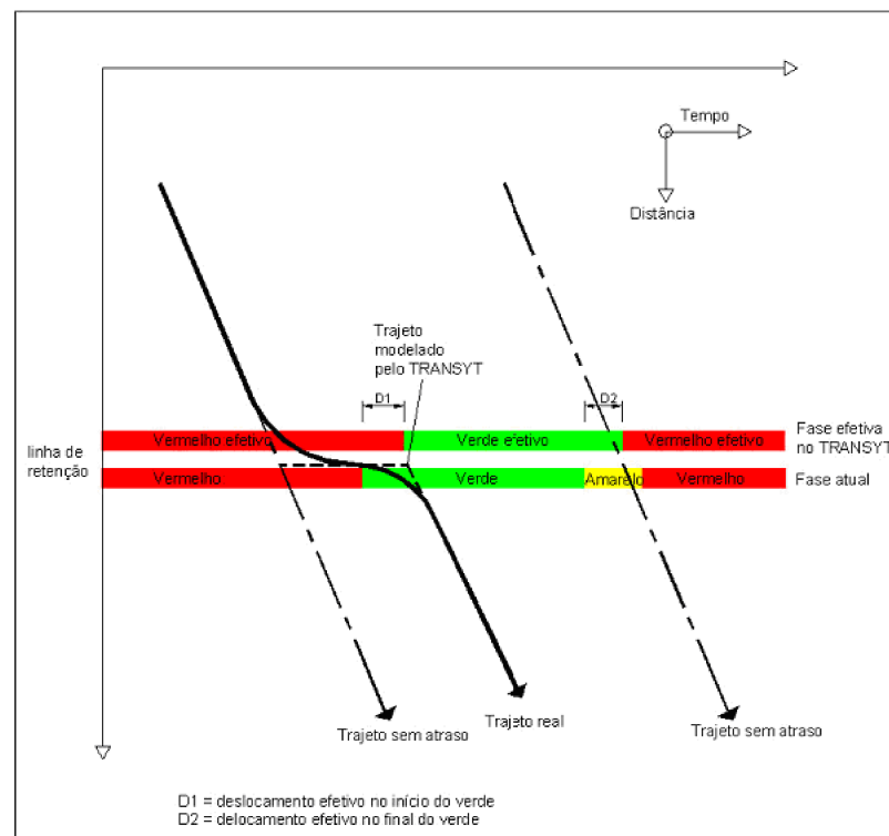
Figura 2.8 – Modelagem do comportamento do tráfego no TRANSYT
