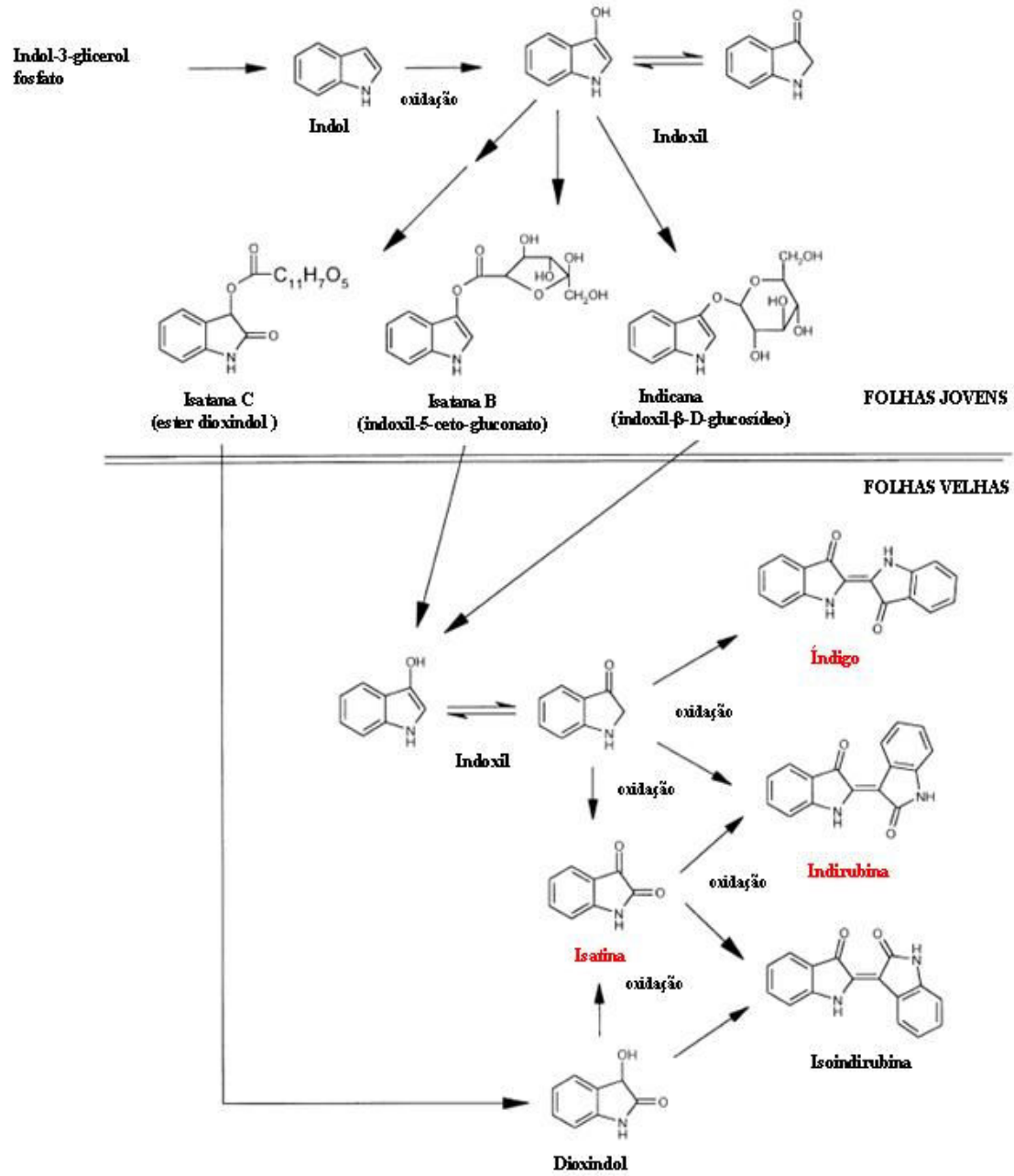
Figura 5 – Biosíntese dos pigmentos indigóides em plantas Fonte: Maugard et al. (2001)
