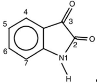
Figura 1 – Estrutura química da isatina (MATHEUS et al., 2007).
