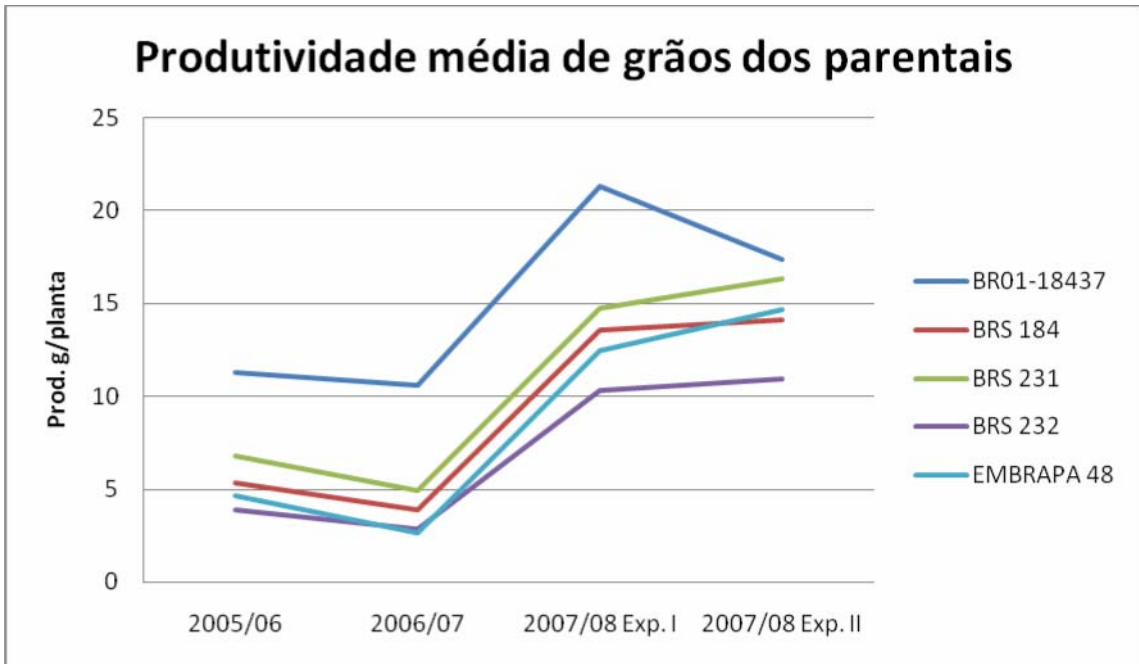
Figura 3.1 – Produtividade média de grãos dos parentais, experimentos não tratados com fungicidas, em Londrina, PR.
