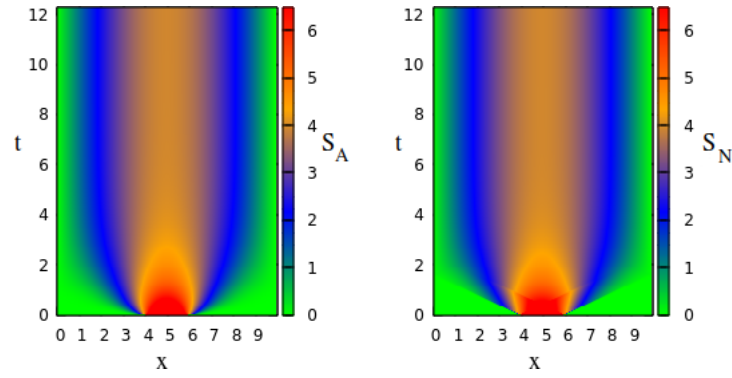
Figura 5.8: Soluções analítica ( S_A ) e numérica ( S_N ) para a densidade populacional em regime permanente para K_1 = 0.1 .
