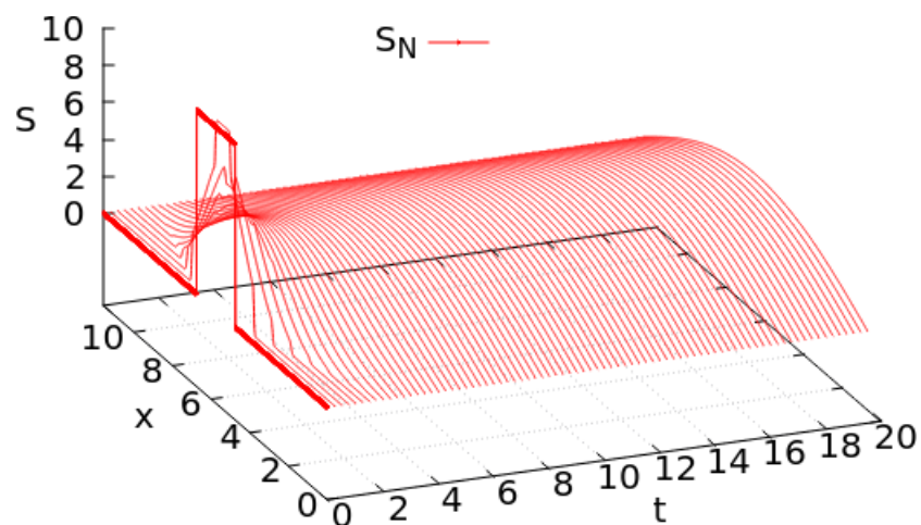
Figura 5.13: Solução numérica ( S_N ) para a densidade populacional em regime permanente com o modelo logístico.
