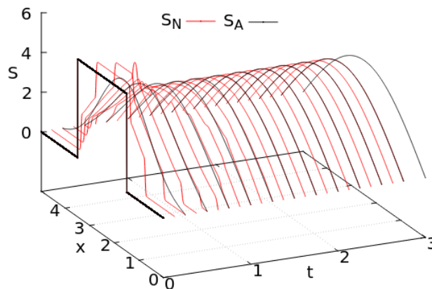
Figura 5.4: Soluções numérica ( S_N ) e analítica ( S_A ) para a densidade populacional em regime permanente, com o modelo exponencial.
