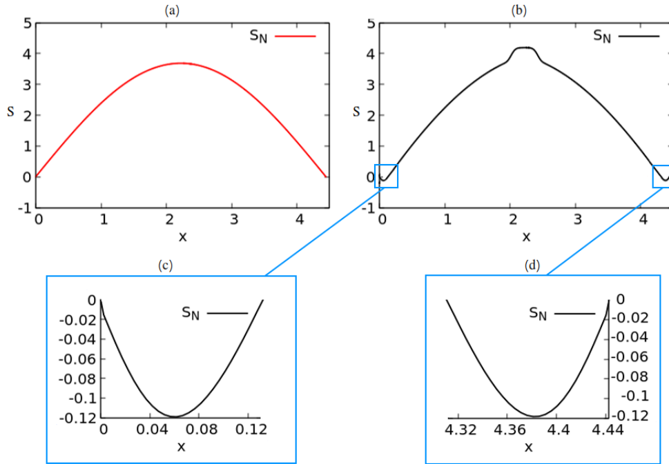
Figura 5.3: Solução numérica para a densidade populacional no instante t = 2.3 com ni = 900 , para \tau = \frac{1}{2\lambda} = 1.6 \times 10^{-1} (a) e \tau = 0.5 (b).
