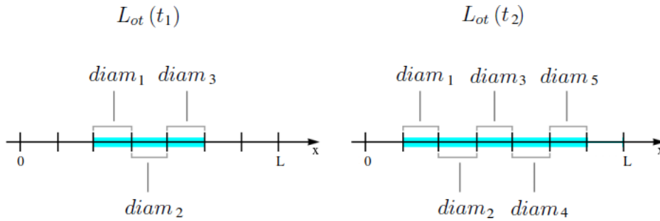
Figura 3.2: Ilustração de uma ocupação territorial em dois tempos subsequentes.
