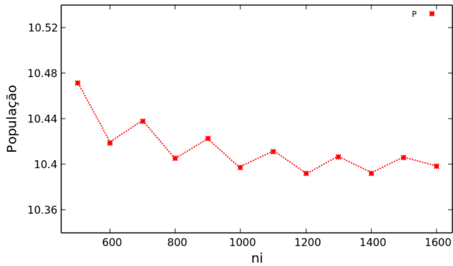
Figura 5.1: Refinamento da malha com a população em regime permanente, com o modelo exponencial.
