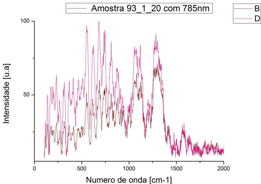
Figura 7.24 - Superposição de espectros Raman de duas cores; pontos “P2” e “P3” da amostra 93_1_20
