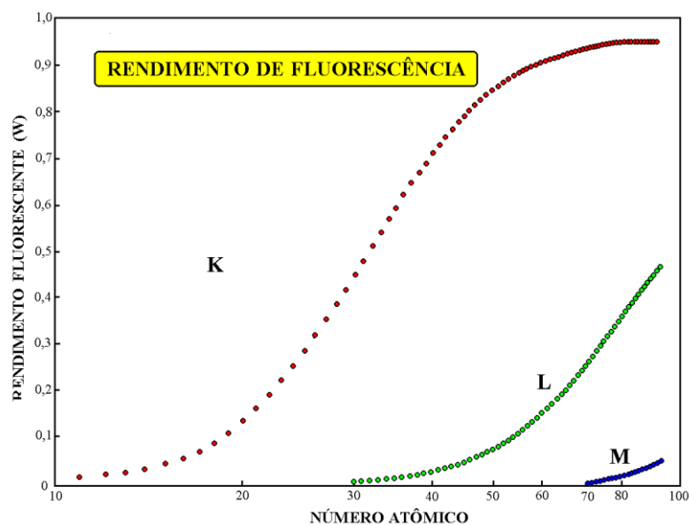
Figura 4.11 - Rendimento de fluorescência para a camada K, L, e M em função do número atômico dos elementos. (NASCIMENTO FILHO, 1999).
