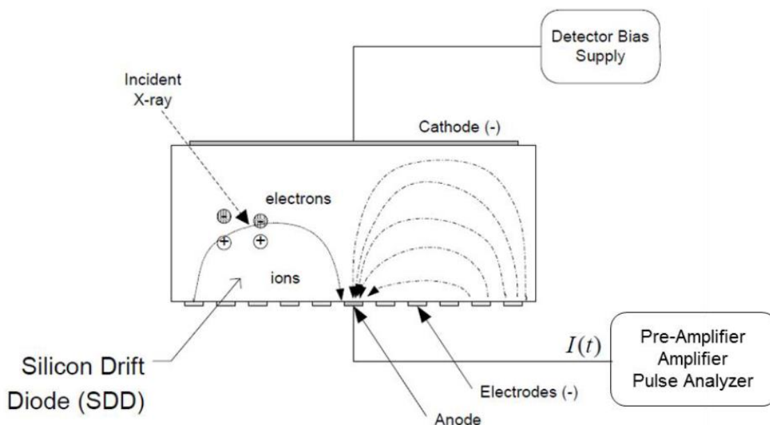
Figura 4.12 - Esquema ilustrando o funcionamento do detector de SDD (Otoni, 2015).
