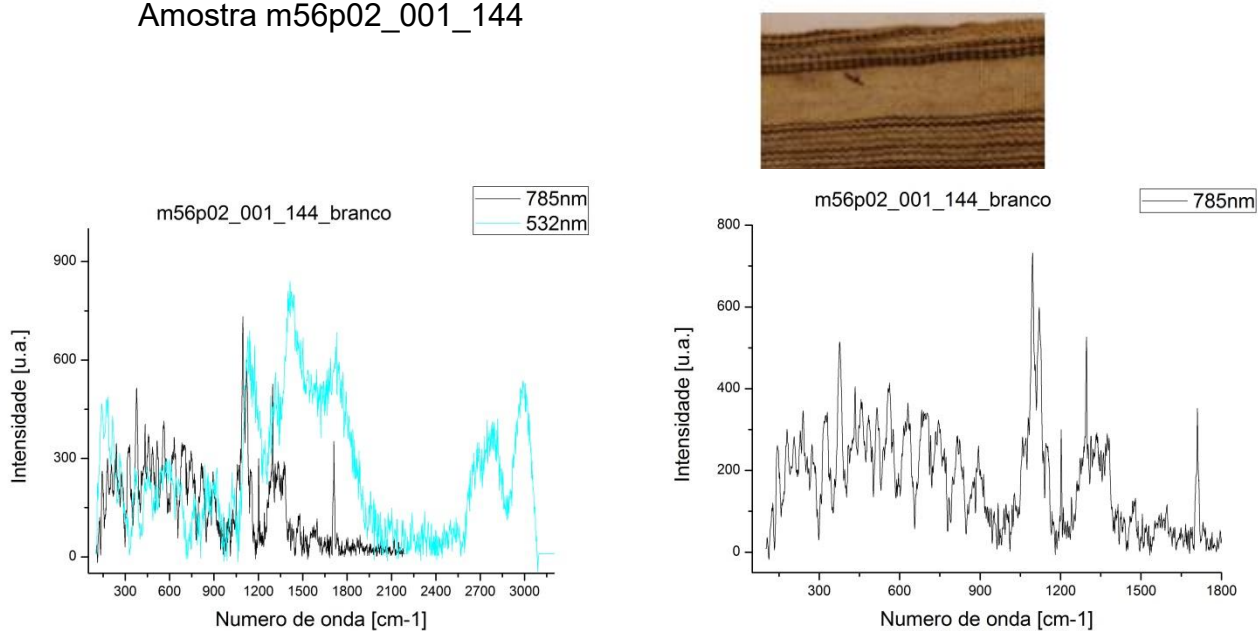
Figura 7.14 - Lado esquerdo, superposição de espectros Raman medidos na área branca com lasers de comprimento de onda 785nm e 532nm. Lado direito, zoom do espectro Raman da mesma área com laser 785nm.
