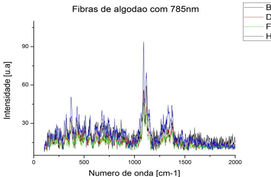
Figura 7.27 - Superposição de espectros Raman de fibras de algodão.
