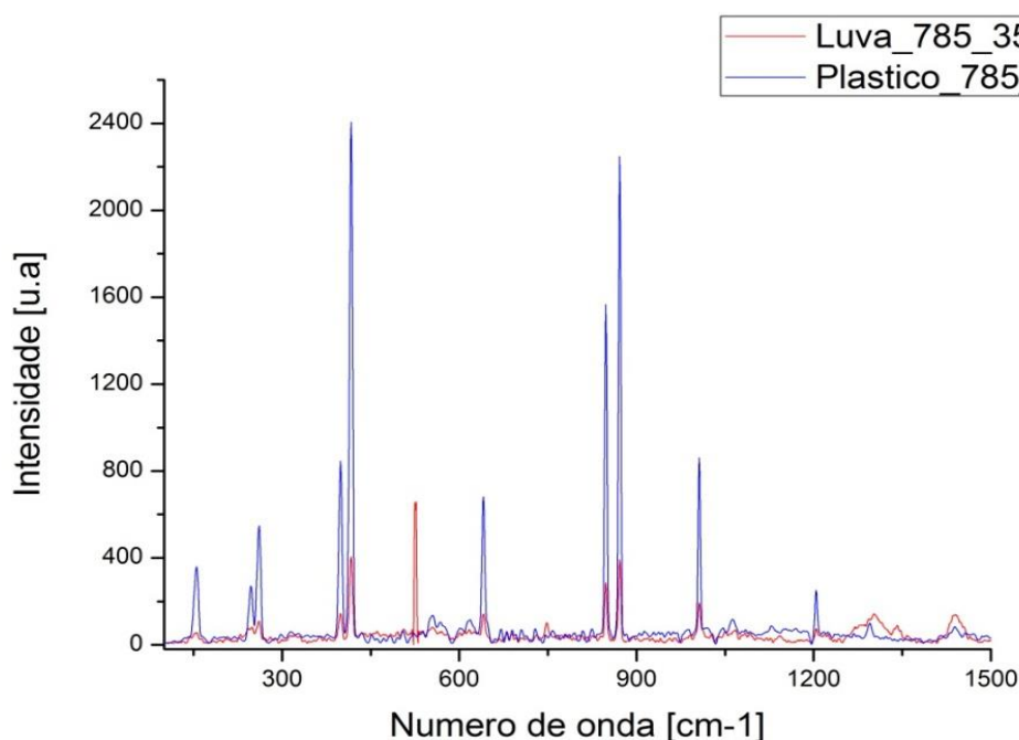
Figura 7.9 - Sobreposição de espectros Raman medido de materiais sintéticos luva (cor vermelha) e plástico (cor azul) com laser 785nm.
