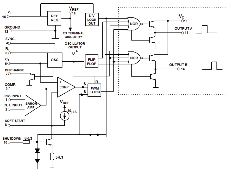
Figura 26 – Diagrama de blocos do CI3525.
