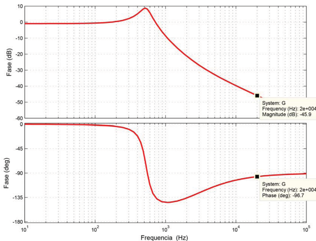
Figura 18 – Diagrama de Bode de Módulo e Fase de G_V(s) .
