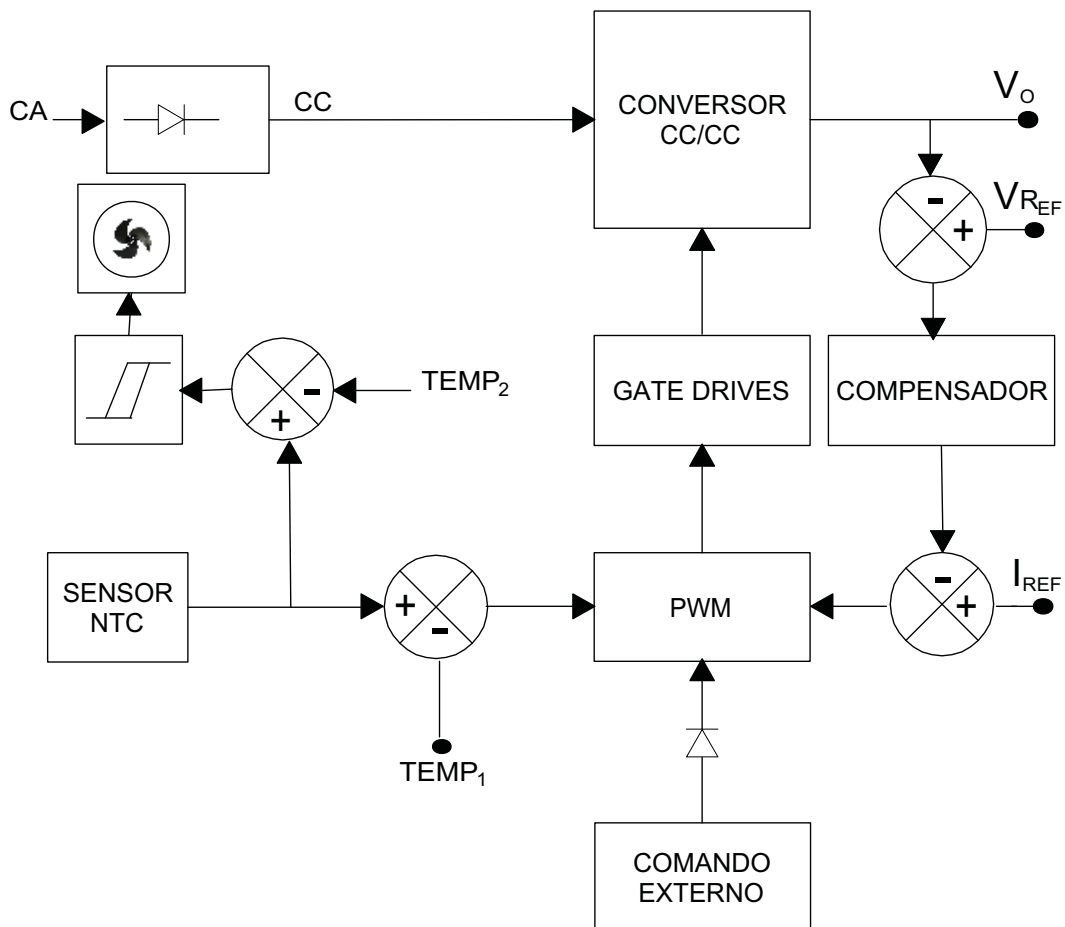
Figura 32 – Diagrama de blocos do controle de temperatura.
