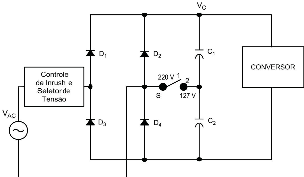
Figura 68 – Módulo retificador.
