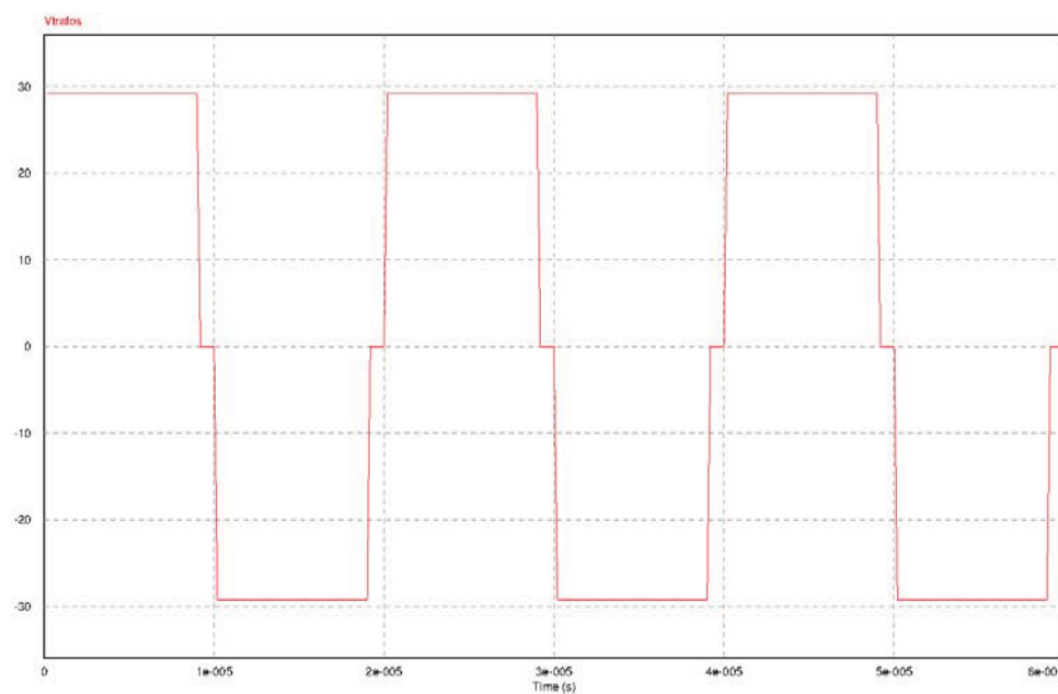
Figura 40 – Forma de onda da tensão de saída dos dois transformadores em série na simulação do conversor em malha aberta.
