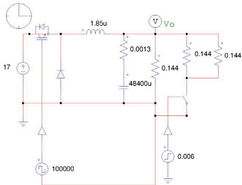
Figura 47 – Esquema utilizado na simulação do conversor buck equivalente em malha aberta para um degrau de corrente de saída.
