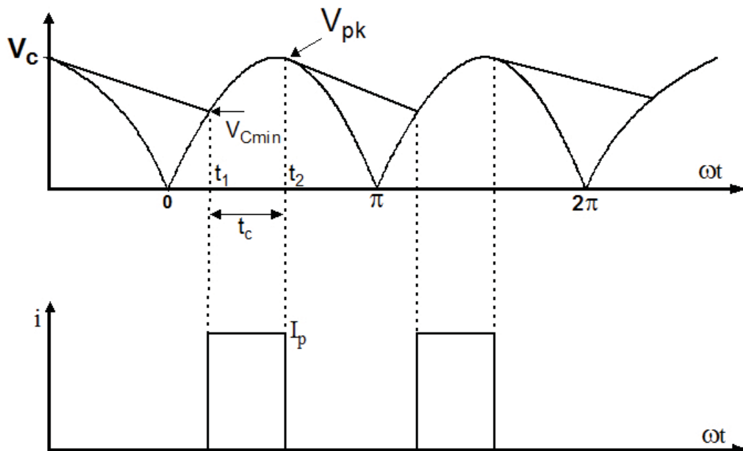
Figura 71 – Tensão e Corrente nos Capacitores C_1 e C_2 em série (C).
