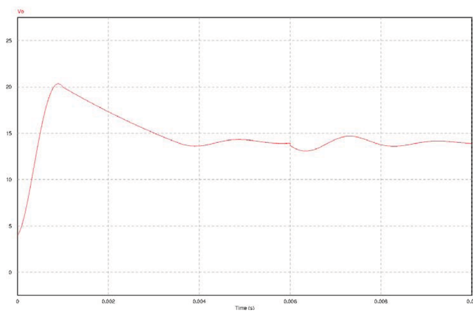
Figura 44 – Forma de onda da tensão de saída para um degrau de corrente do conversor CC/CC com dobrador de corrente na simulação em malha aberta.
