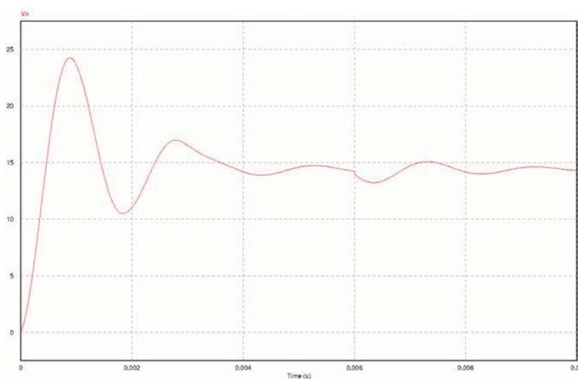
Figura 48 – Forma de onda da tensão de saída para um degrau de corrente do conversor buck equivalente na simulação em malha aberta.
