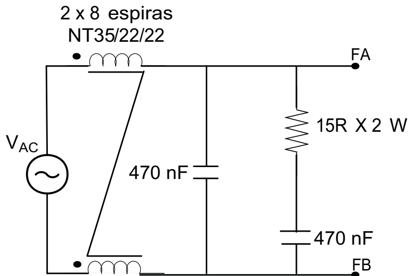
Figura 80 – Filtro RFI.
