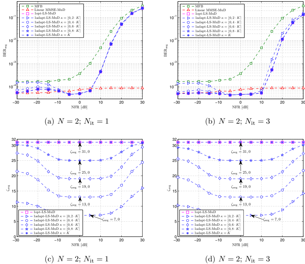
Figura 5.10: Robustez ao efeito perto-longe dado por NFR^{(II)} dos detectores 1opt-LS-MuD e 1adapt-LS-MuD; algoritmos de busca com N_{it} = 1 iteração em (a) e com N_{it} = 3 iterações em (b); respectivas quantidades médias de cálculos da função custo em (c) e (d); K = 30 usuários; seqüências de Gold e L = 31 ; sistema SIMO com N = 2 antenas; canal com desvanecimento Rayleigh plano e SNR = 18 dB.
