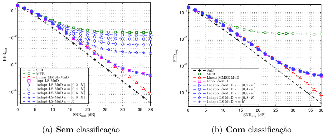
Figura 5.7: Desempenho do detector 1adapt-LS-MuD sem classificação dos sinais em (a) e com classificação dos sinais em ordem crescente de amplitude em (b); sistema SISO; canal com desvanecimento Rayleigh plano e efeito NFR (1) ; K = 30 usuários; sequências de Gold e L = 31 ; algoritmos LS com N_{it} = 3 iterações.
