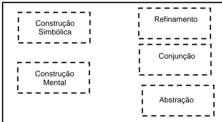
Figura 8 – Pensamento Matemático-Computacional
