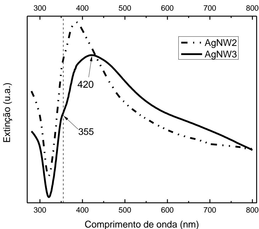
Figura 36: Desvio para o vermelho no pico correspondente ao modo transversal da SPR como resultado de um maior tempo de aquecimento durante a síntese AgNW3.
