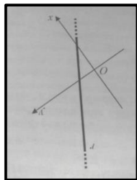
Figura 02: Representação Gráfica da reta r
