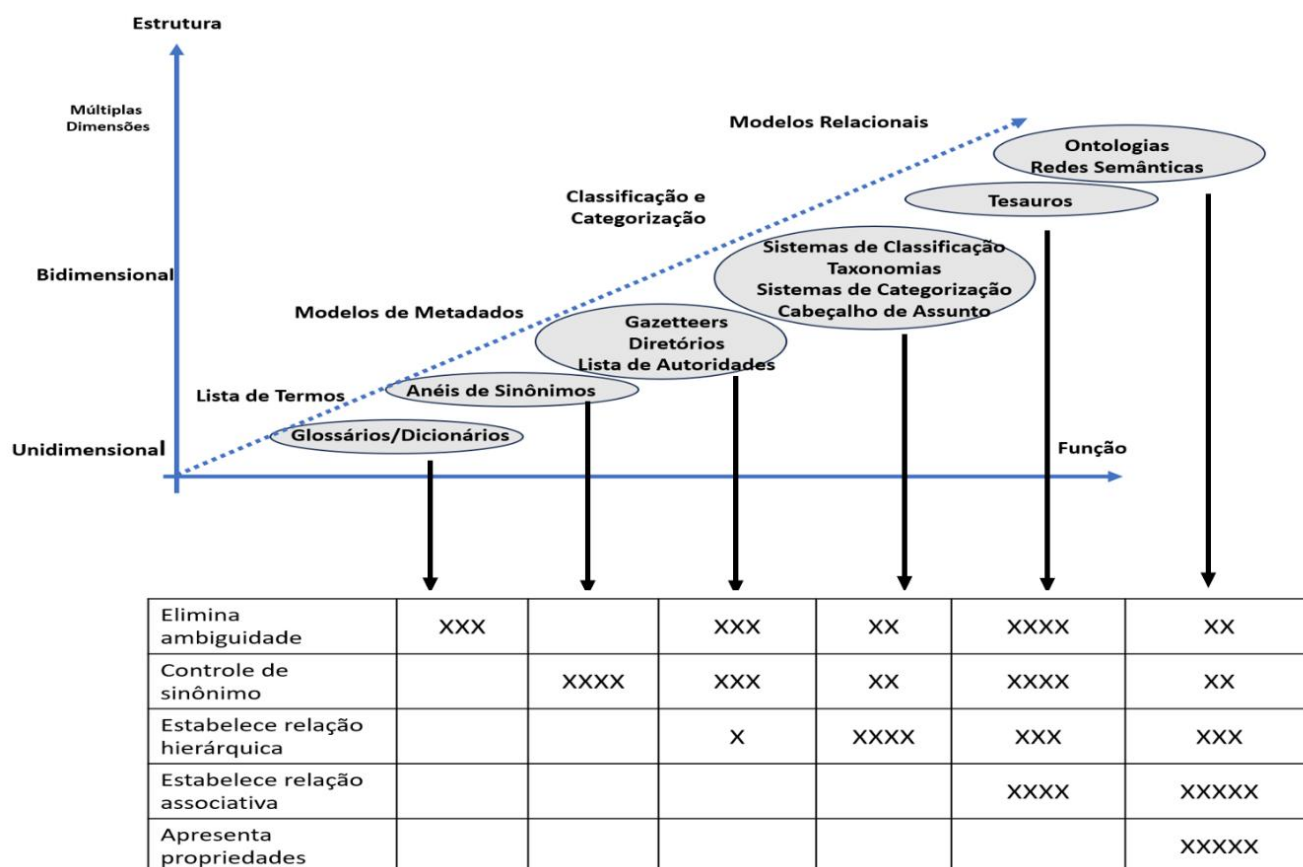
Figura 7 - Uma visão geral das estruturas e funções dos SOC
