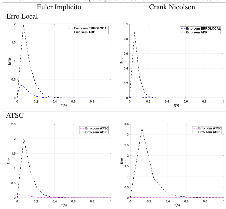
Figura 4.9: Comparação entre os erros das soluções, com adaptação e passo constante, com o mesmo número de iterações para lei de resfriamento de Newton.
