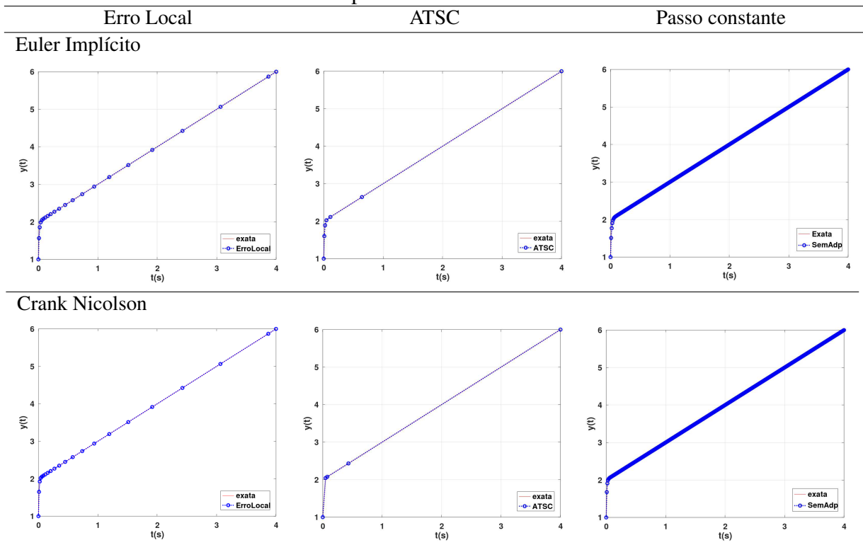
Figura 4.2: Soluções exata e numéricas dos métodos com adaptação e passo constante para problema de Gear
