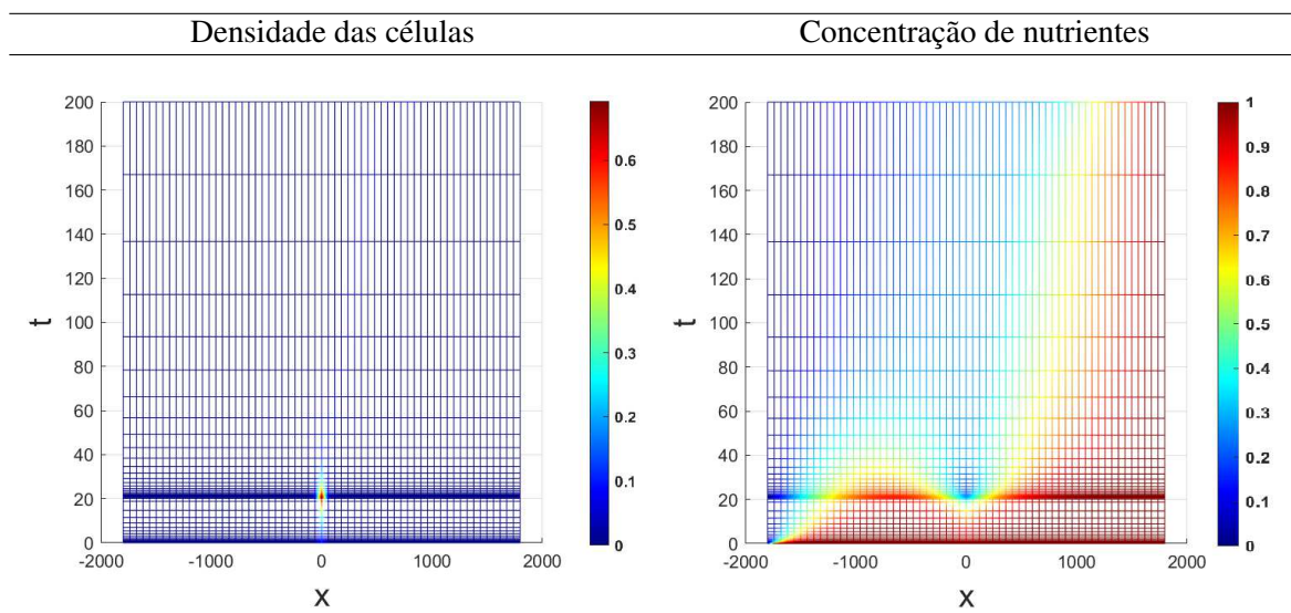
Figura 6.7: Malha gerada usando o método de Crank Nicolson com adaptação
