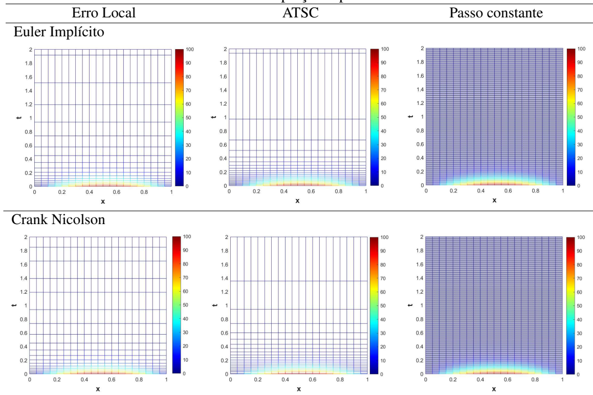
Figura 4.13: Comparação da malha entre a solução exata e numérica, para os métodos numéricos com adaptação e passo constante.
