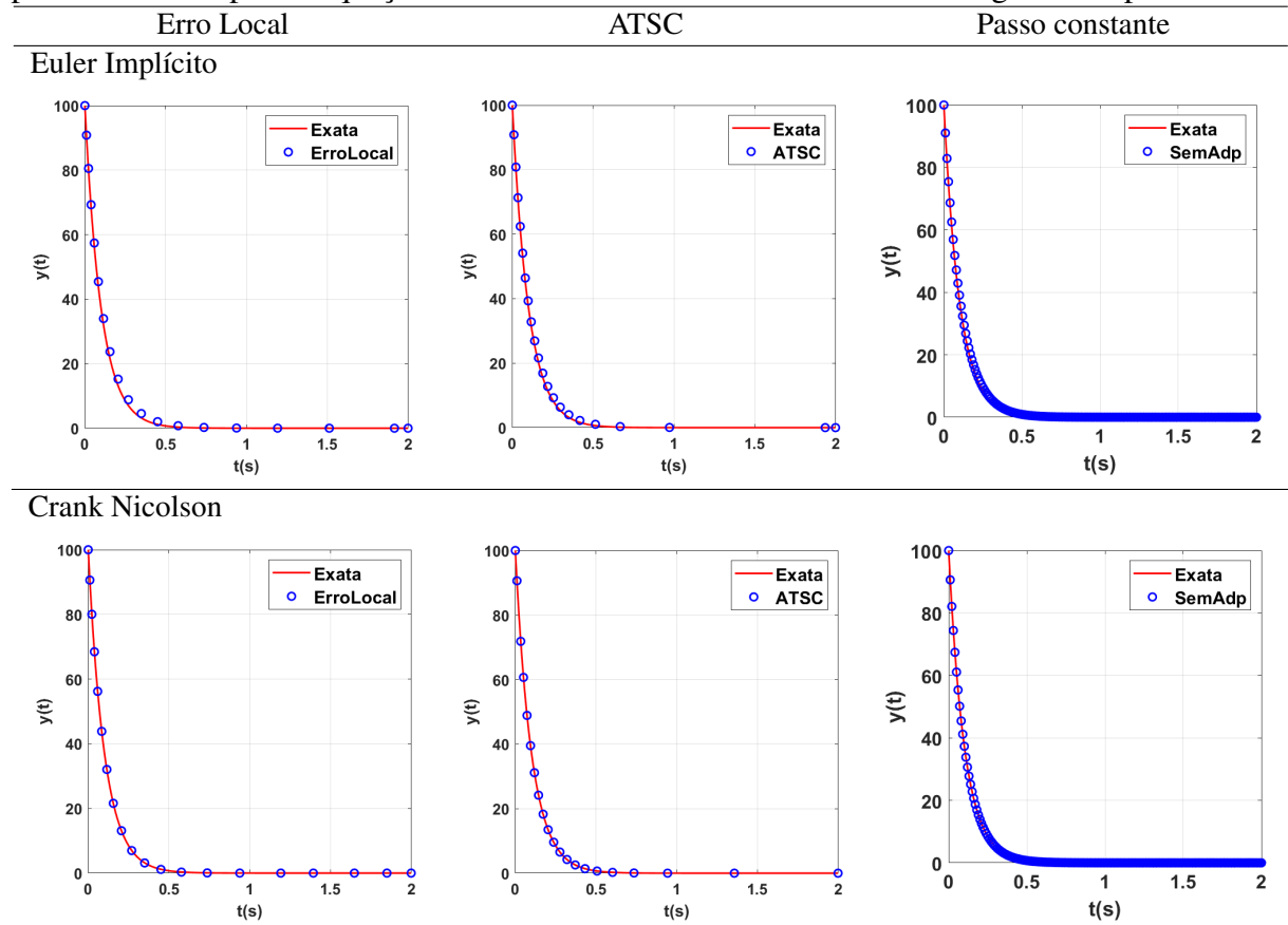
Figura 4.12: Comparação entre a solução exata e numérica, para os métodos com adaptação e passo constante para a equação da difusão do calor unidimensional em regime não permanente.
