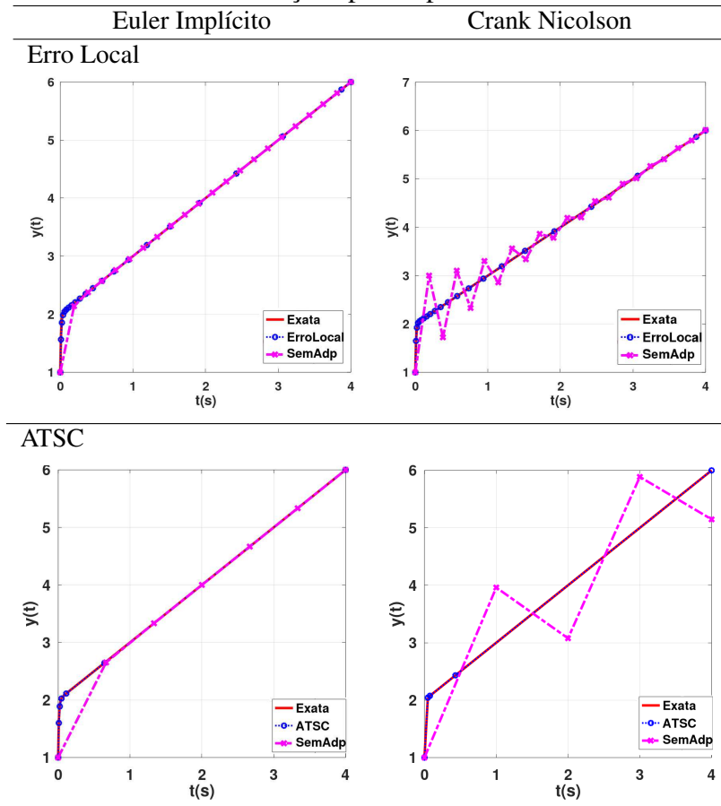
Figura 4.5: Soluções exata e numéricas dos métodos com adaptação e passo constante: mesmo número de iterações para o problema de Gear
