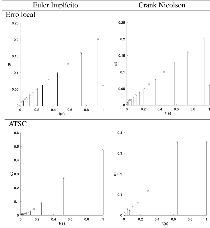
Figura 4.8: Histórico de passos no tempo para as técnicas adaptativas de tempo.
