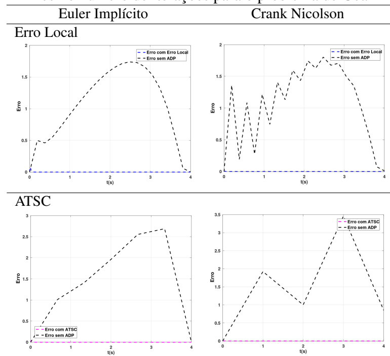
Figura 4.4: Comparação entre os erros das soluções, com adaptação e passo constante, com o mesmo número de iterações para o problema de Gear
