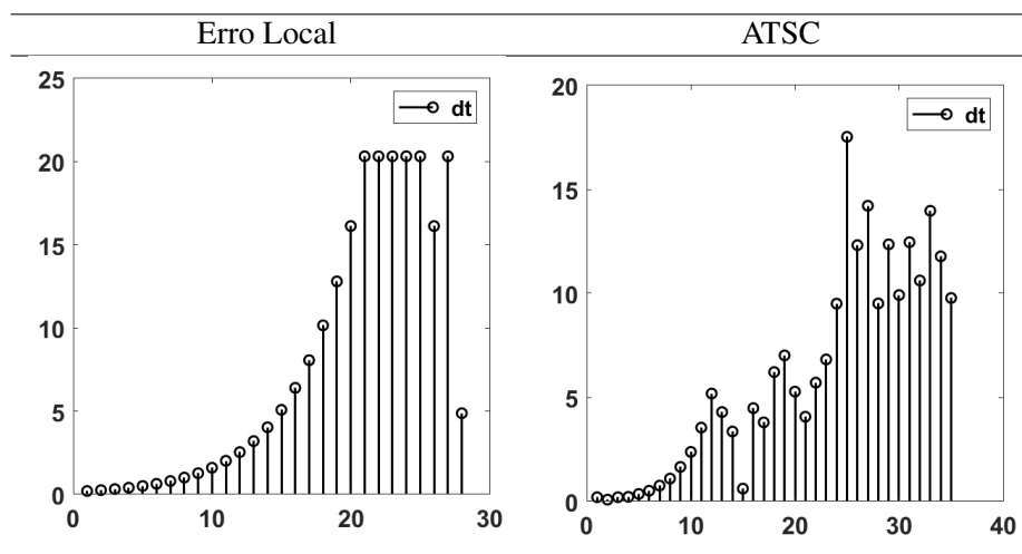
Figura 6.4: Histórico de passos no tempo
