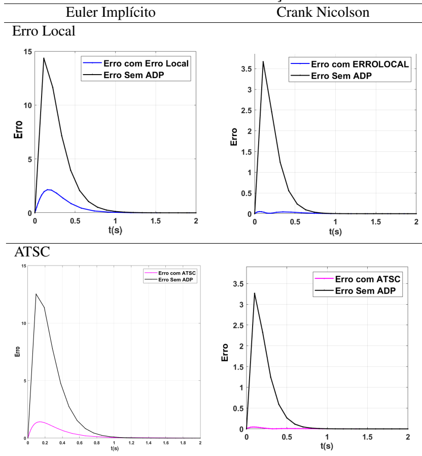
Figura 4.15: Comparação entre os erros das soluções, com adaptação e passo constante, com o mesmo número de iterações.
