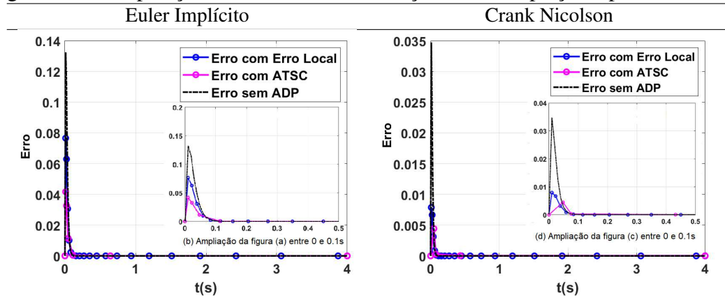
Figura 4.1: Comparação entre os erros das soluções com adaptação e passo constante
