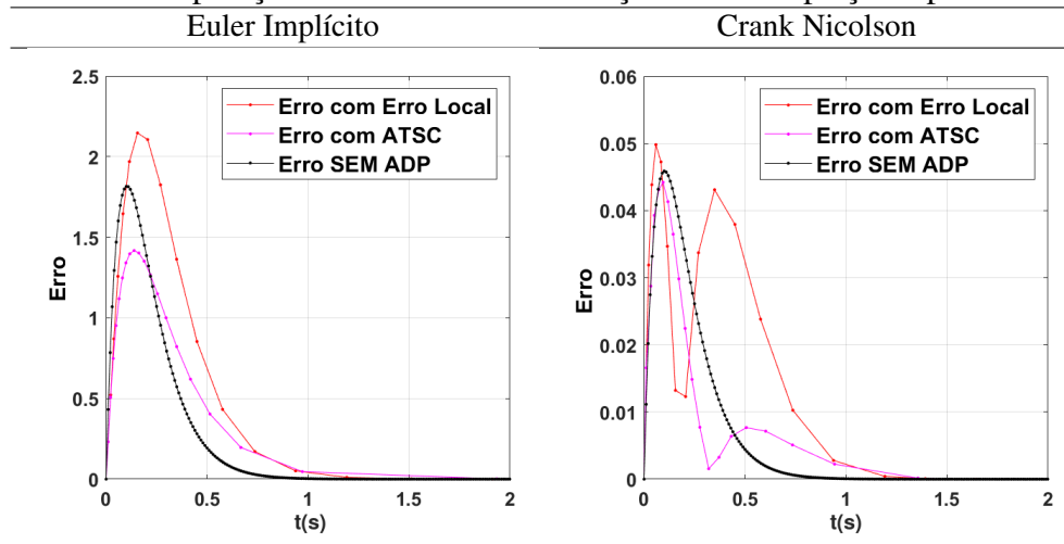
Figura 4.11: Comparação entre os erros das soluções com adaptação e passo constante
