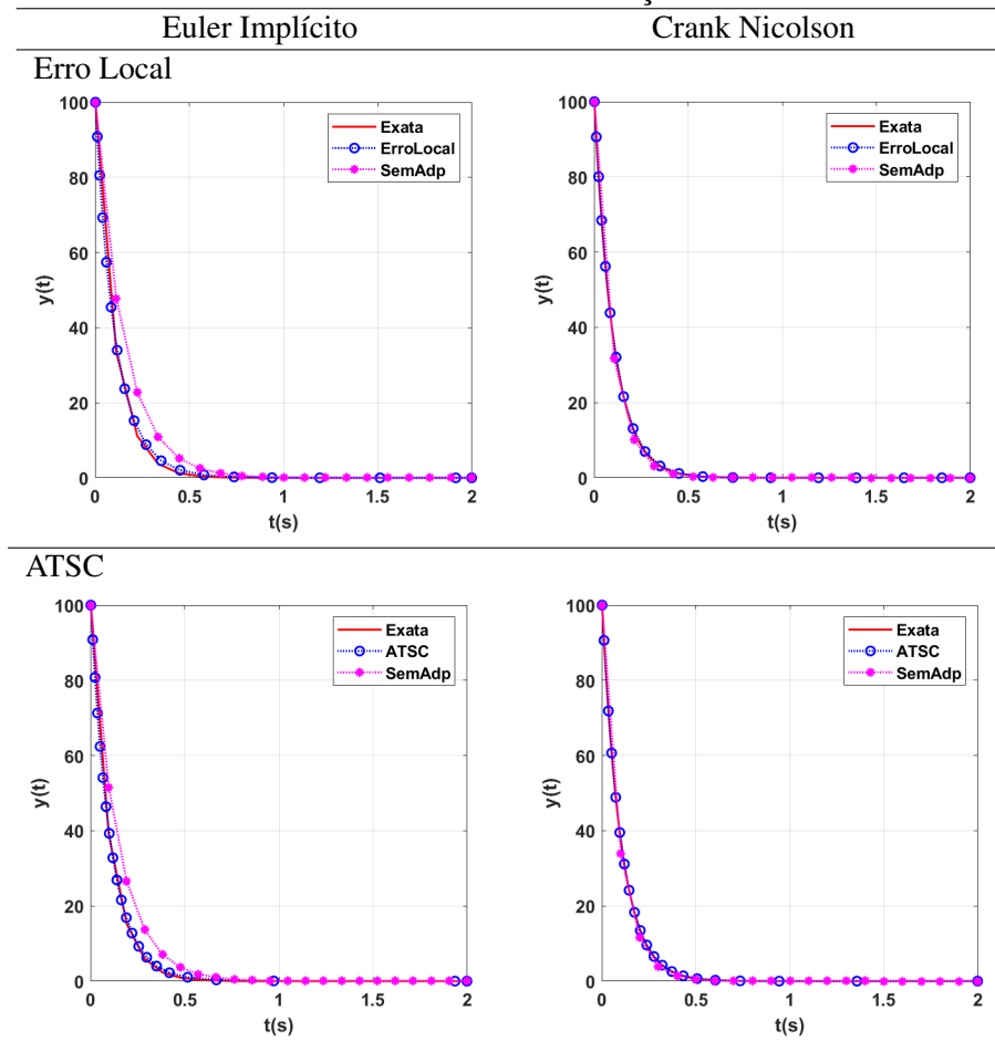
Figura 4.16: Soluções exata e numéricas dos métodos com adaptação e passo constante: mesmo número de iterações.
