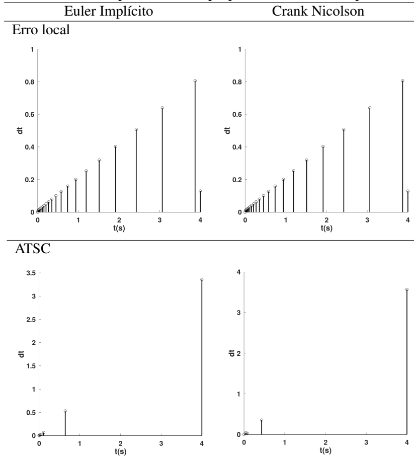
Figura 4.3: Histórico de passos no tempo para as técnicas adaptativas de tempo
