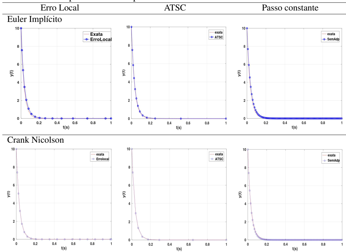
Figura 4.7: Comparação entre a solução exata e numérica, para os métodos com adaptação e passo constante para a lei de resfriamento de Newton.
