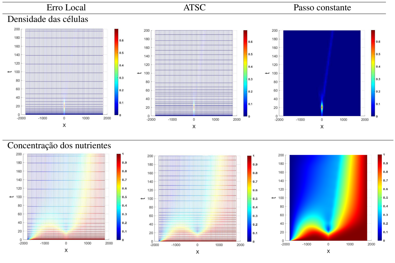
Figura 6.3: Comparação entre as malhas das soluções com adaptação e passo constante
