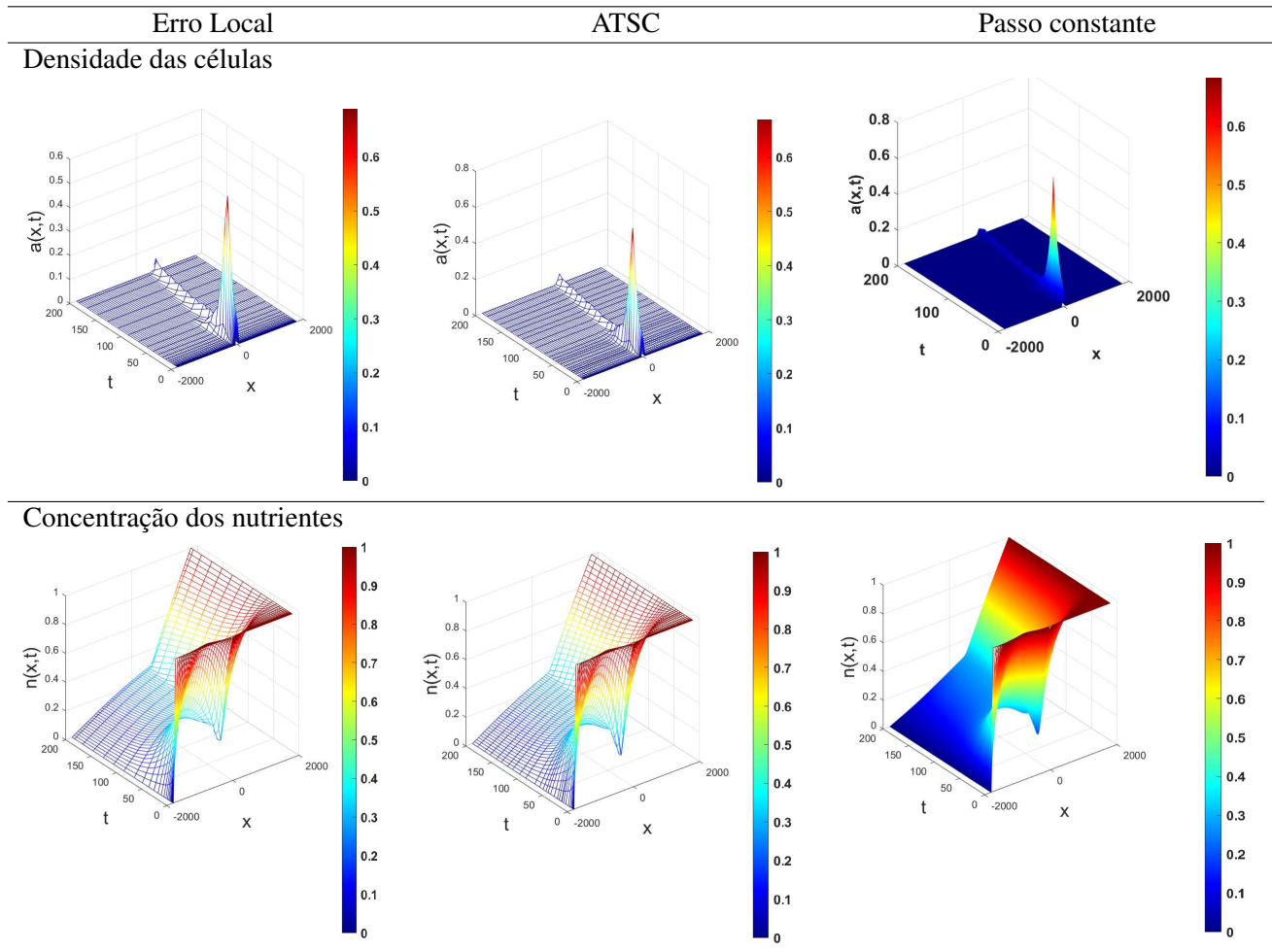
Figura 6.1: Comparação entre as soluções com adaptação e passo constante
