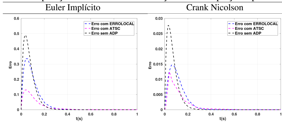
Figura 4.6: Comparação entre os erros das soluções com adaptação e passo constante
