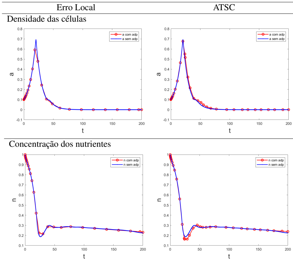
Figura 6.2: Comparação das soluções com adaptação e passo constante, corte em x=0
