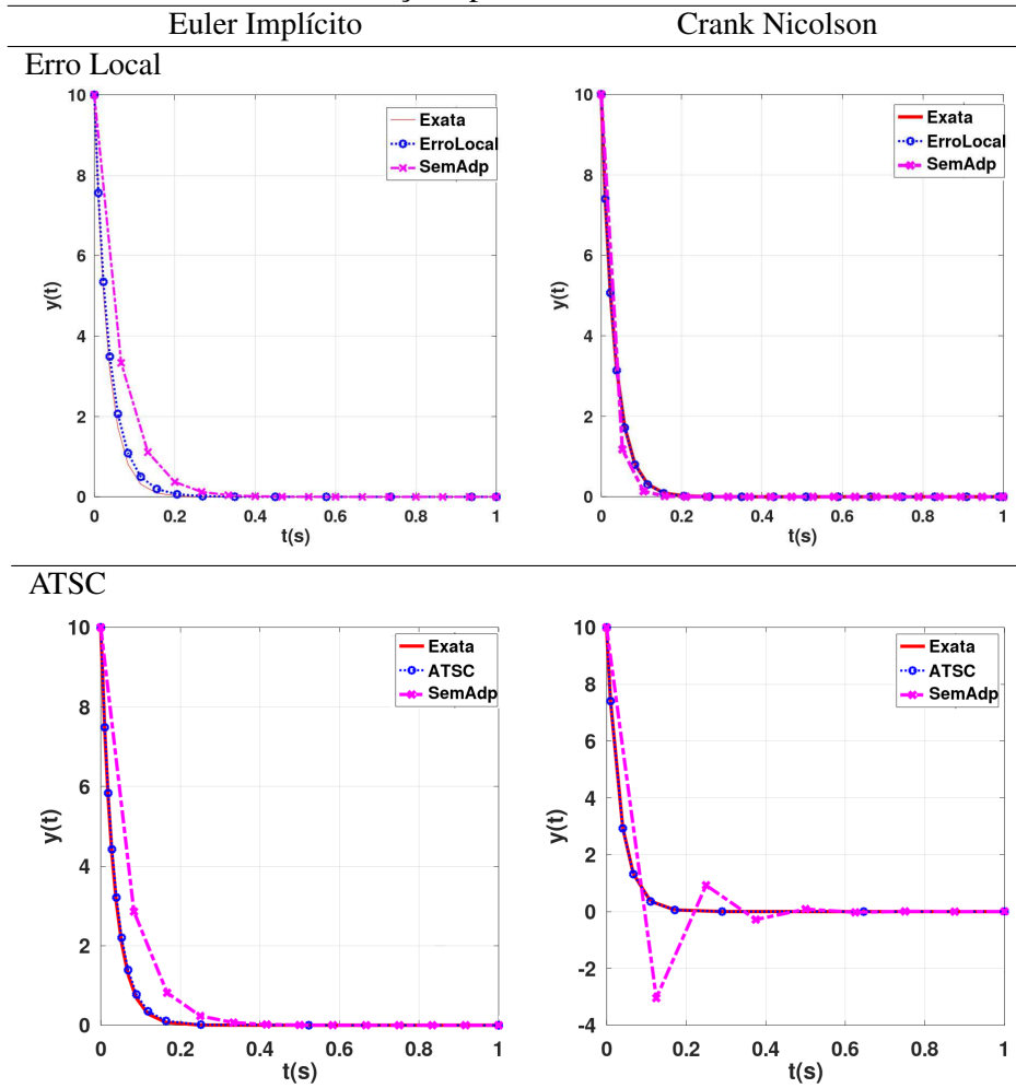
Figura 4.10: Soluções exata e numéricas dos métodos com adaptação e passo constante: mesmo número de iterações para lei de resfriamento de Newton.
