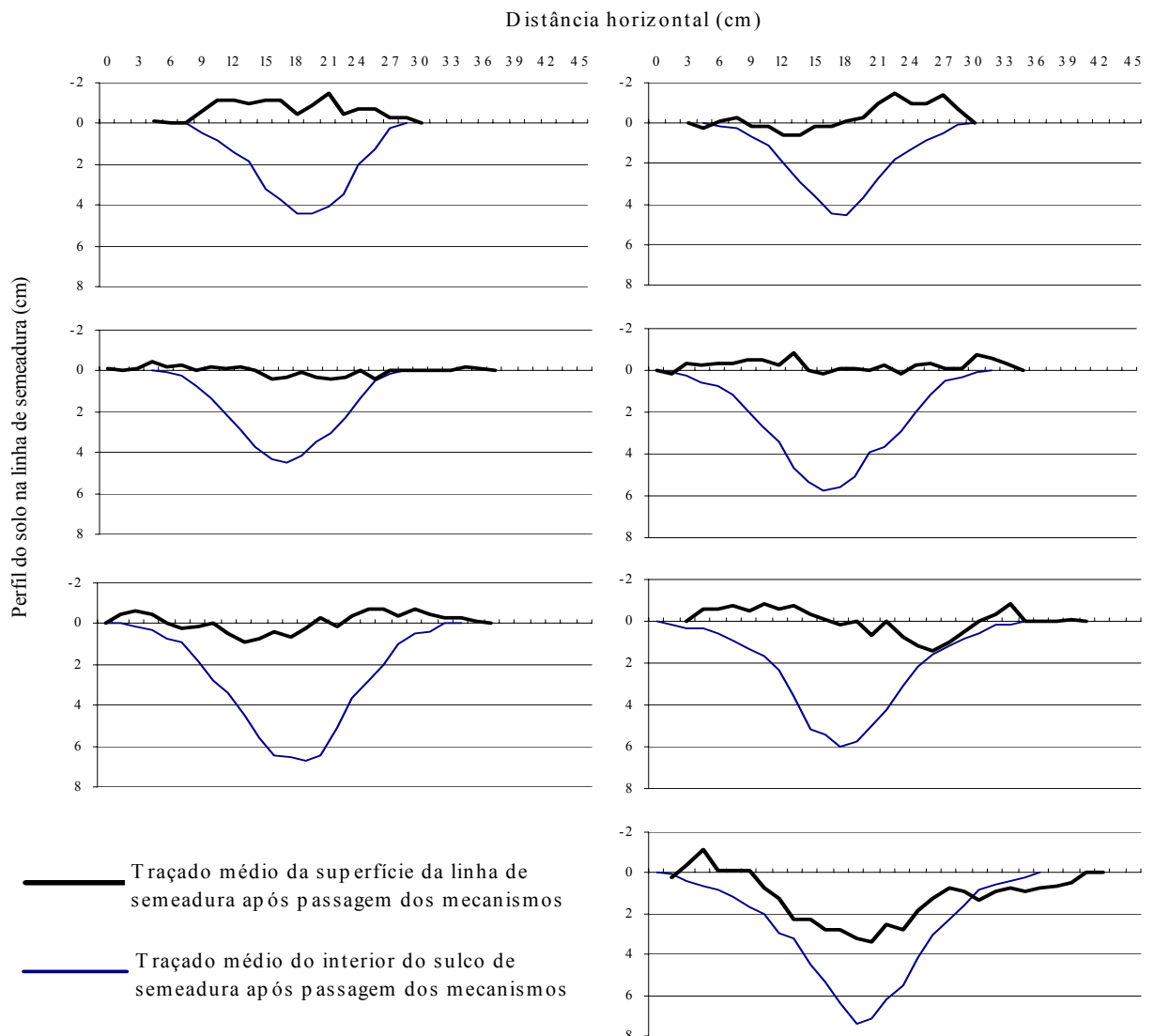
Figura 03 – Traçado médio da superfície da linha de semeadura após a passagem dos mecanismos e traçado médio do interior do sulco de semeadura após a passagem dos mecanismos de manejo da linha.
