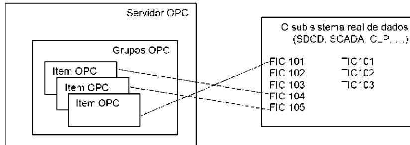
Figura 22 – Mapeamento de Itens OPC
