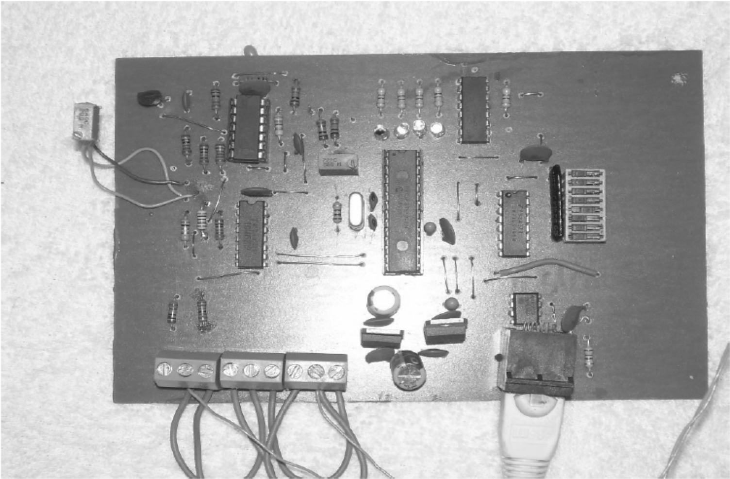
Figura 57 – Fotografia da segunda versão do terminal de rede implementado em PIC 16F876 para validação do sistema
