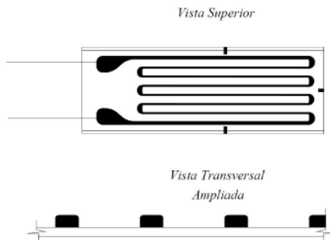
Figura 5 – Extensômetro elétrico laminar ( foil gauges )
