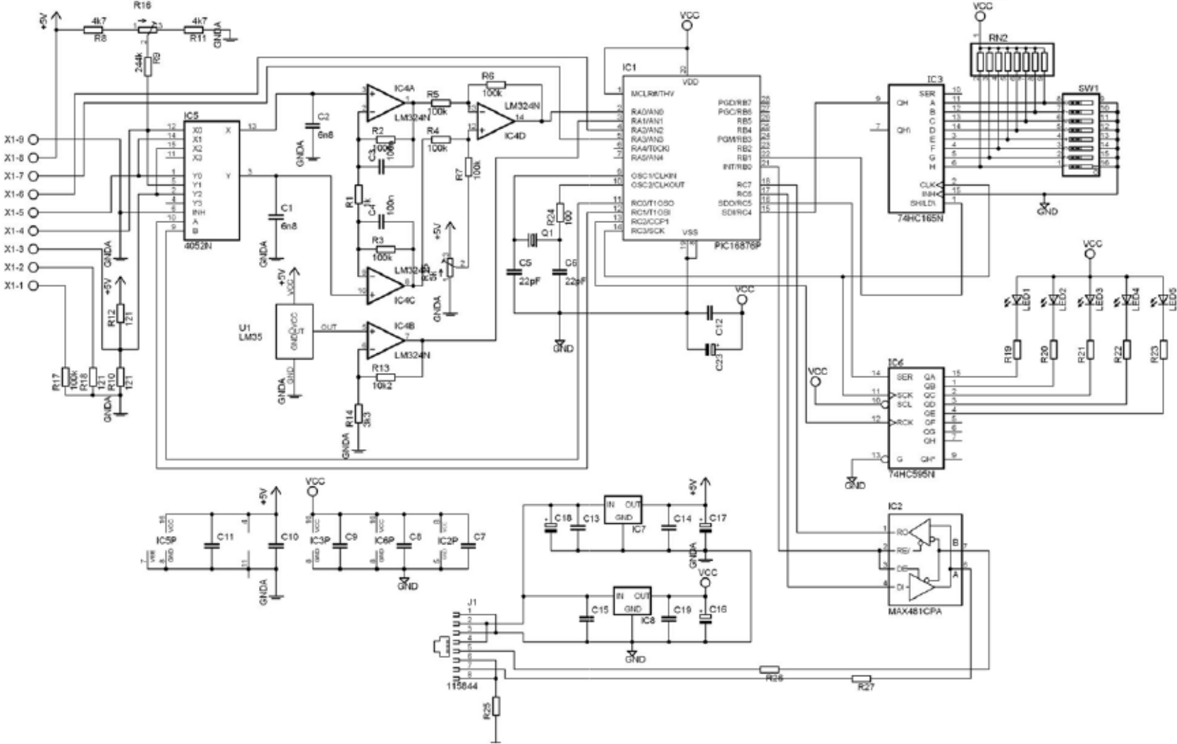
Figura 104 – Diagrama Esquemático Completo do Nó de Rede
