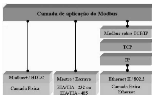
Figura 45 – Localização do protocolo MODBUS em correspondência ao modelo OSI/ISO.
