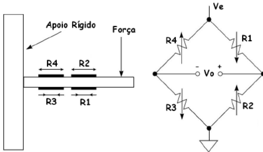
Figura 12 – Configuração utilizando 4 extensômetros ativos ( full bridge )
