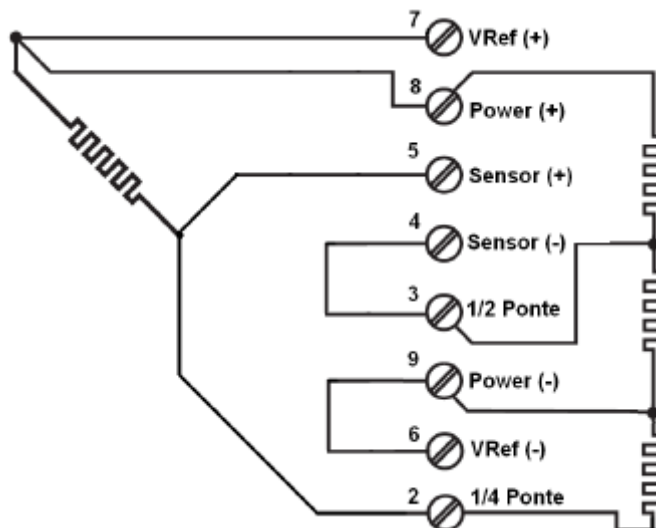
Figura 31 – Diagrama de ligação de 1/4 de ponte.
