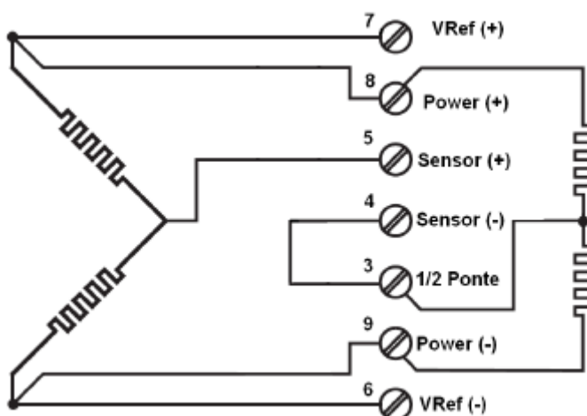
Figura 32 – Diagrama para ligação dos extensômetros em 1/2 ponte
