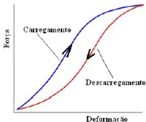
Figura 99 – Curva de histerese para materiais elásticos
