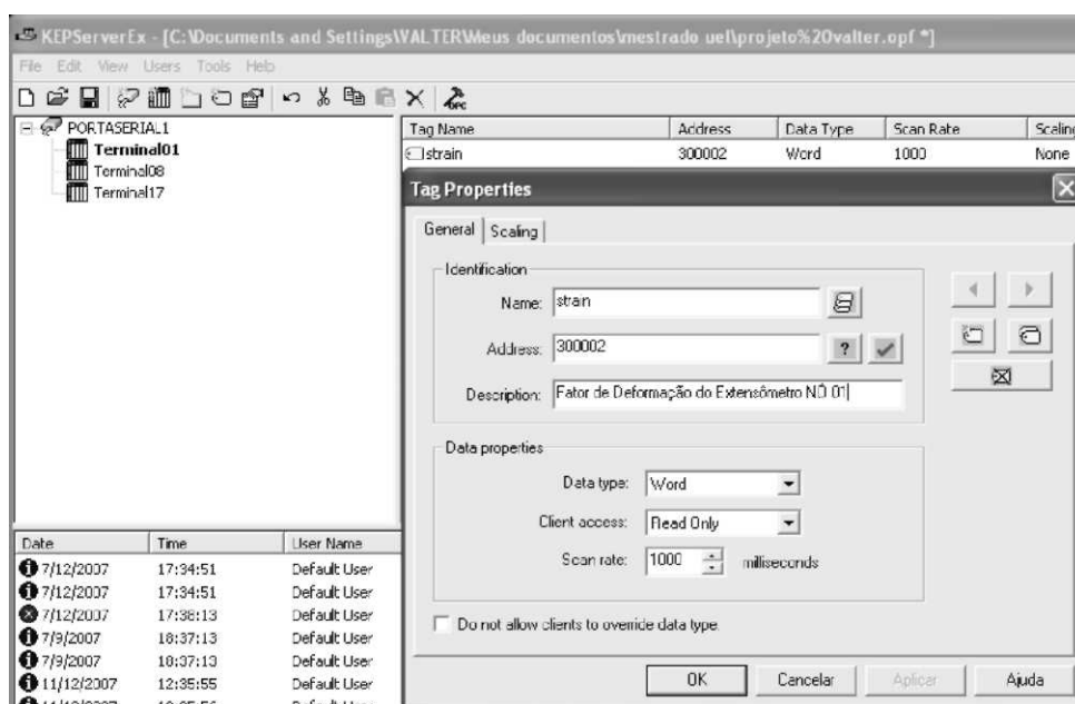
Figura 74 – Criação de uma nova tag no software Kepware Server Modbus
