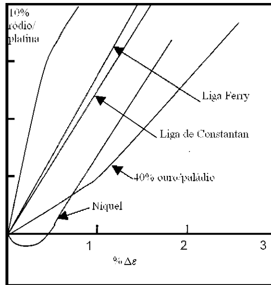
Figura 10 – Curva dos fatores de sensibilidade de diversos materiais
