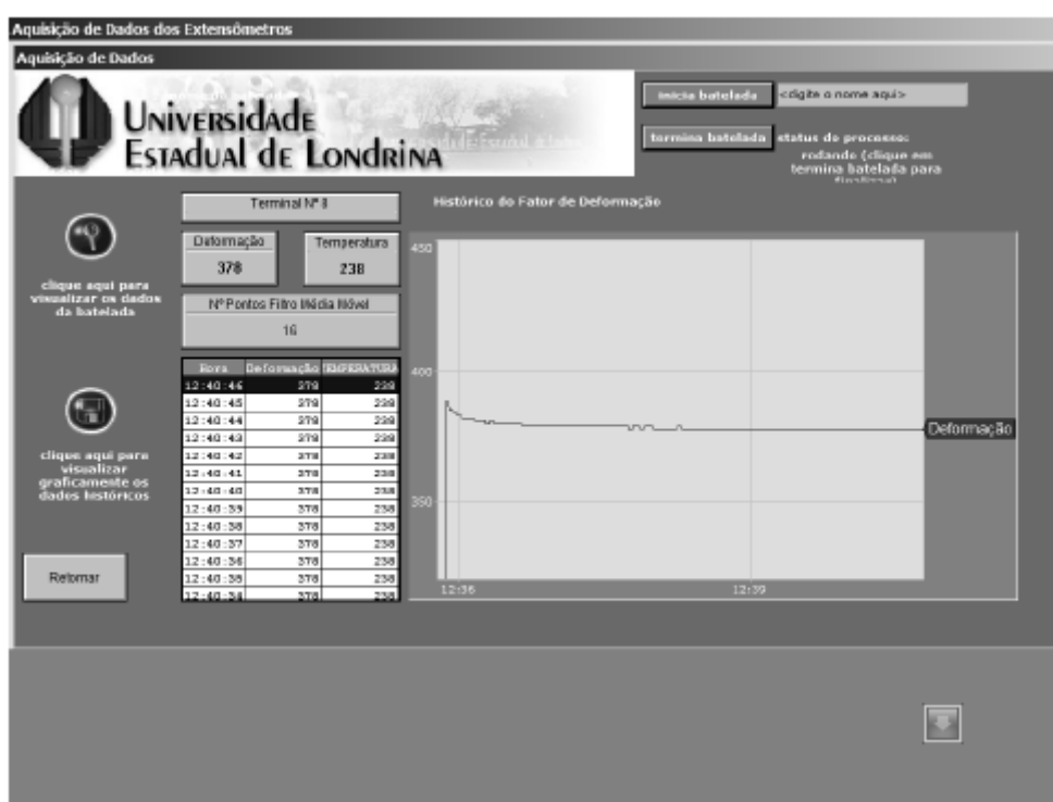
Figura 95 – Tela de coleta de dados logo após o sistema ter sido ligado (regime transiente)
