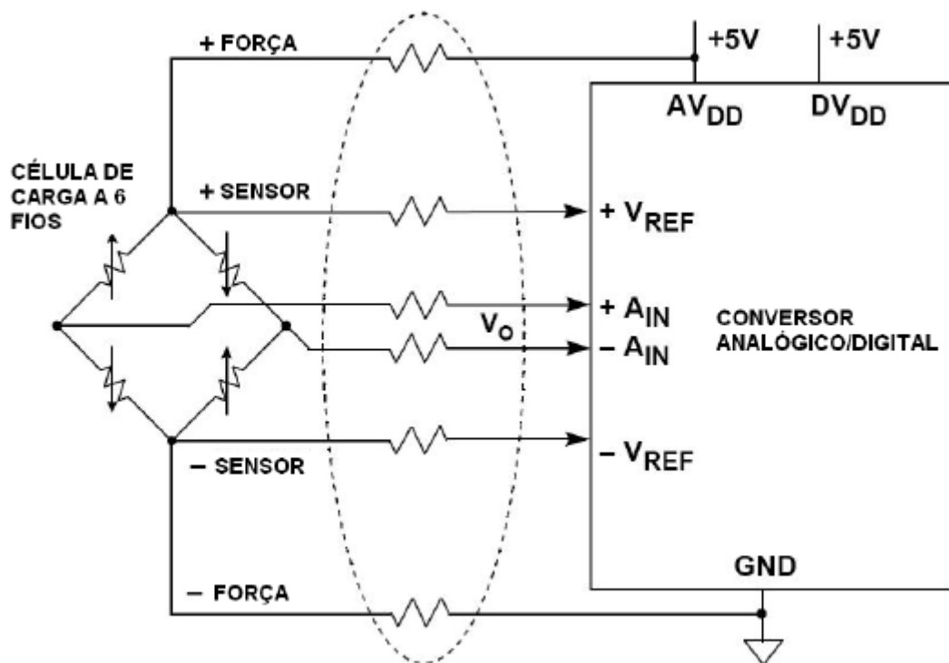
Figura 17 – Efeito da fiação na medição
