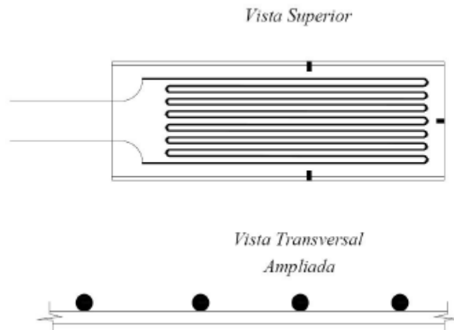
Figura 4 – Extensômetro Elétrico a fio ( wire gauges )
