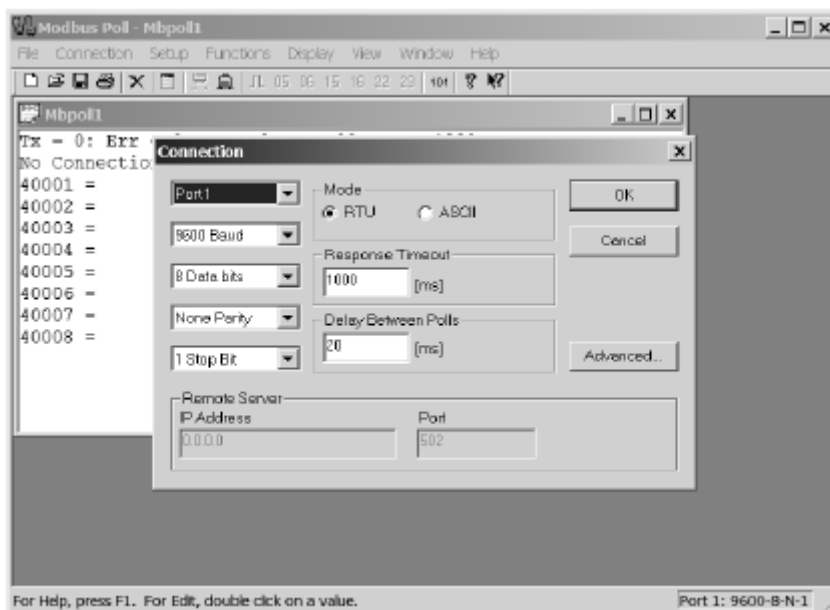
Figura 86 – Configuração da Comunicação no software MBPOLL
