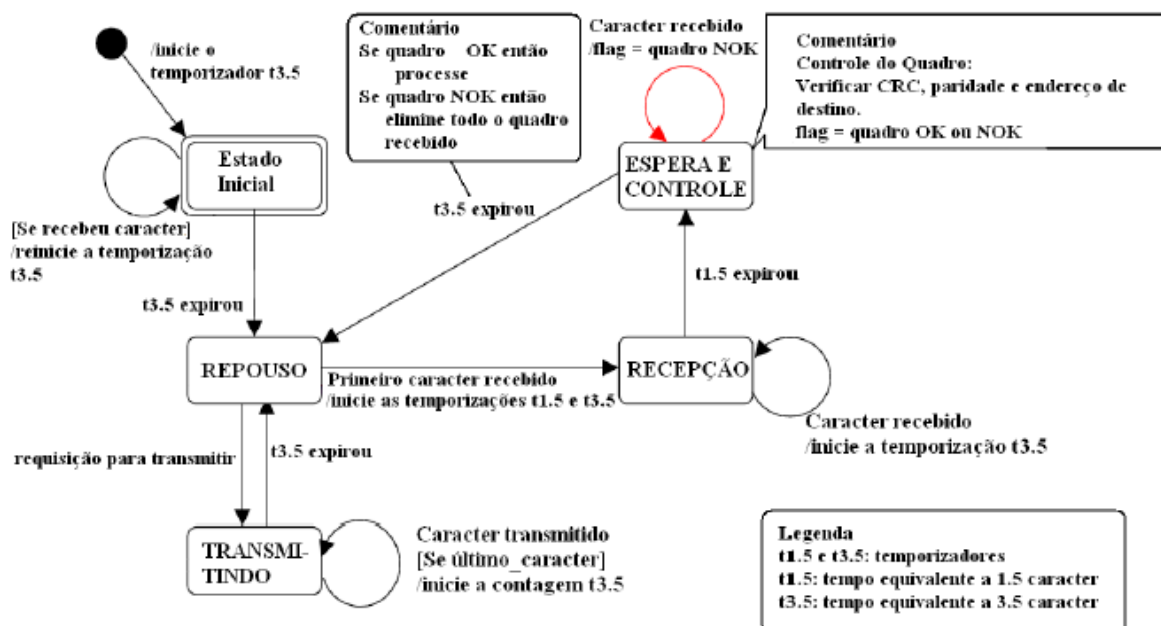
Figura 52 – Máquina de estados MODBUS-RTU TX e RX da estação escrava (MODBUS-IRDA, 2007).
