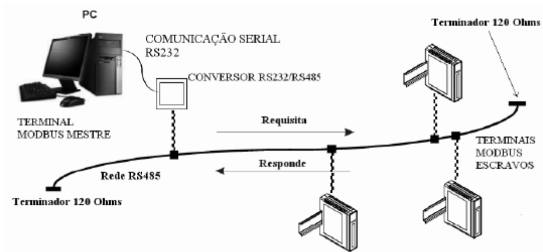
Figura 18 – Arquitetura geral do sistema proposto
