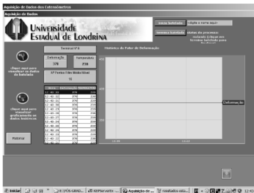
Figura 96 – Tela de coleta de dados mostrando estabilidade com o passar do tempo (regime permanente)
