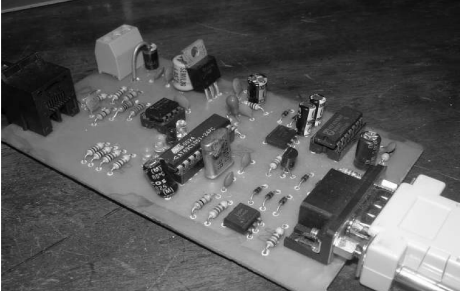
Figura 61 – Fotografia do Conversor RS232/RS485 Implementado
