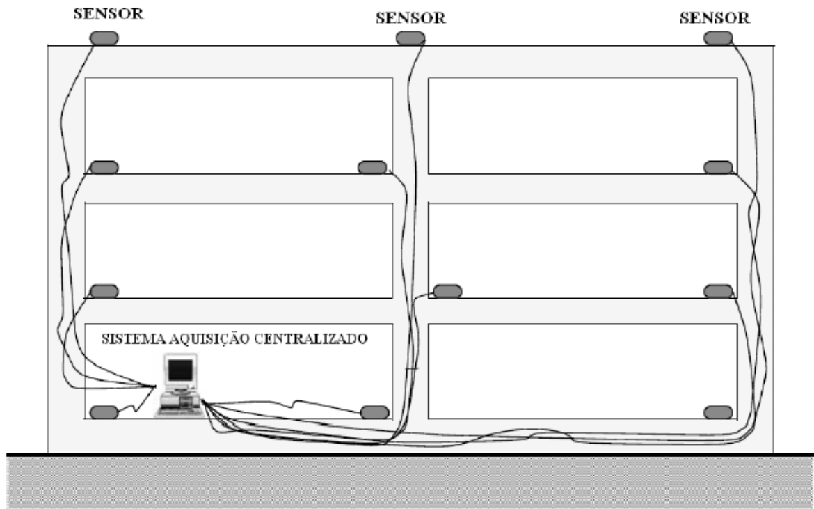
Figura 1 – Sistema convencional de aquisição de dados extensométricos
