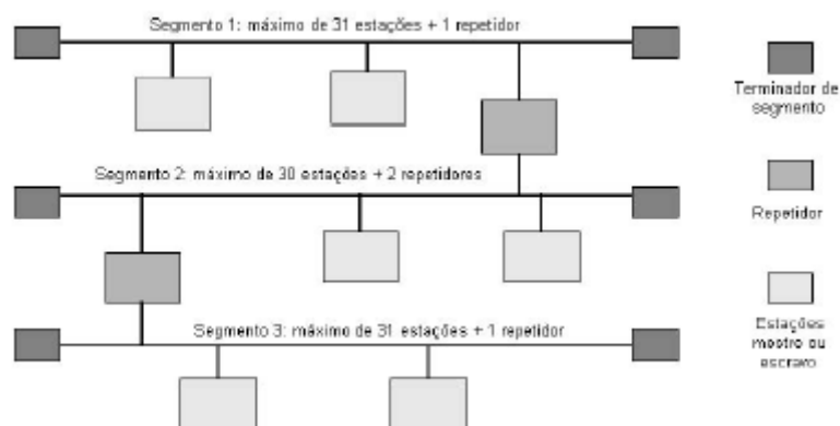
Figura 59 – Utilização de repetidores (TRISTÃO, 2004).
