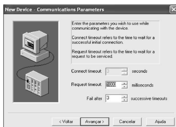
Figura 69 – Criação de um novo nó na rede no software Kepware Server Modbus - etapa 4 parâmetros da comunicação.
