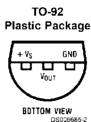
Figura 41 – Encapsulamento do sensor de temperatura LM35 (TO-92)
