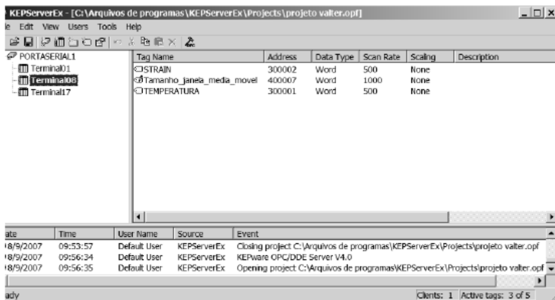
Figura 94 – Configuração do Servidor OPC MODBUS
