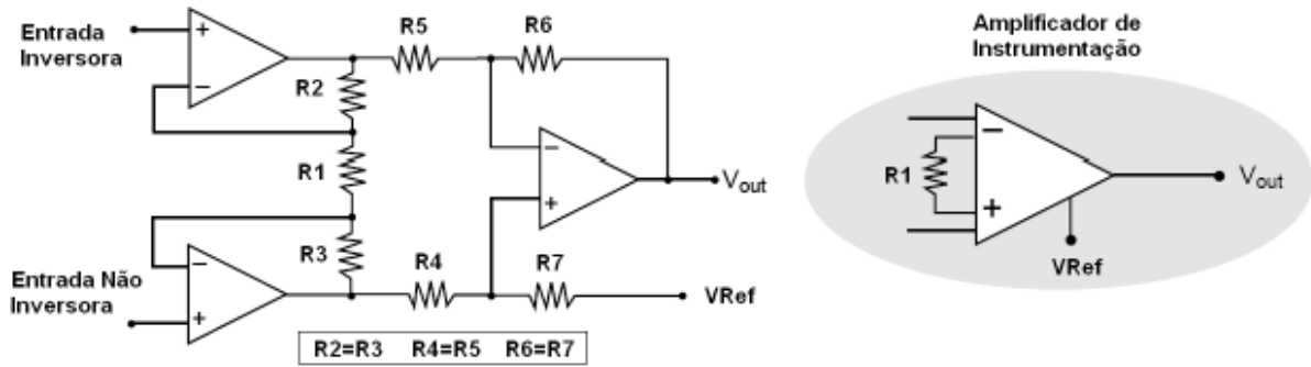
Figura 27 – Amplificador de Instrumentação utilizando 3 amplificadores operacionais
