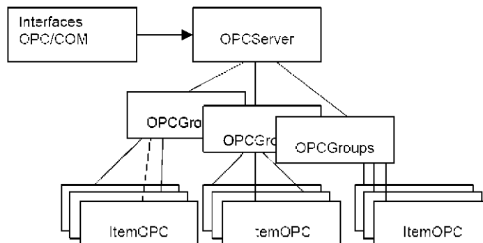
Figura 23 – Estrutura organizacional de um servidor OPC contendo uma hierarquia de grupos e itens
