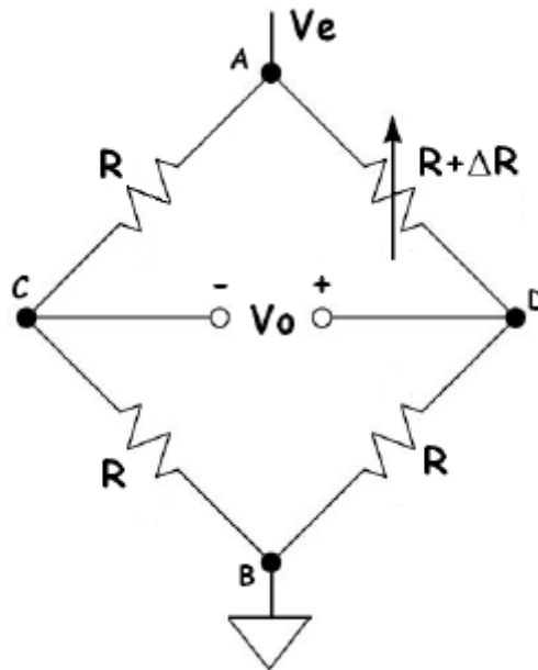
Figura 13 – Extensômetro ligado em um quarto de ponte
